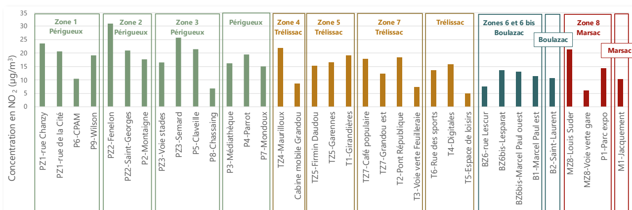
Figure 25 | Concentrations moyennes de NO 2 mesurées par tubes passifs, triés par zone
