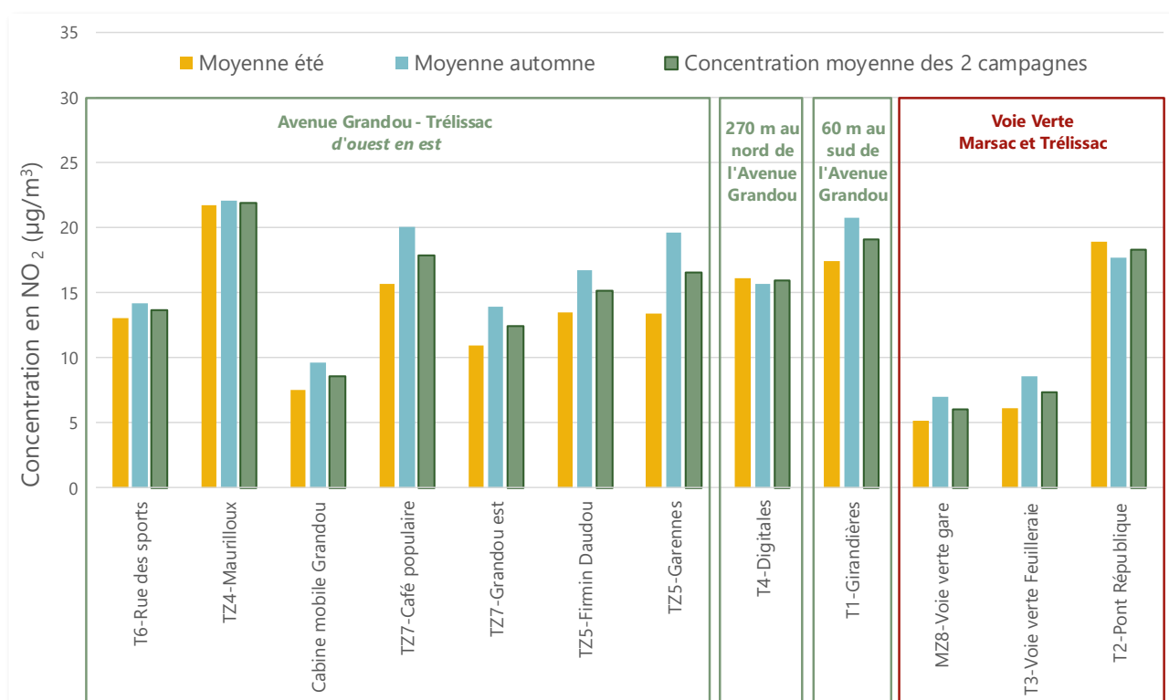
Figure 28 | Concentrations moyennes de \text{NO}_2 mesurées par tubes passifs, zoom voies vertes et avenue Michel Grandou
