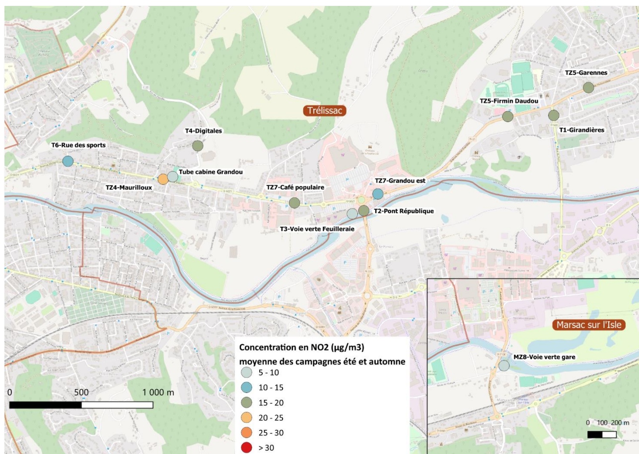
Figure 29 | Cartographie des concentrations moyennes de NO 2 , zoom voies vertes et avenue Michel Grandou
