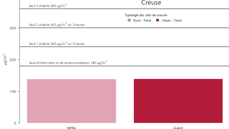
O 3 – maximum horaire en 2019 Creuse
