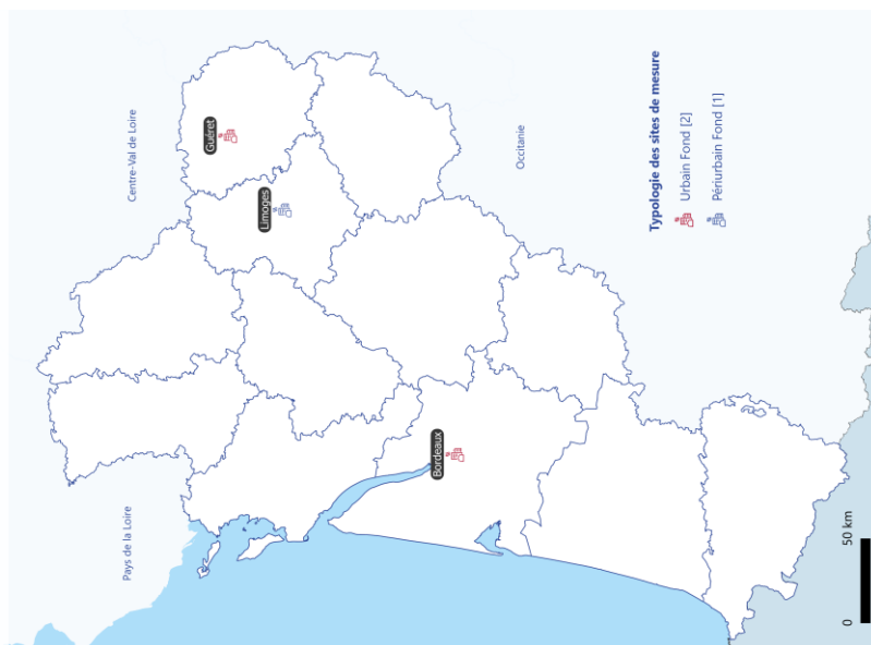
Sites fixes de mesure des métaux lourds - 2019
