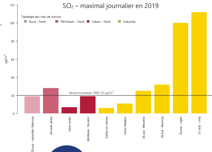
SO 2 – maximal journalier en 2019
