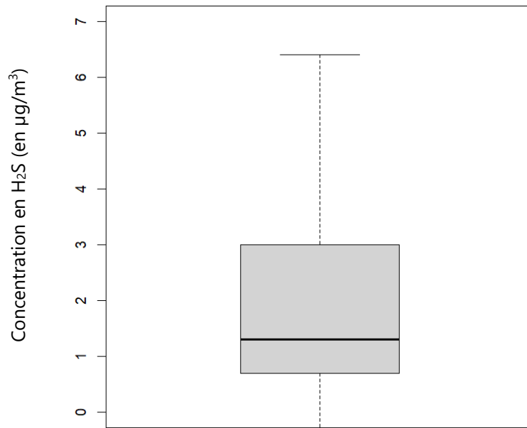
Figure 22 : boxplot des concentrations en sulfure d'hydrogène mesurées sur le parking de l'usine (moyennes horaires)
