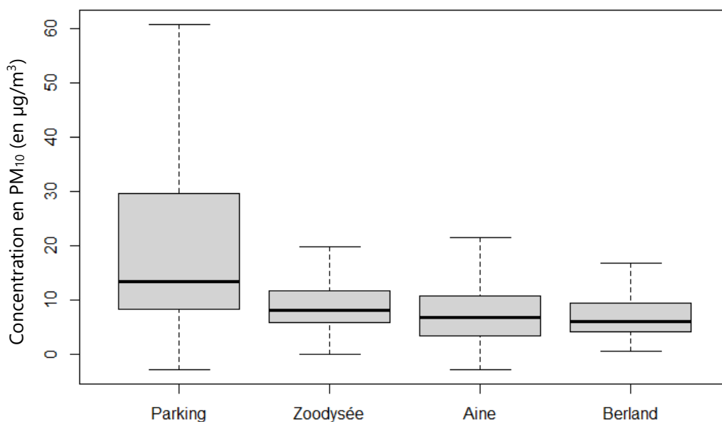
Figure 27 : boxplot des concentrations en PM 10 mesurées (en moyennes horaires)
