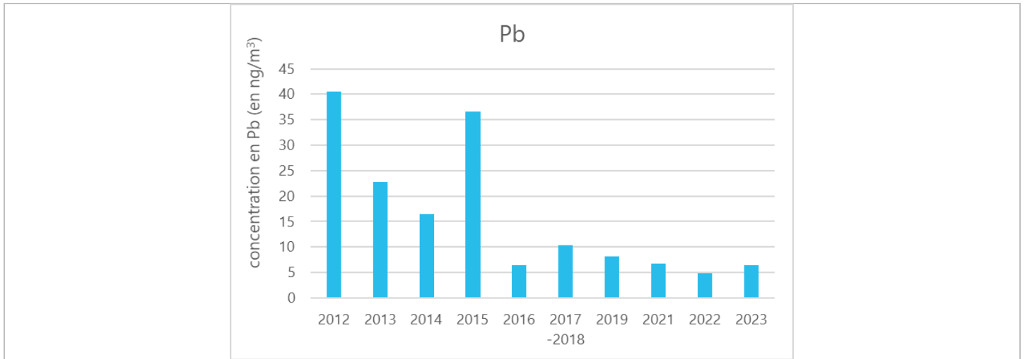
Figure 11 : évolution des concentrations en métaux dans l'air ambiant depuis 2012
