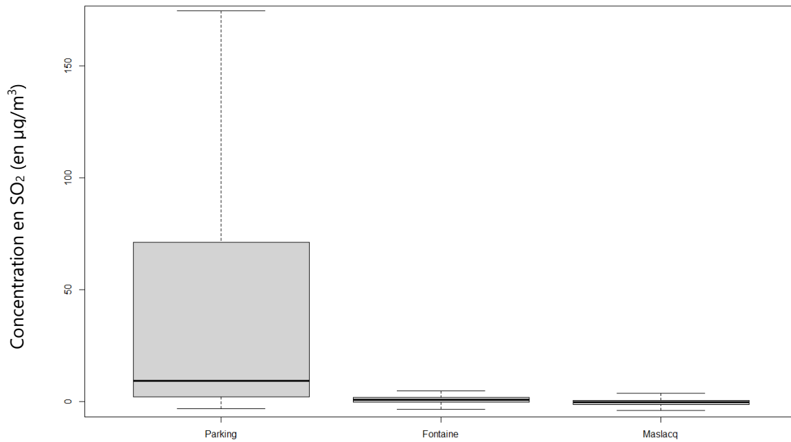
Figure 18 : boxplot des concentrations en dioxyde de soufre mesurées (moyennes horaires)
