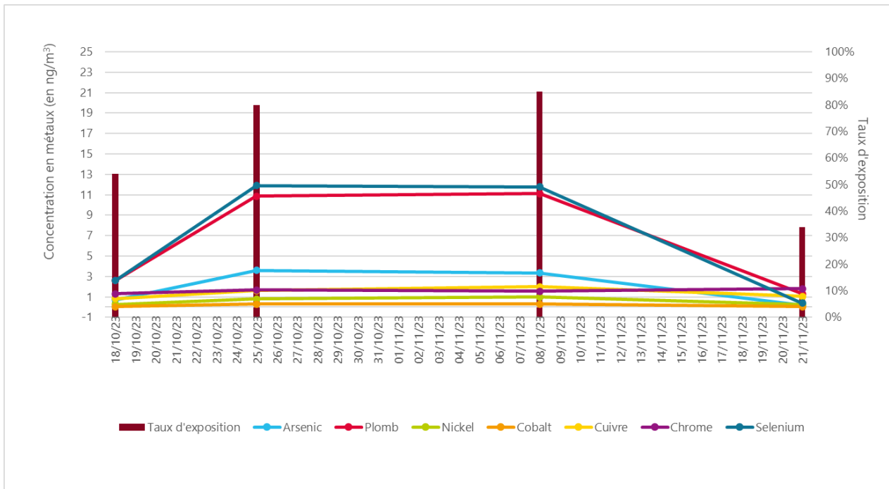
Figure 10 : résultats des prélèvements de métaux en air ambiant
