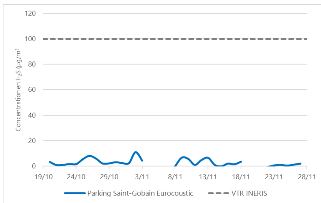
Figure 25 : évolution des concentrations en sulfure d'hydrogène sur la période de mesure (en moyennes journalières)
