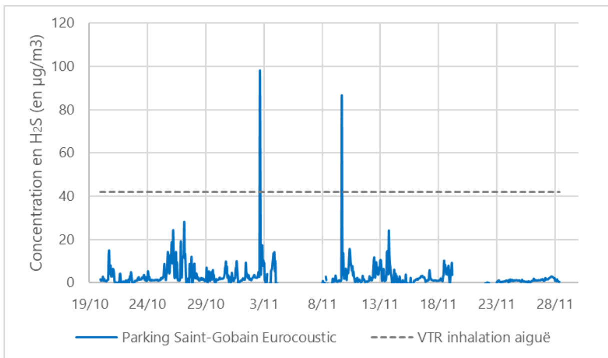
Figure 24 : évolution des concentrations en sulfure d'hydrogène sur la période de mesure (en moyennes horaires)
