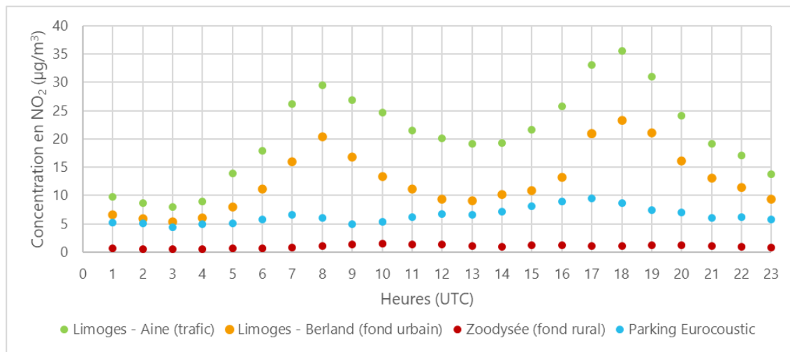
Figure 16 : profils moyens journaliers du dioxyde d'azote pendant la période de mesure
