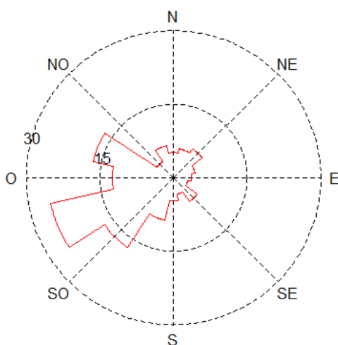
Figure 17 : rose de concentration en NO 2 pendant la période de mesure (en µg/m 3 ) (moyennes horaires)
