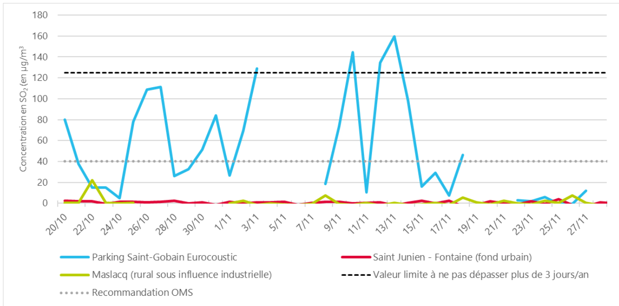
Figure 20 : évolution des concentrations en dioxyde de soufre sur la période de mesure (en moyennes journalières)
