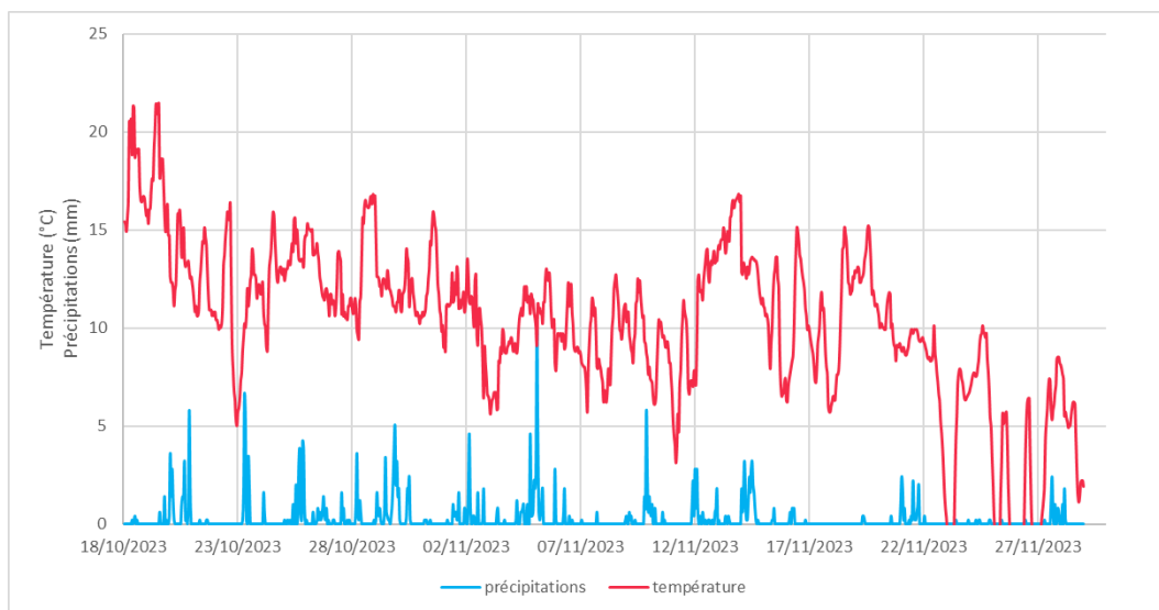
Figure 9 : températures moyennes et pluviométrie entre le 18/10 et le 29/11/2023
