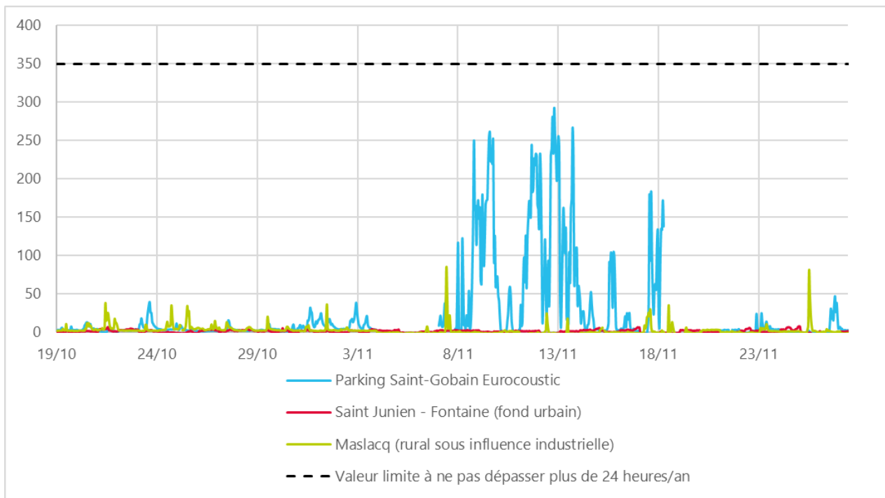
Figure 19 : évolution des concentrations en dioxyde de soufre sur la période de mesure (en moyennes horaires)
