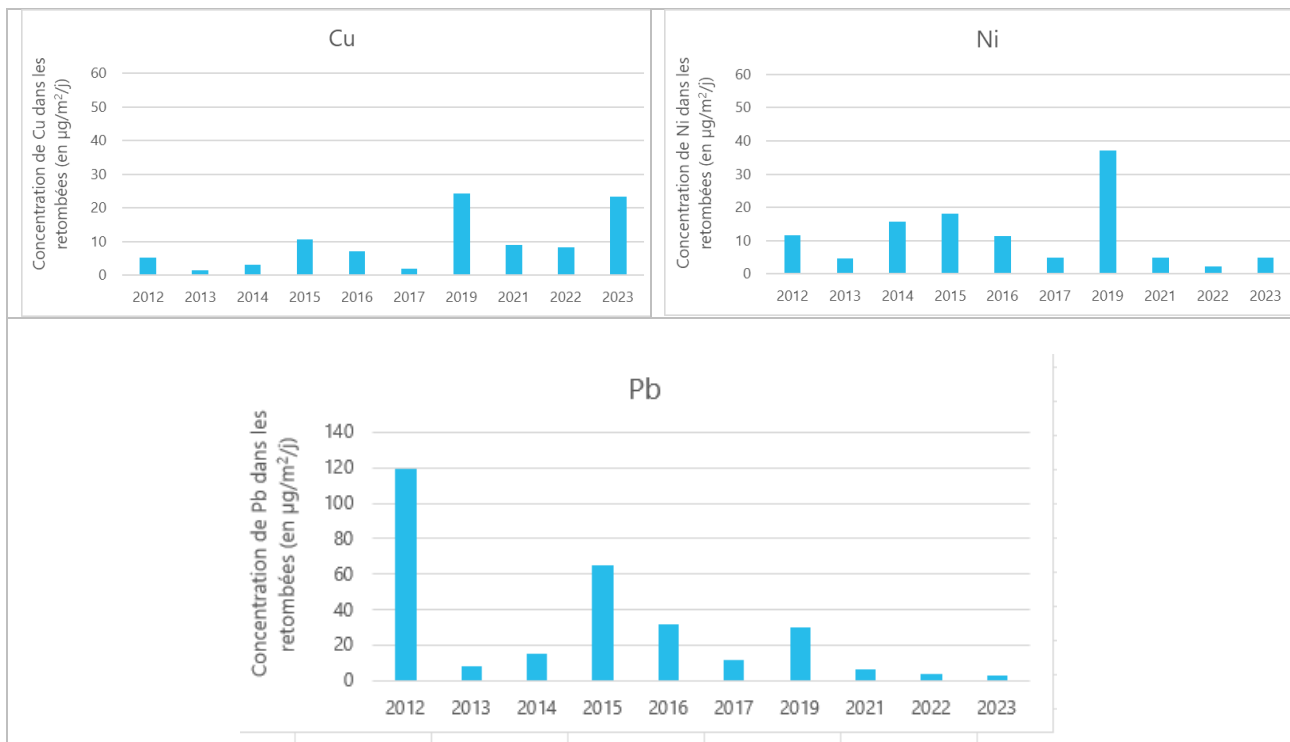
Figure 12 : évolution des concentrations en métaux dans les retombées depuis 2012
