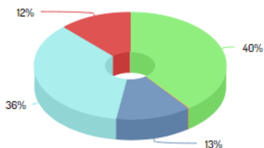
Figure 3 : émissions de PM 10 en Nouvelle Aquitaine- Inventaire des émissions 2018
