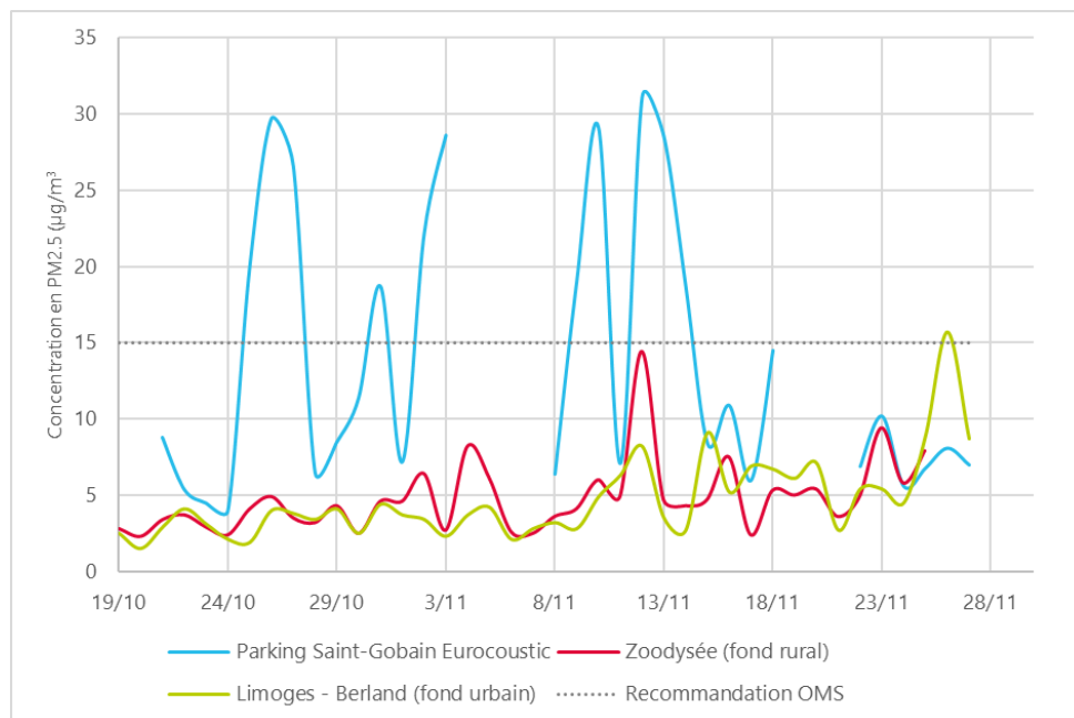
Figure 31 : évolution des concentrations en PM 2.5 sur la période de mesure (en moyennes journalières)
