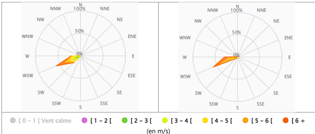
Figure 33 : roses des vents moyenne sur la station Météo France de Genouillac
