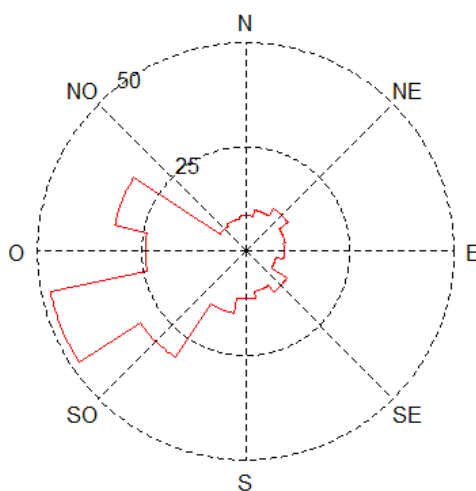
Figure 29 : rose de concentration en \text{PM}_{10} pendant la période de mesure (en \mu\text{g}/\text{m}^3 ) (en moyennes horaires)
