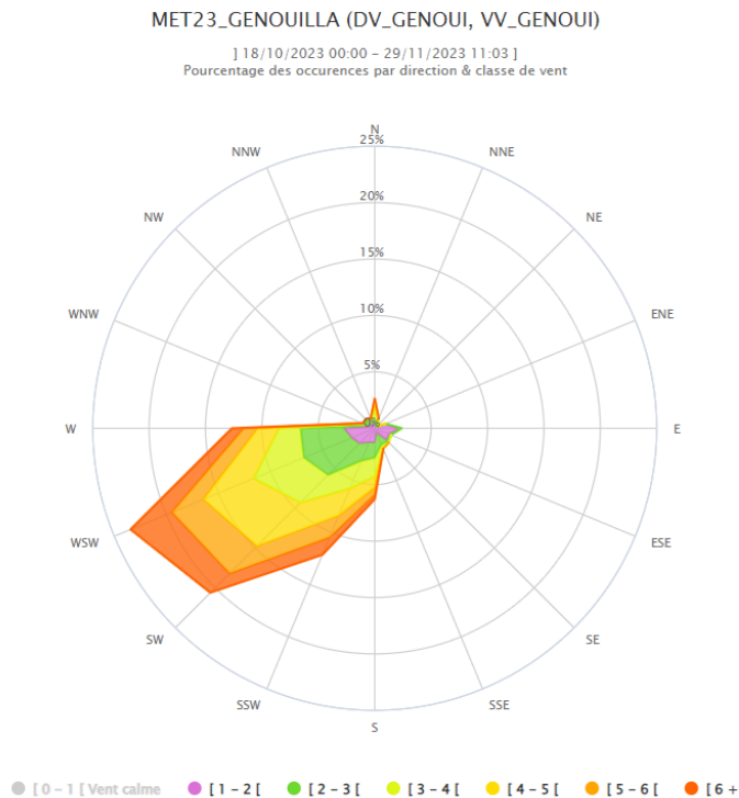
Figure 8 : rose des vents moyenne sur la station Météo France de Genouillac du 18/10 au 29/11/2023
