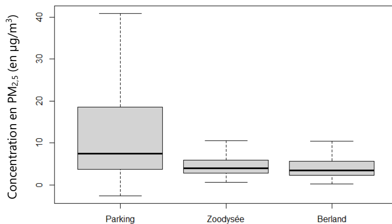
Figure 30 : boxplot des concentrations en PM 2.5 mesurées (en moyennes horaires)
