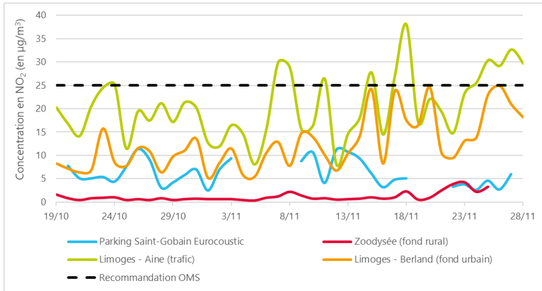
Figure 15 : évolution des concentrations en dioxyde d'azote sur la période de mesure (en moyennes journalières)
