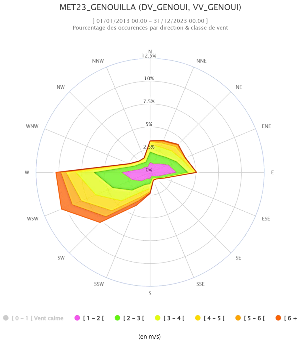
Figure 6 : rose des vents moyenne sur la station Météo France de Genouillac sur une période de 10 ans, du 01/01/2013 au 31/12/2023
