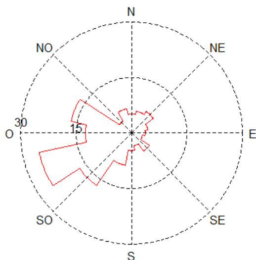
Figure 32 : rose de concentration en PM_{2,5} pendant la période de mesure (en \mu g/m^3 ) (en moyennes horaires)
