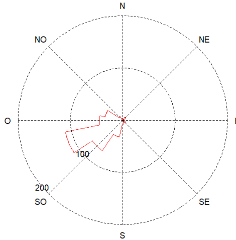
Figure 21 : rose de concentration en SO 2 pendant la période de mesure (en µg/m 3 ) (moyennes horaires)
