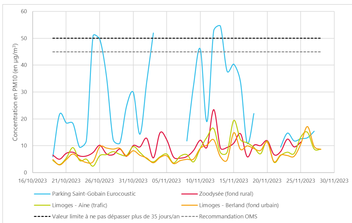
Figure 28 : évolution des concentrations en PM 10 sur la période de mesure (en moyennes journalières)
