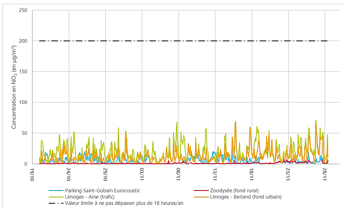
Figure 14 : évolution des concentrations en dioxyde d'azote sur la période de mesure (en moyennes horaires)
