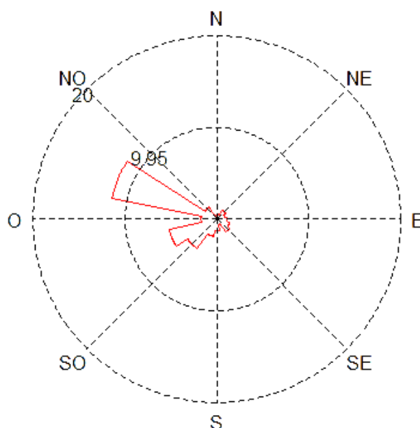
Figure 26 : rose de concentration en H 2 S pendant la période de mesure (en µg/m 3 ) (moyennes horaires)
