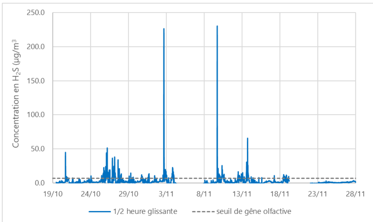
Figure 23 : évolution des concentrations en sulfure d'hydrogène sur la période de mesure (en moyennes demi-heure glissantes)
