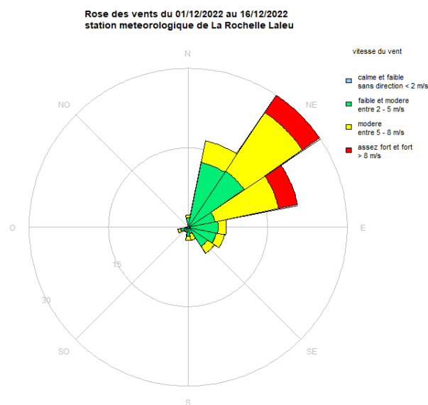
Figure 10 : Rose des vents campagne mesure site STEP
