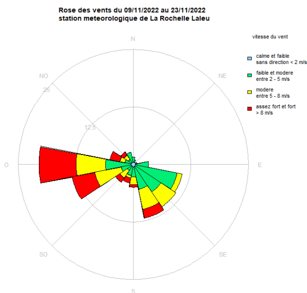
Figure 4 : Rose des vents première campagne de mesure Port-Neuf
