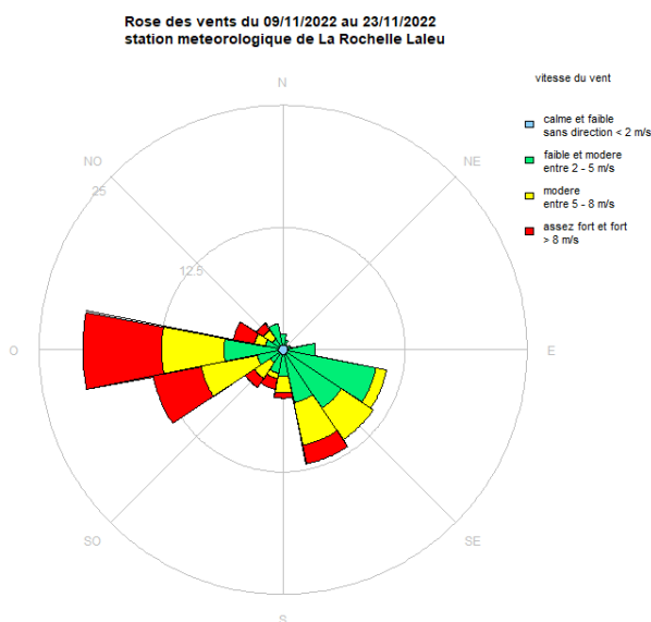
Figure 9 : Rose des vents campagne de mesure site Bassin STEP et Port-Neuf
