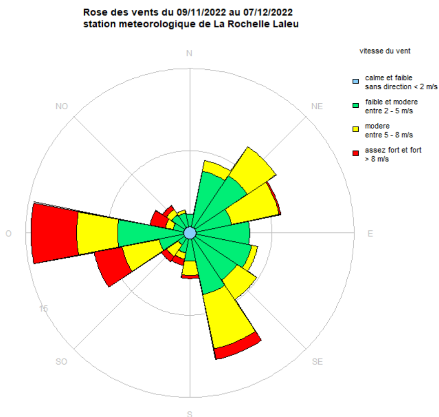
Figure 2 : Rose des vents campagne de mesure
