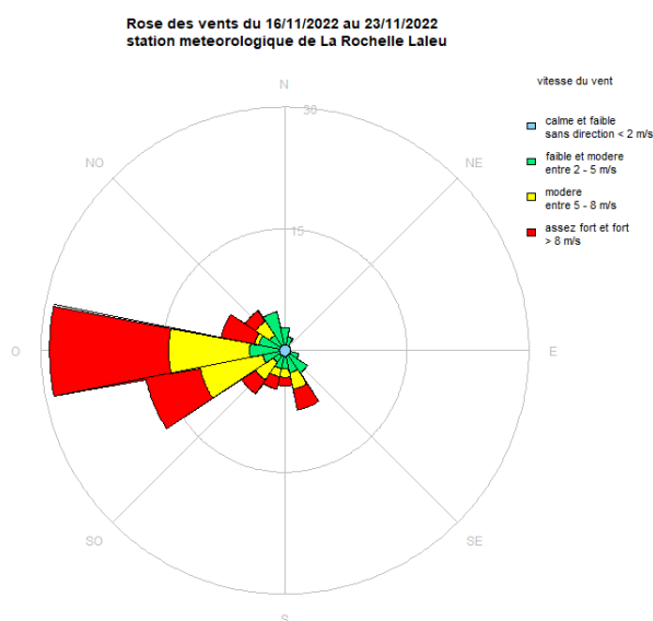
Figure 8 : Rose des vents deuxième campagne mesure
