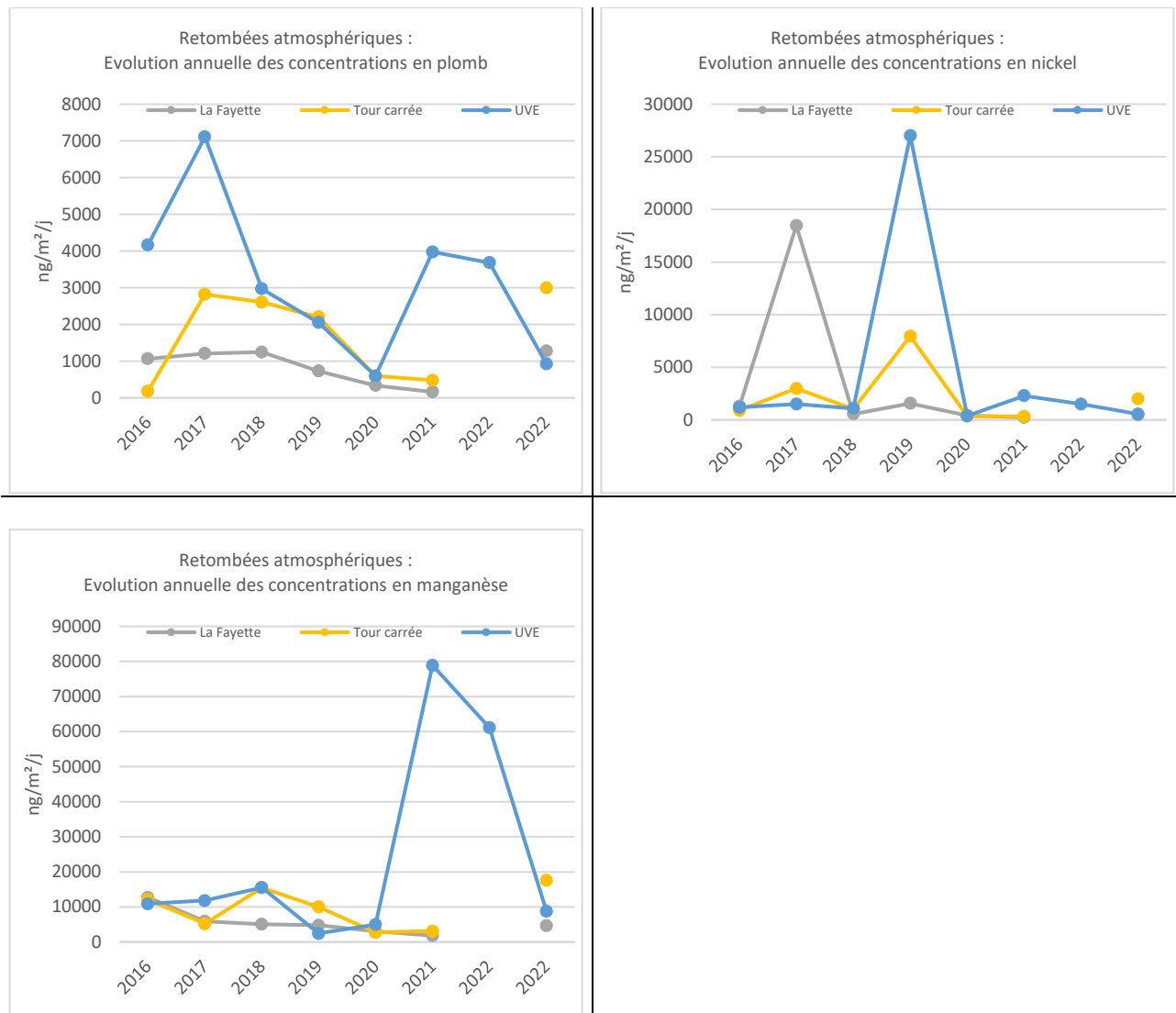
Figure 23 : 2016 – 2022 : évolution de la concentration en métaux lourds au niveau des trois sites de mesure
