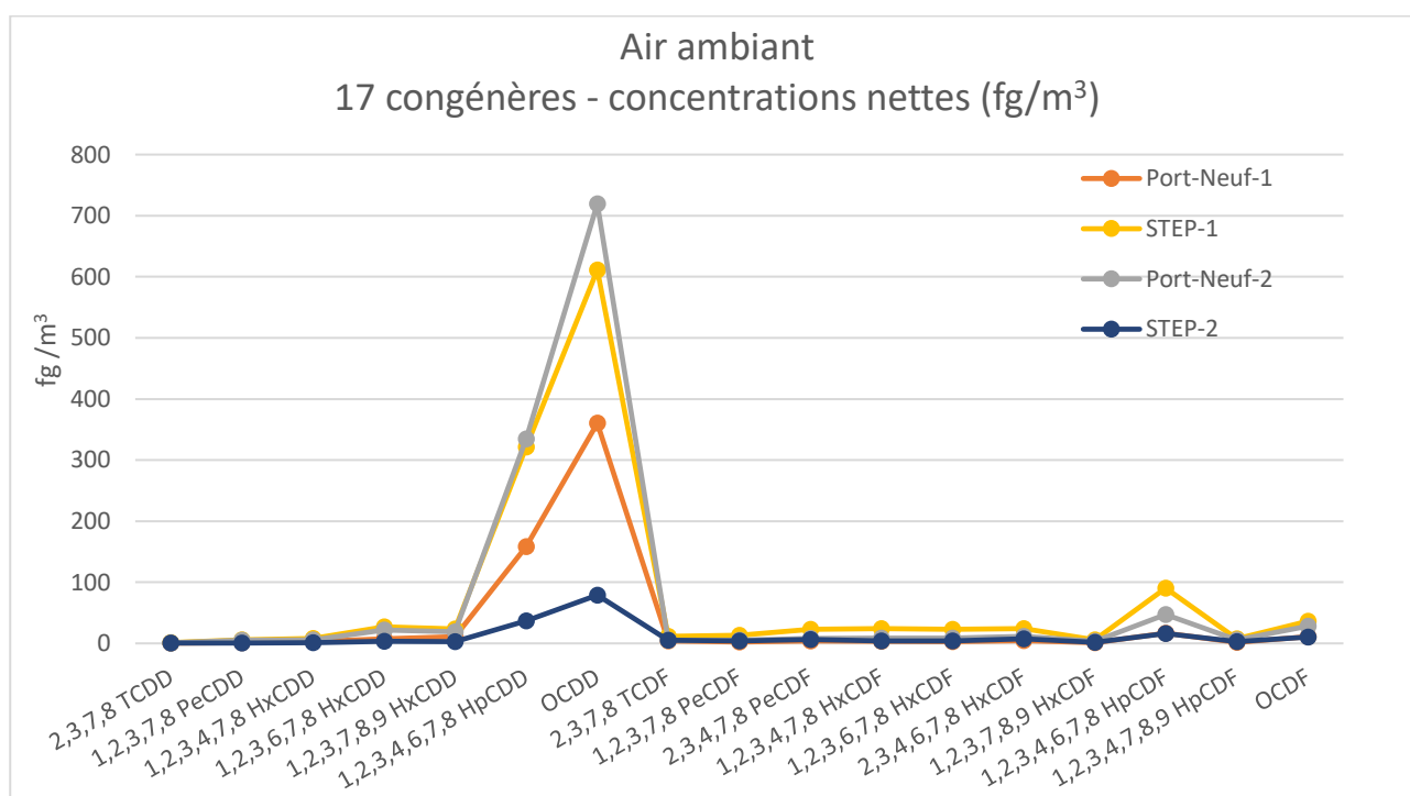
Figure 11 : Concentrations nettes des 17 congénères en air ambiant
