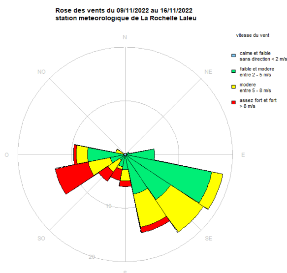
Figure 7 : Rose des vents première campagne mesure
