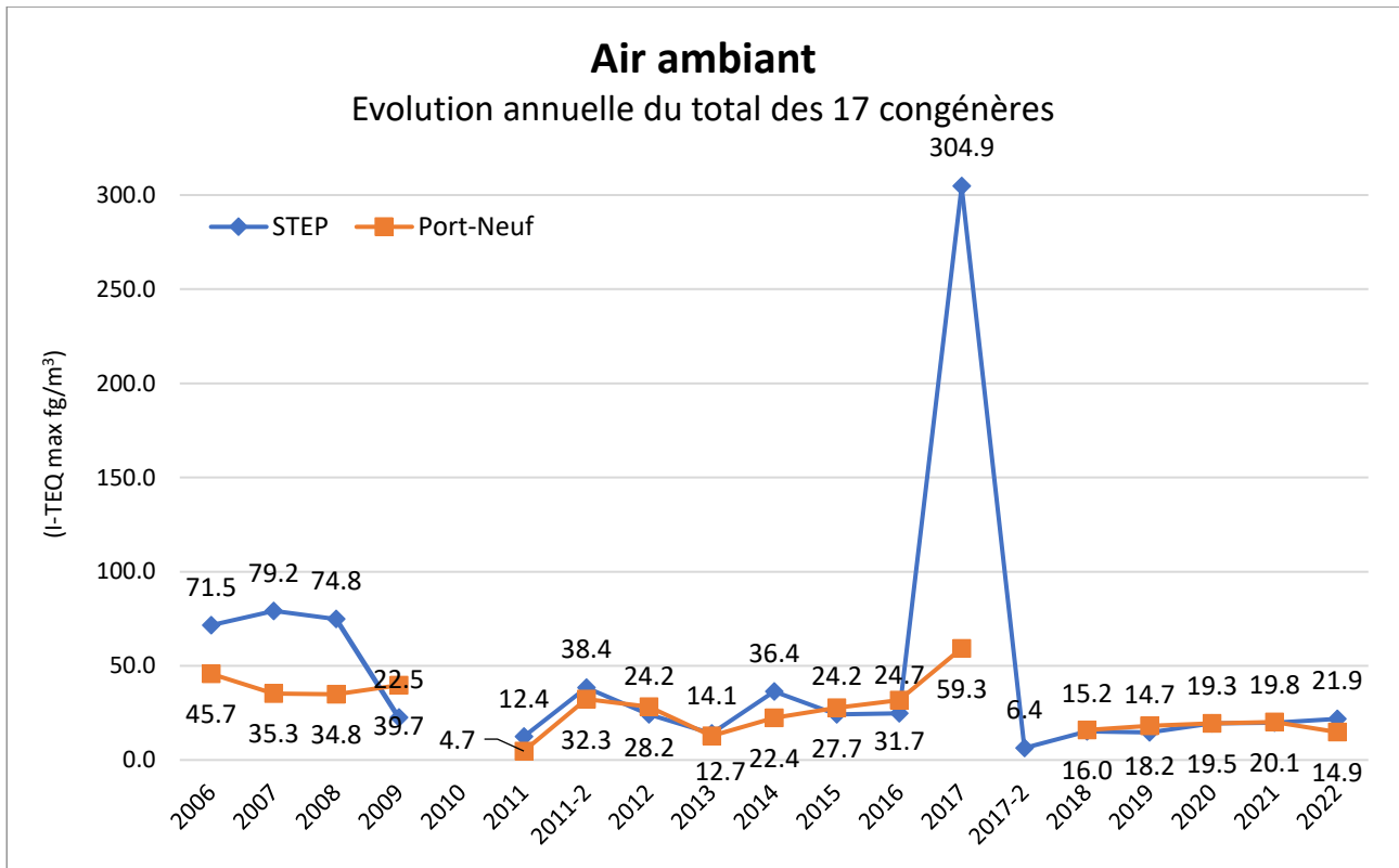
Figure 13 : Évolution annuelle des concentrations en équivalence toxique du total des 17 congénères
