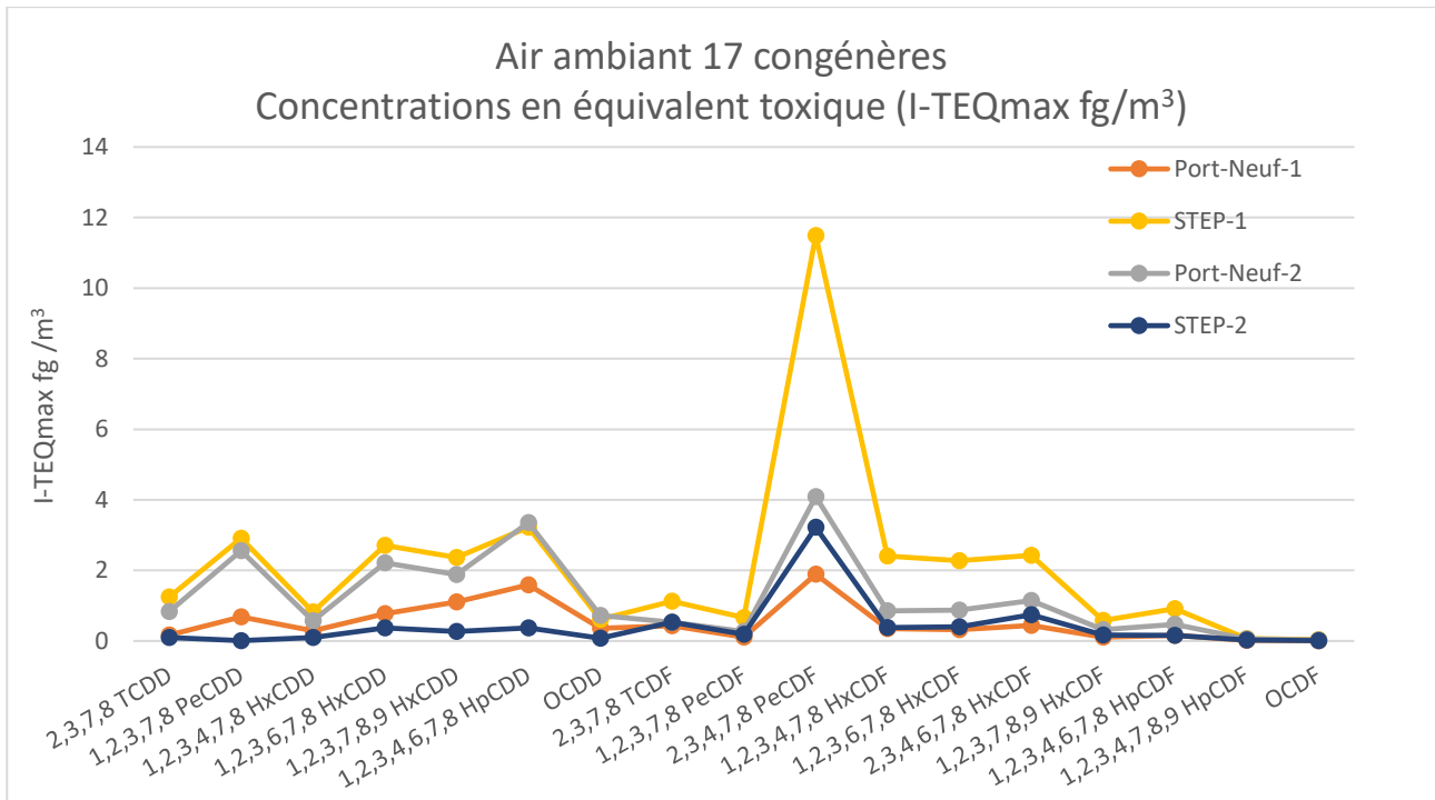
Figure 12 : Concentrations en équivalent toxique des 17 congénères en air ambiant
