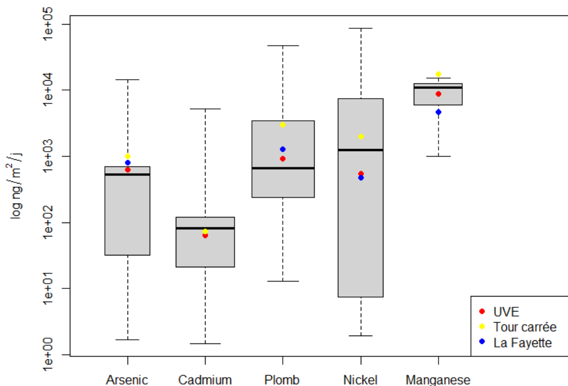
Figure 24 : Comparaison des concentrations en métaux lourds avec des campagnes de mesure réalisées en Nouvelle-Aquitaine entre 2007 et 2018
