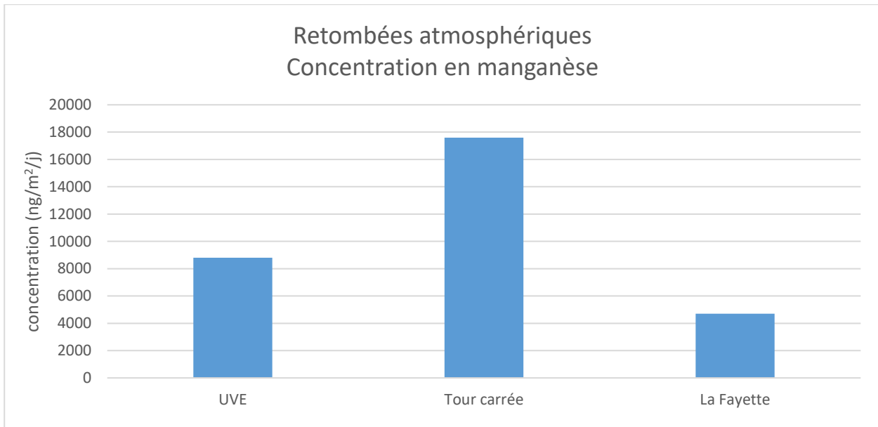
Figure 22 : Concentrations en manganèse dans les retombées atmosphériques
