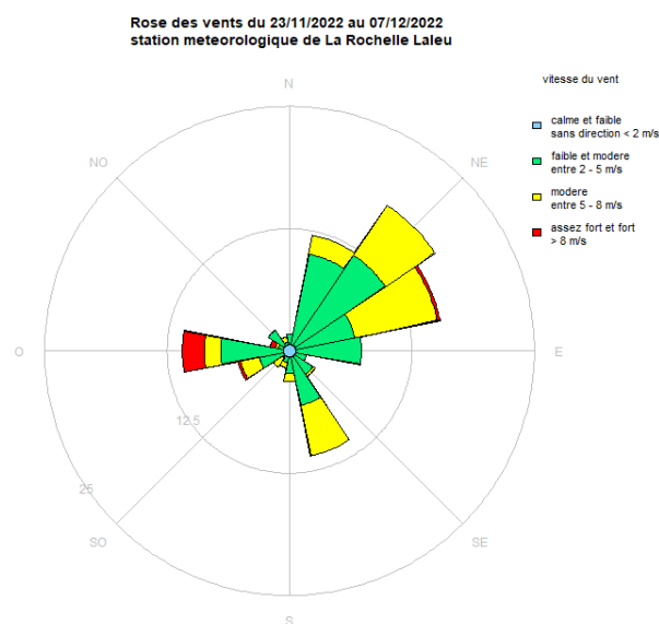
Figure 5 : Rose des vents deuxième campagne mesure Port-Neuf, première campagne de mesure STEP
