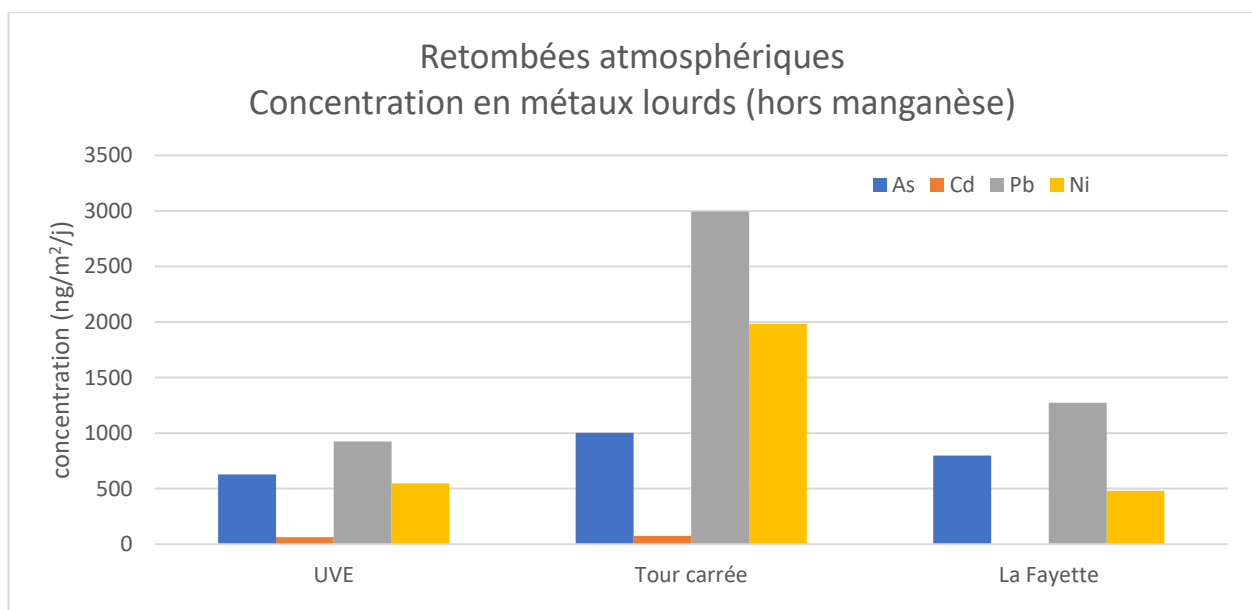
Figure 21 : Concentrations en métaux lourds dans les retombées atmosphériques
