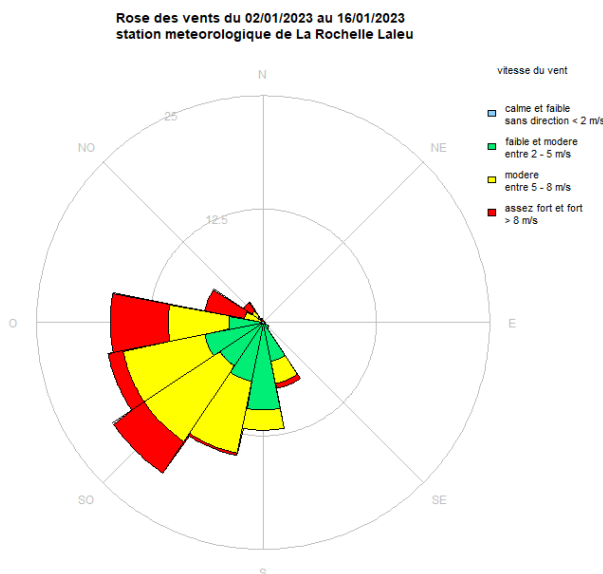
Figure 6 : Rose des vents deuxième campagne de mesure STEP
