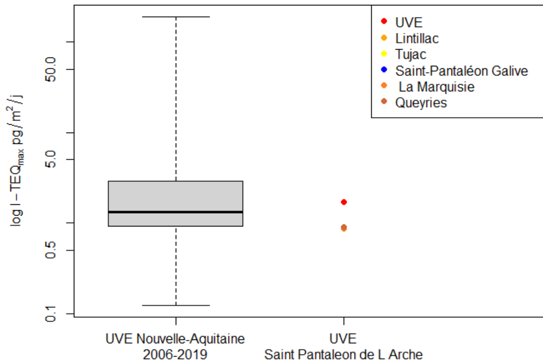
Figure 13 : Comparaison avec les concentrations mesurées en équivalent toxique dans les retombées atmosphériques sur la région Nouvelle-Aquitaine
