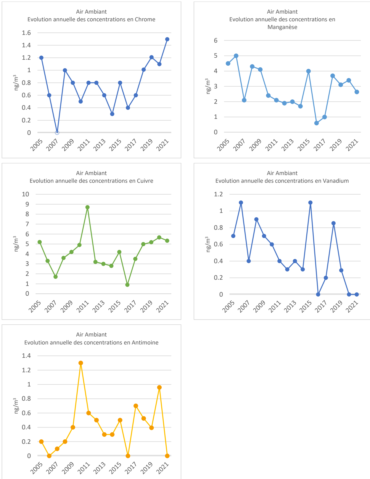
Figure 20 : Évolution des concentrations métaux lourds non réglementés en air ambiant
