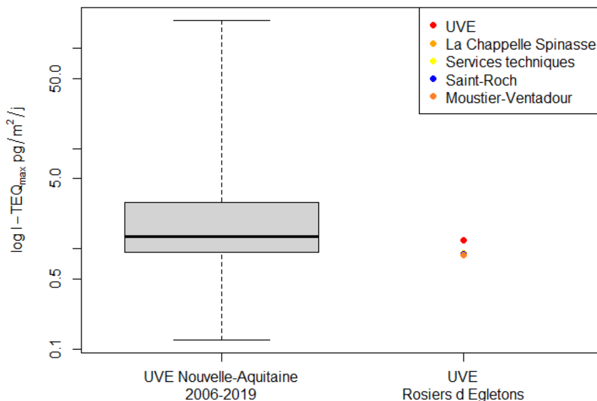
Figure 35 : Comparaison avec les concentrations mesurées en équivalent toxique dans les retombées atmosphériques sur la région Nouvelle-Aquitaine
