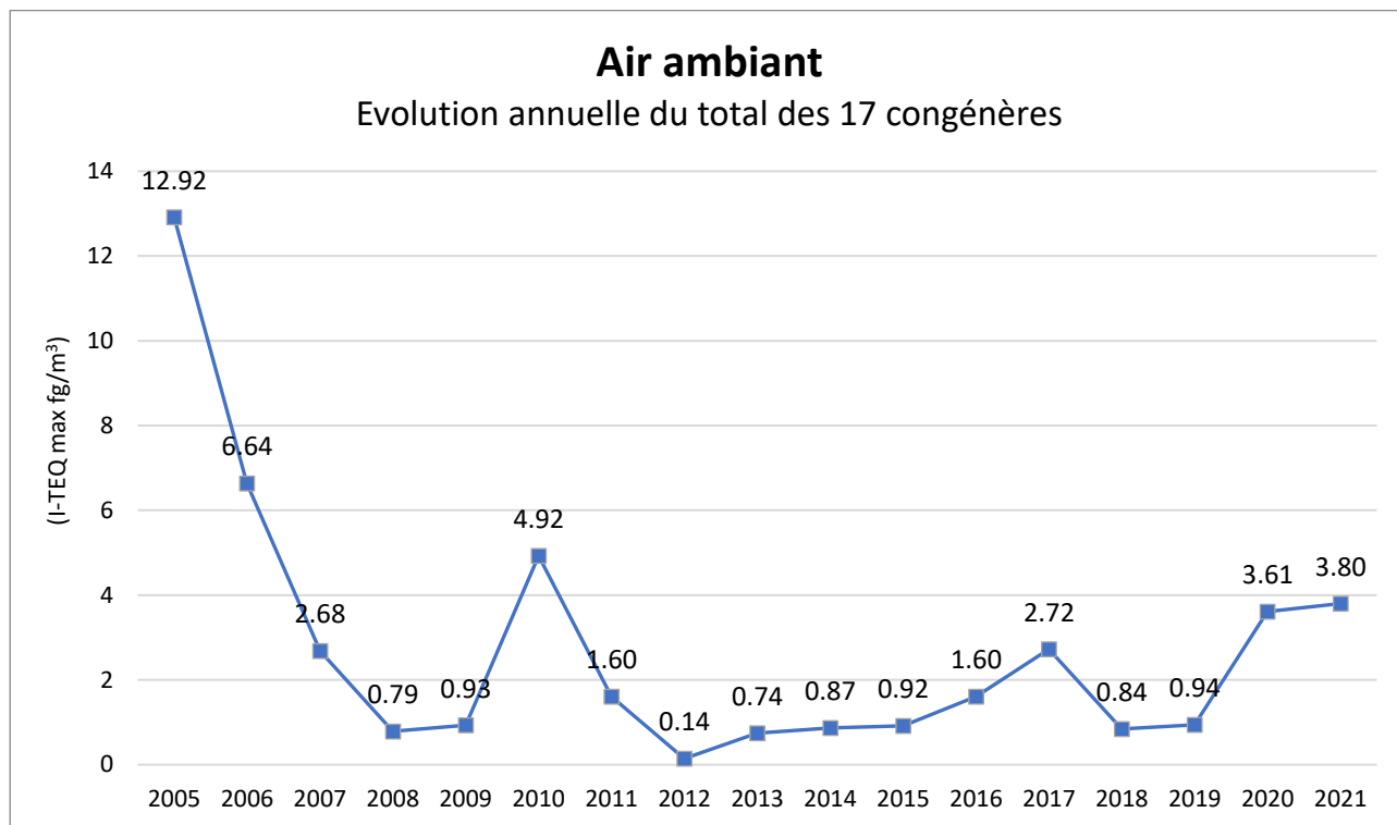
Figure 31 : Évolution annuelle des concentrations en équivalence toxique du total des 17 congénères
