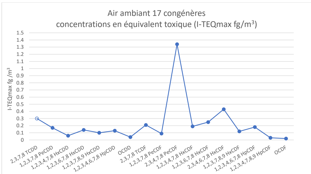
Figure 30 : Concentration en équivalence toxique des 17 congénères en air ambiant
