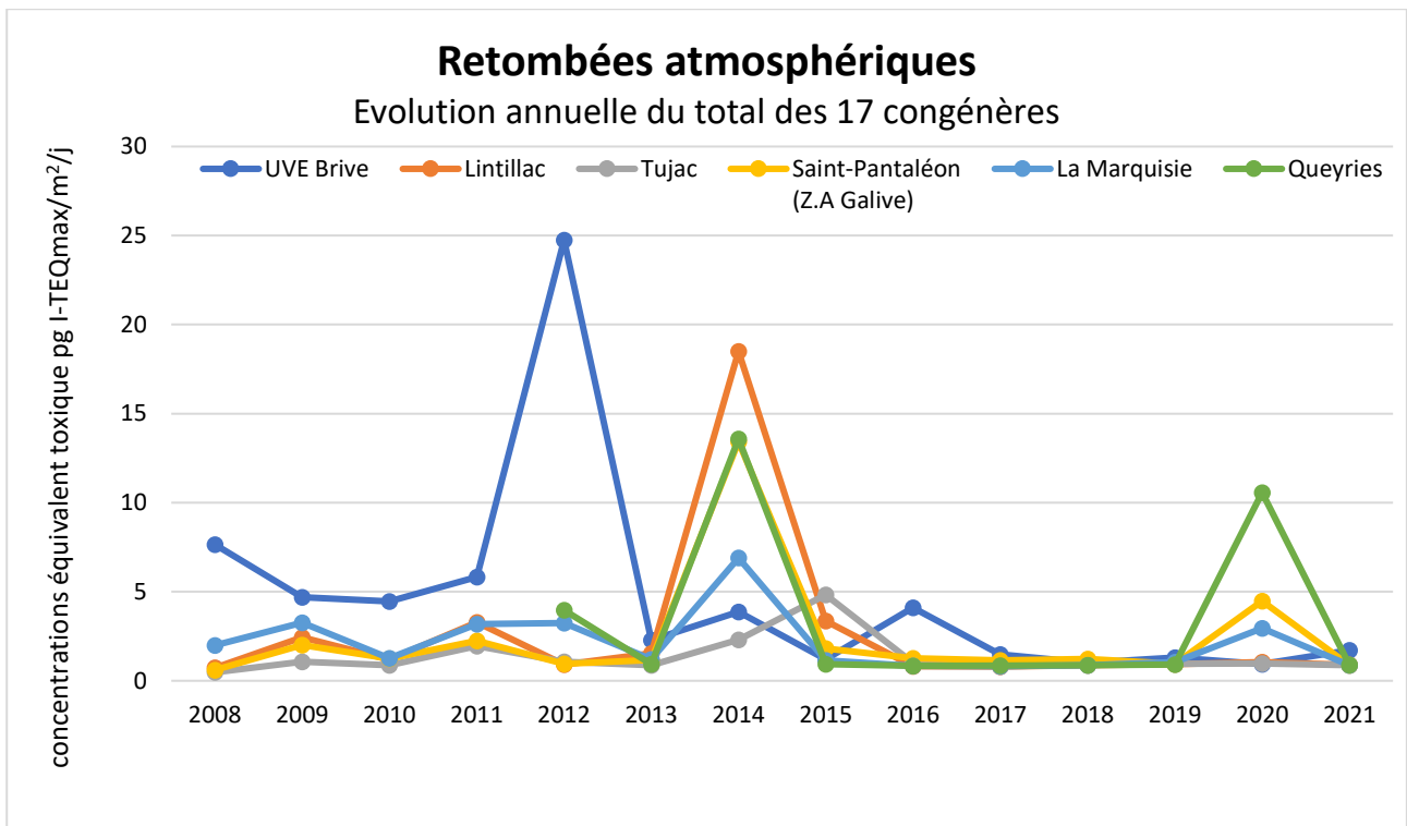
Figure 12 : Évolution annuelle de l'indice ITEQ dans les retombées atmosphériques
