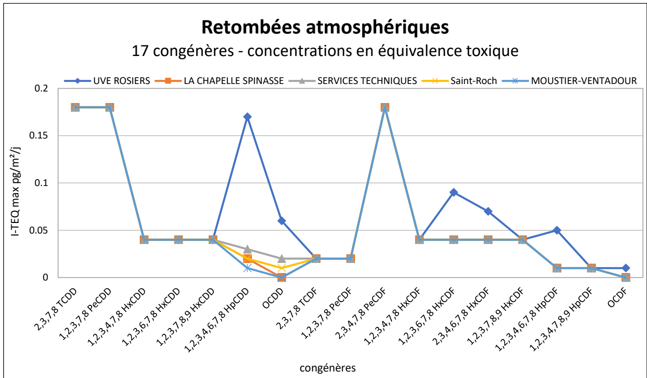
Figure 33 : Résultats d'analyses en équivalents toxiques des 17 congénères dans les retombées atmosphériques
