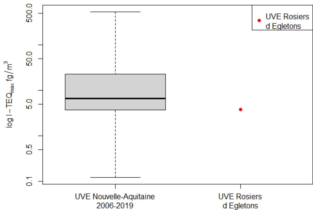
Figure 32 : Comparaison avec les concentrations mesurées en équivalent toxique en air ambiant sur la région Nouvelle-Aquitaine
