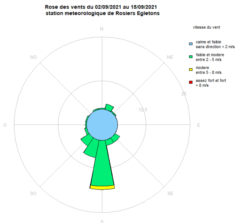
Figure 28 : Rose des vents du 02/09/2021 au 15/09/2021 station Rosiers d'Egletons
