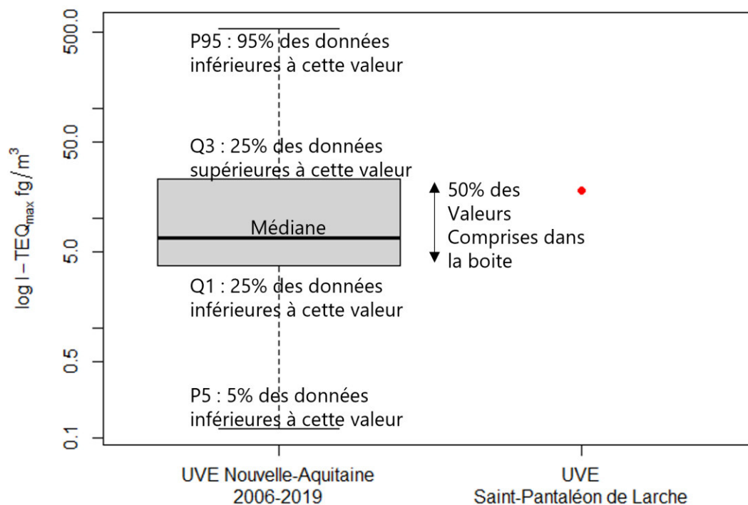
Figure 10 : Comparaison avec les concentrations mesurées en équivalent toxique en air ambiant sur la région Nouvelle-Aquitaine
