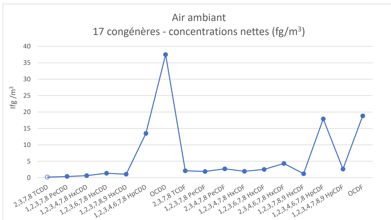
Figure 29 : Concentration nette des 17 congénères en air ambiant
