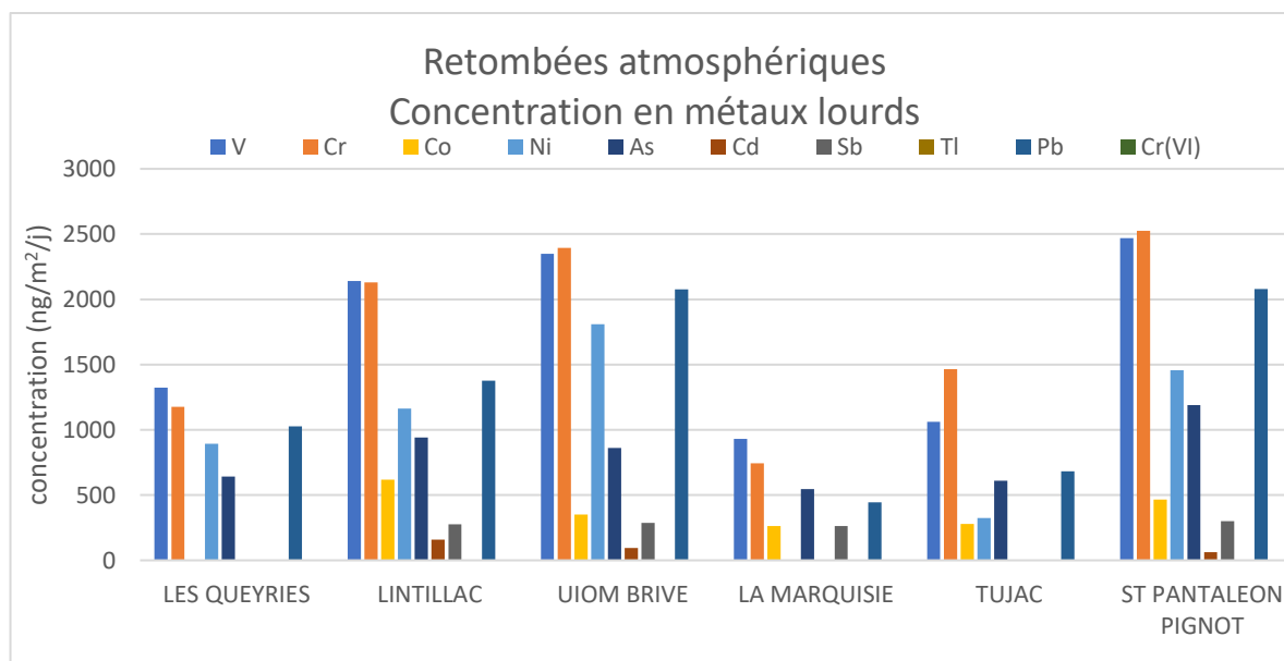
Figure 21 : Concentrations métaux lourds (hors manganèse et cuivre) dans les retombées atmosphériques
