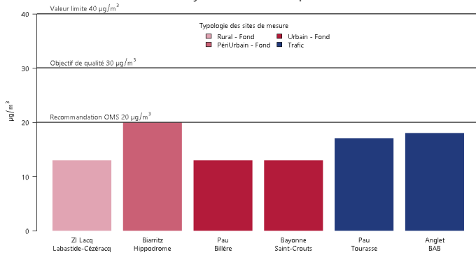
PM10 – moyenne annuelle 2020 Pyrénées-Atlantiques
