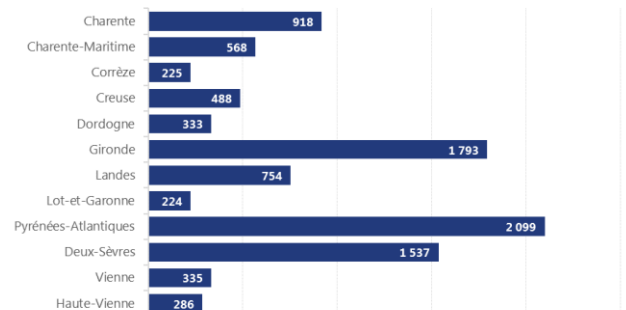
Emissions SO 2 par département - tonne - 2016
