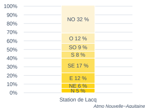
Origine des vents – Août 2022
