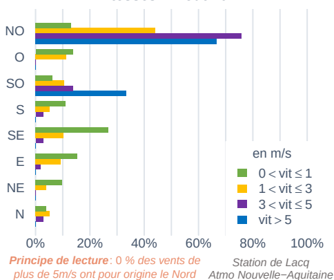
Origine des vents par classes de vitesses – Août 2022
