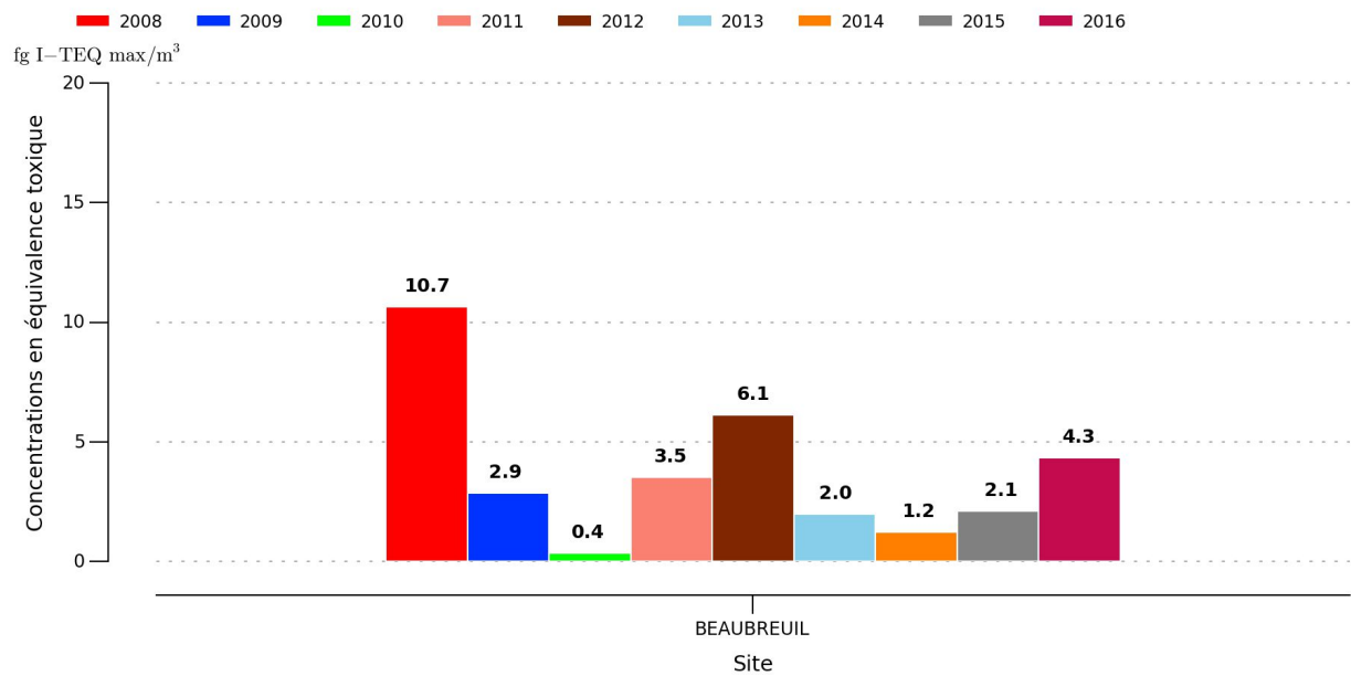
Illustration 14: Evolution annuelle du total des 17 congénères en équivalence toxique
