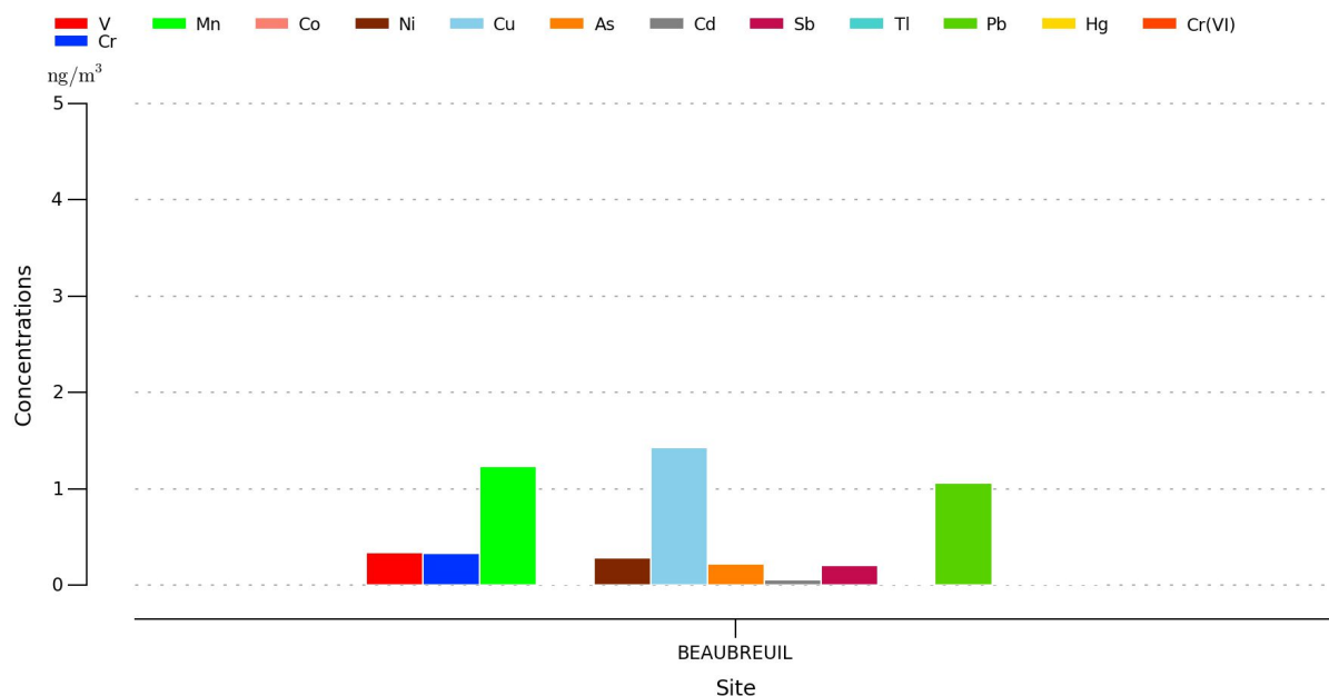
Illustration 17: Diagramme des concentrations en métaux lourds en air ambiant
