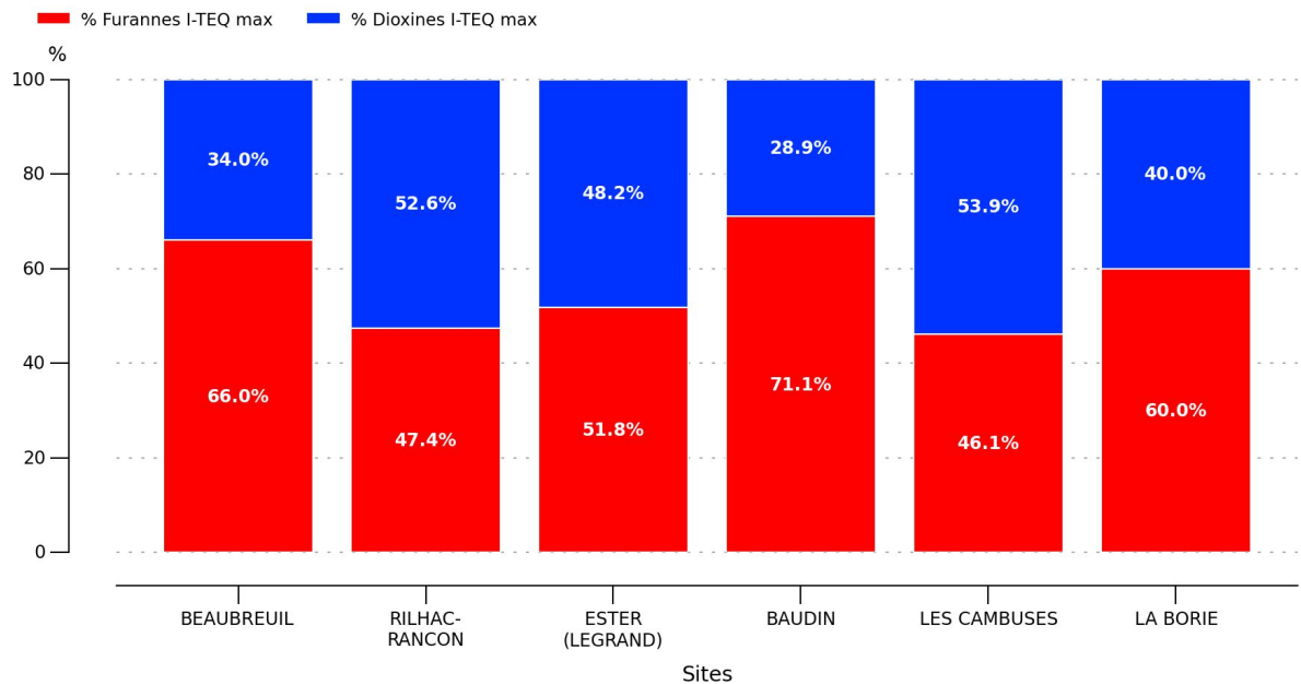
Illustration 9: Comparaison par site des rapports dioxines / furannes en concentration en équivalence toxique pour les 17 congénères
