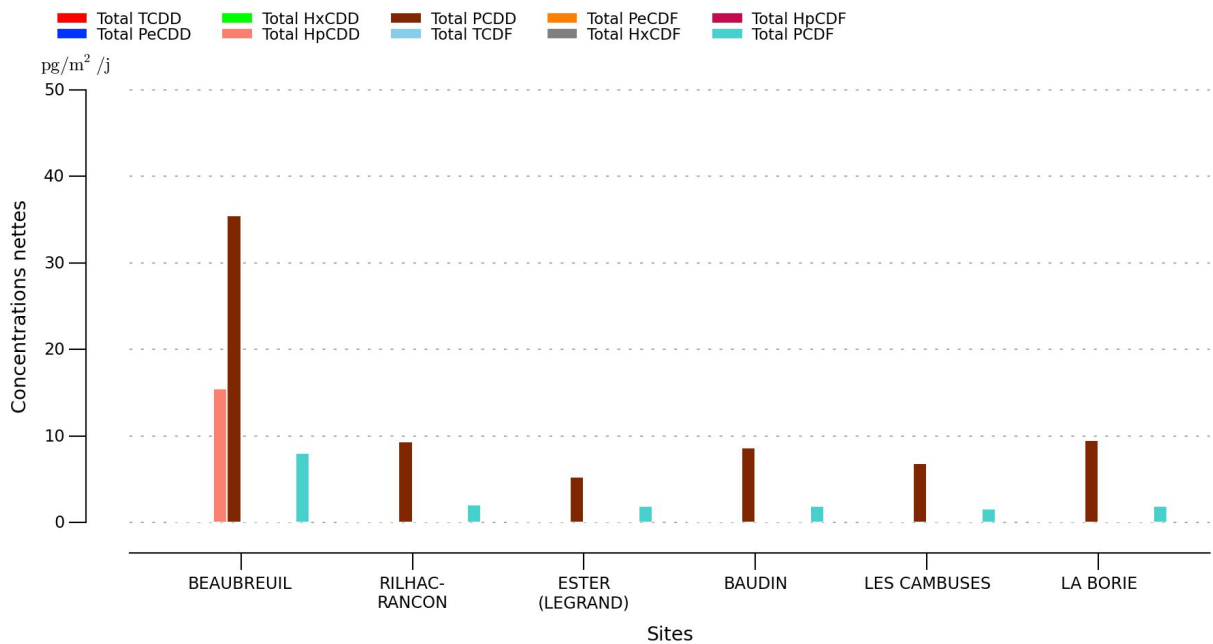
Illustration 5: Diagramme des concentrations nettes pour les familles d'homologues
