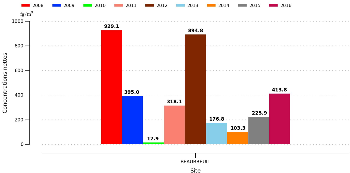
Illustration 12: Evolution annuelle du total des familles d'homologues en air ambiant
