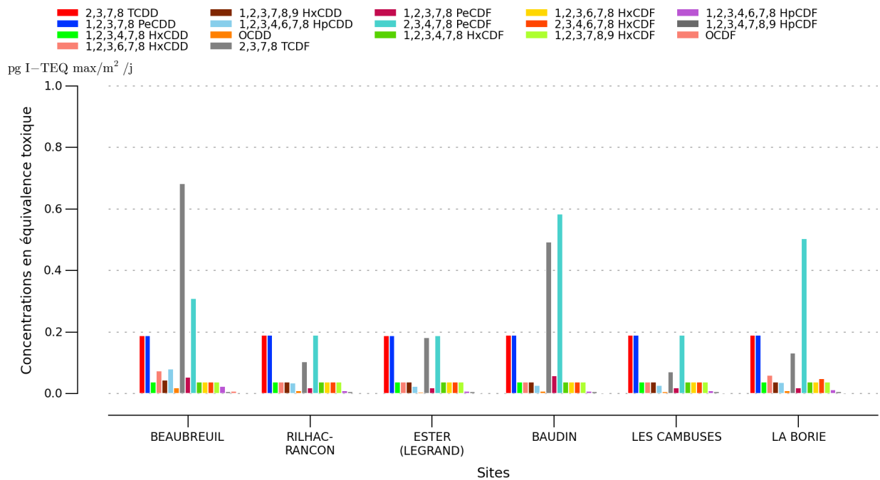
Illustration 8: Diagramme des concentrations en équivalence toxique des 17 congénères
