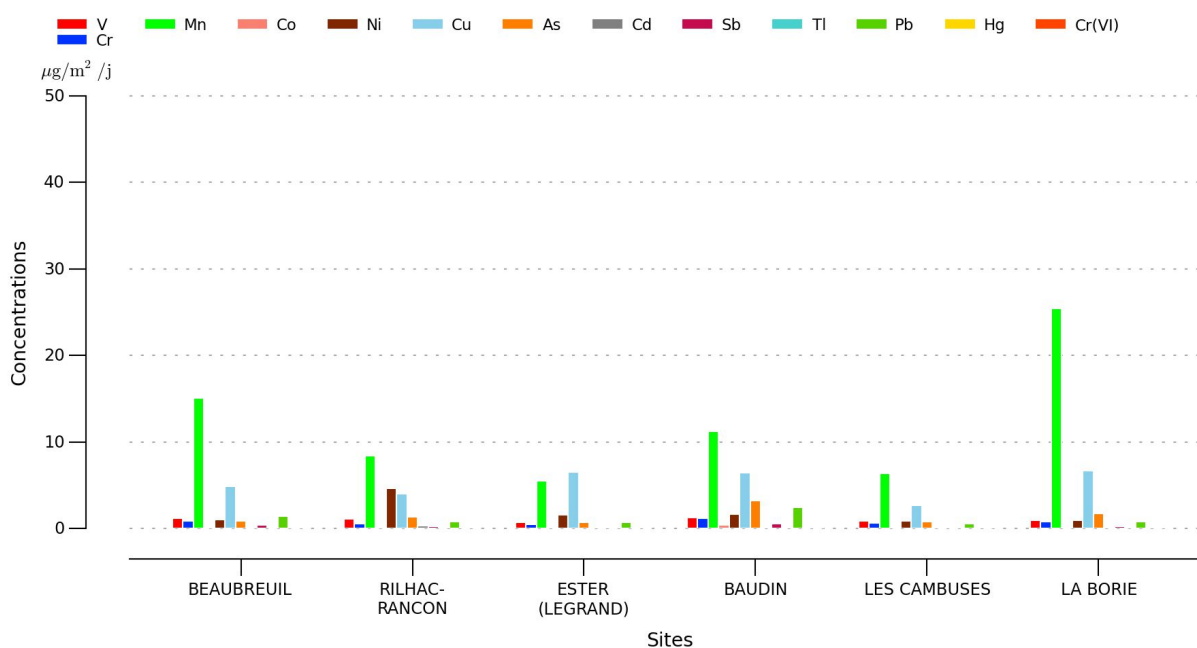
Illustration 16: Concentrations en métaux lourds dans les retombées atmosphériques
