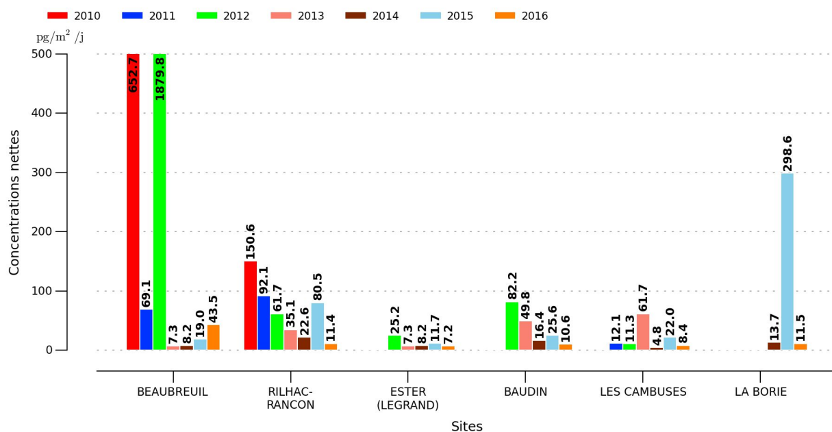
Illustration 7: Evolution annuelle du total des familles d'homologues dans les retombées atmosphériques
