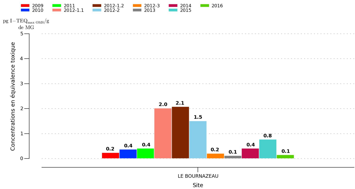
Illustration 15: Evolution annuelle du total des 17 congénères en équivalence toxique dans le lait de vache
