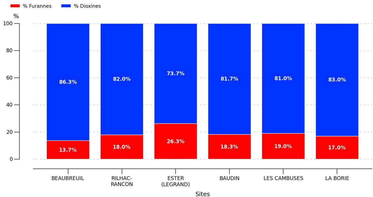
Illustration 6: Comparaison par site des rapport dioxines / furannes en concentrations nettes
