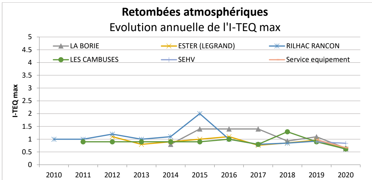
Figure 9 : Évolution annuelle du total des 17 congénères dans les retombées atmosphériques
