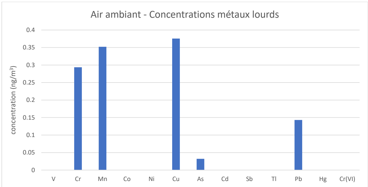
Figure 20 : Concentrations en métaux lourds dans l'air ambiant
