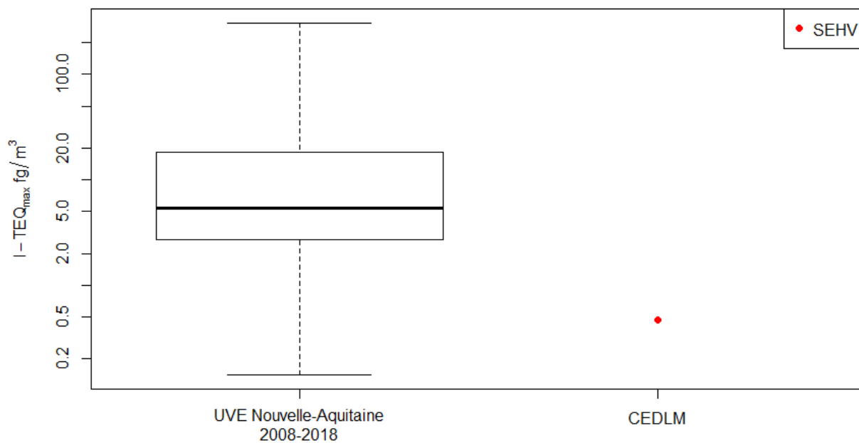
Figure 14 : Comparaison avec les concentrations en équivalent toxique en air ambiant d'UVE de la région Nouvelle-Aquitaine
