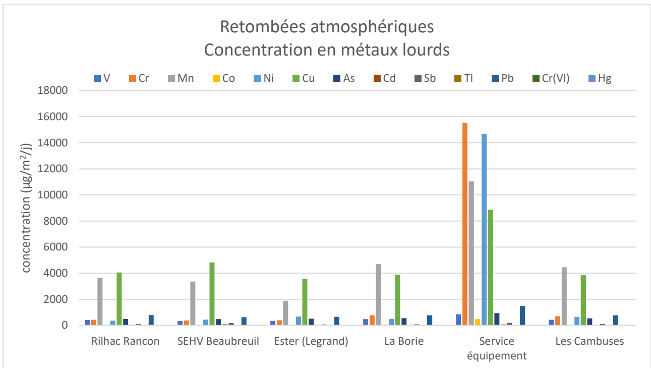
Figure 19 : Concentrations en métaux lourds dans les retombées atmosphériques
