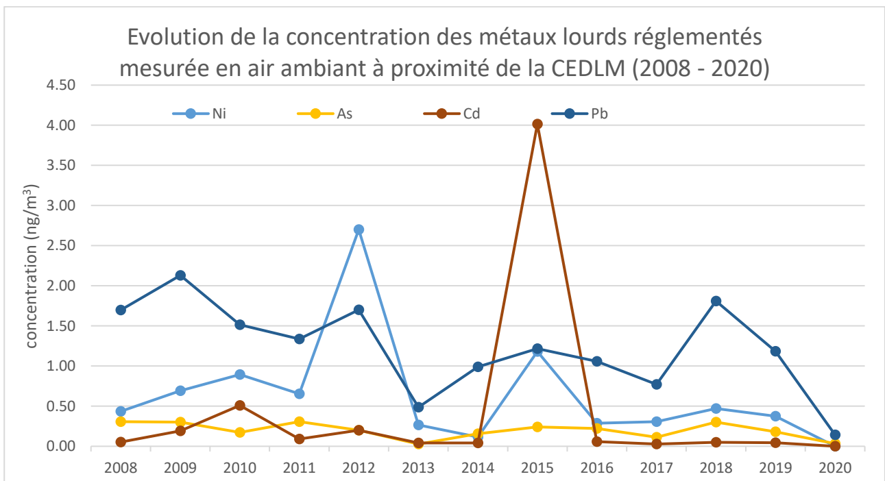
Figure 21 : Évolution de la concentration en air ambiant des métaux lourds réglementés mesurés à proximité de la CEDLM
