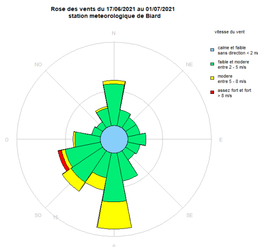
Figure 3 : Rose des vents du 17/06/2021 au 01/07/2021 station Biard
