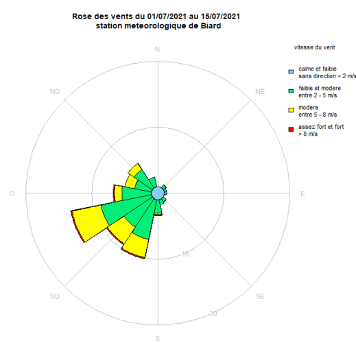
Figure 4 : Rose des vents du 01/07/2021 au 15/07/2021 station Biard
