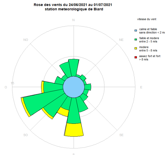
Figure 6 : Rose des vents du 24/06/2021 au 01/07/2021 – station Biard
