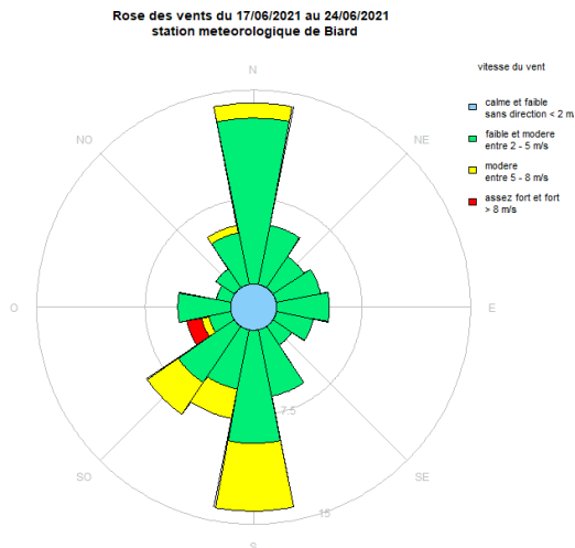
Figure 5 : Rose des vents du 17/06/2021 au 24/06/2021 – station Biard
