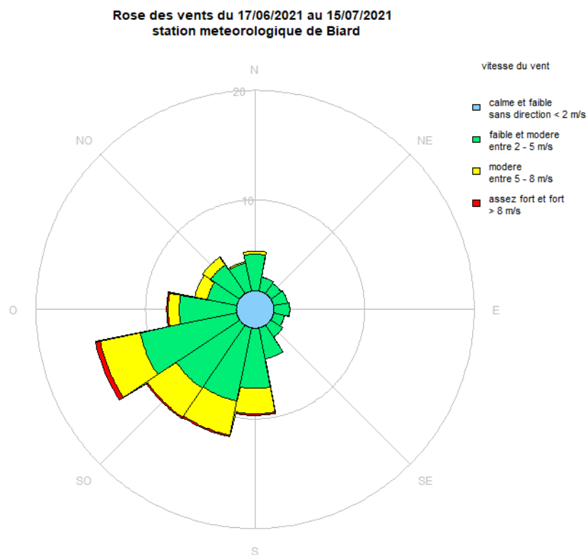
Figure 2 : Rose des vents du 17 juin au 15 juillet 2021 – station Biard
