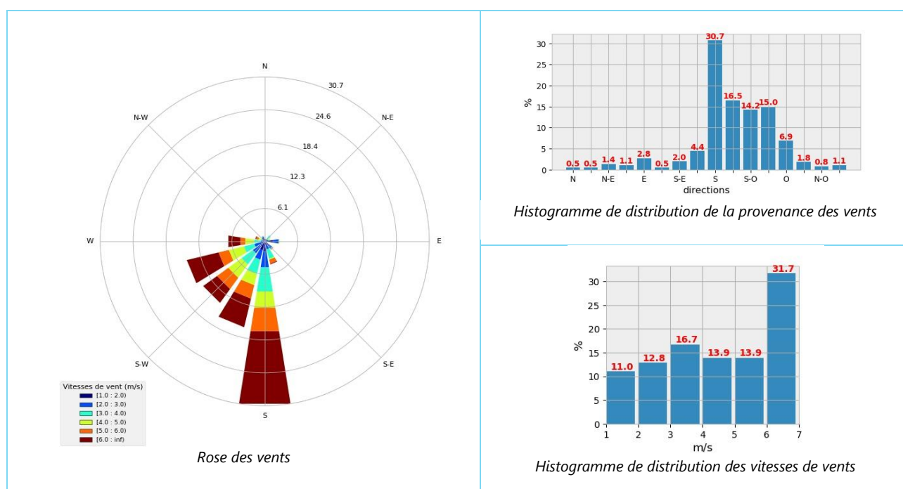
Figure 8 : Données météorologiques sur la période du 5/02 au 6/03/2020
