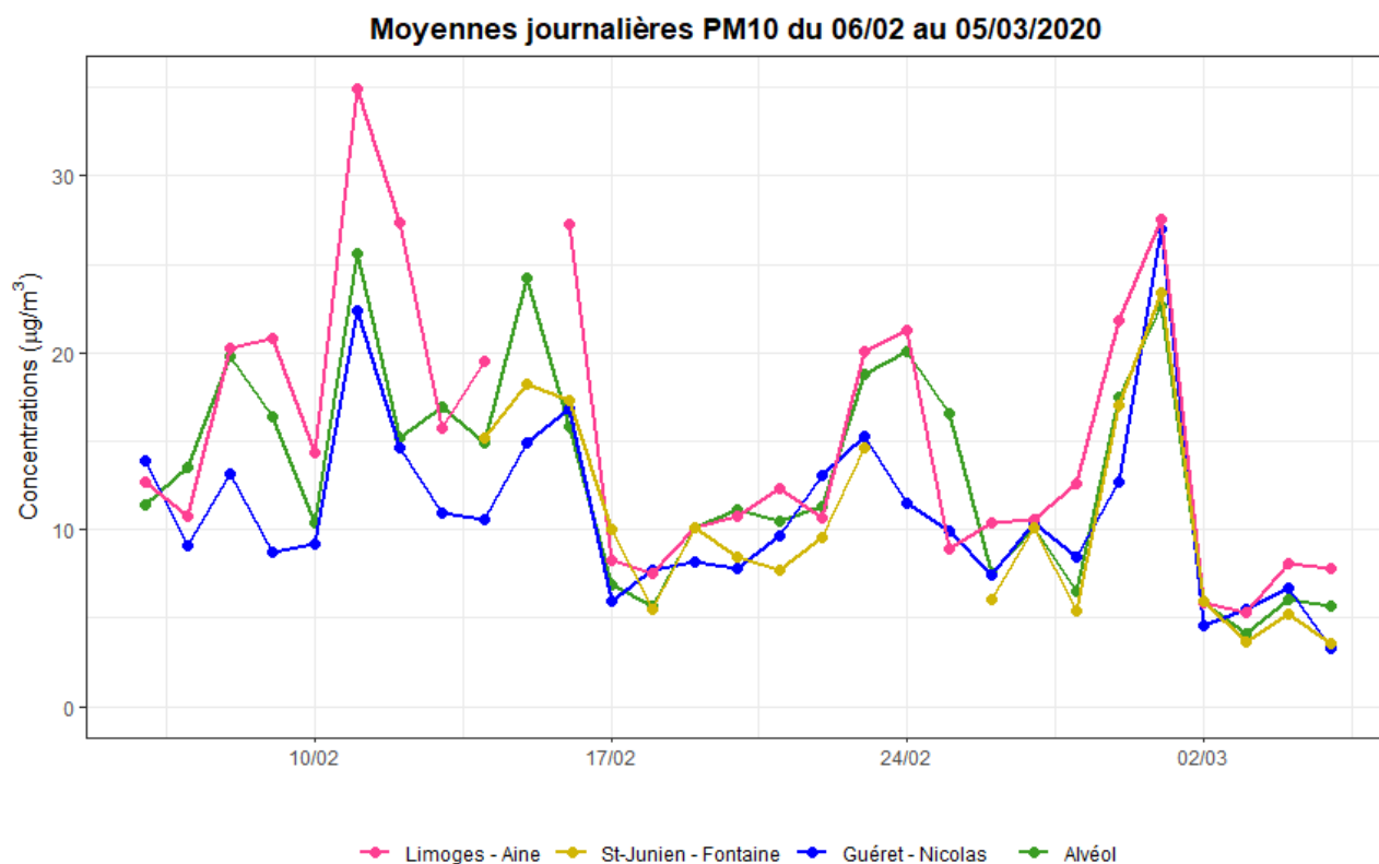
Figure 23 : Evolution des concentrations journalières de PM10
