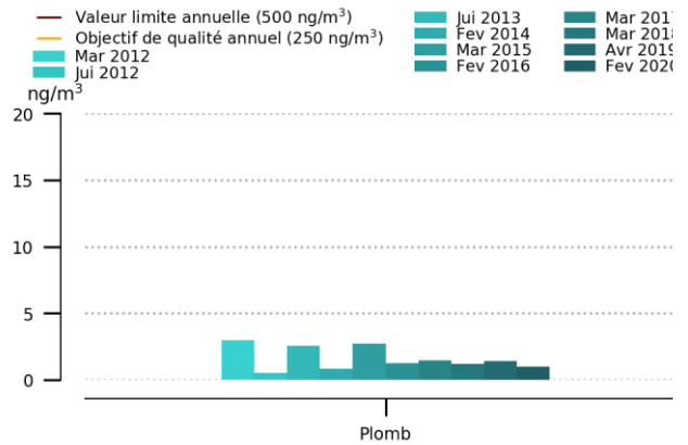
Figure 22 : Evolution des teneurs en plomb
