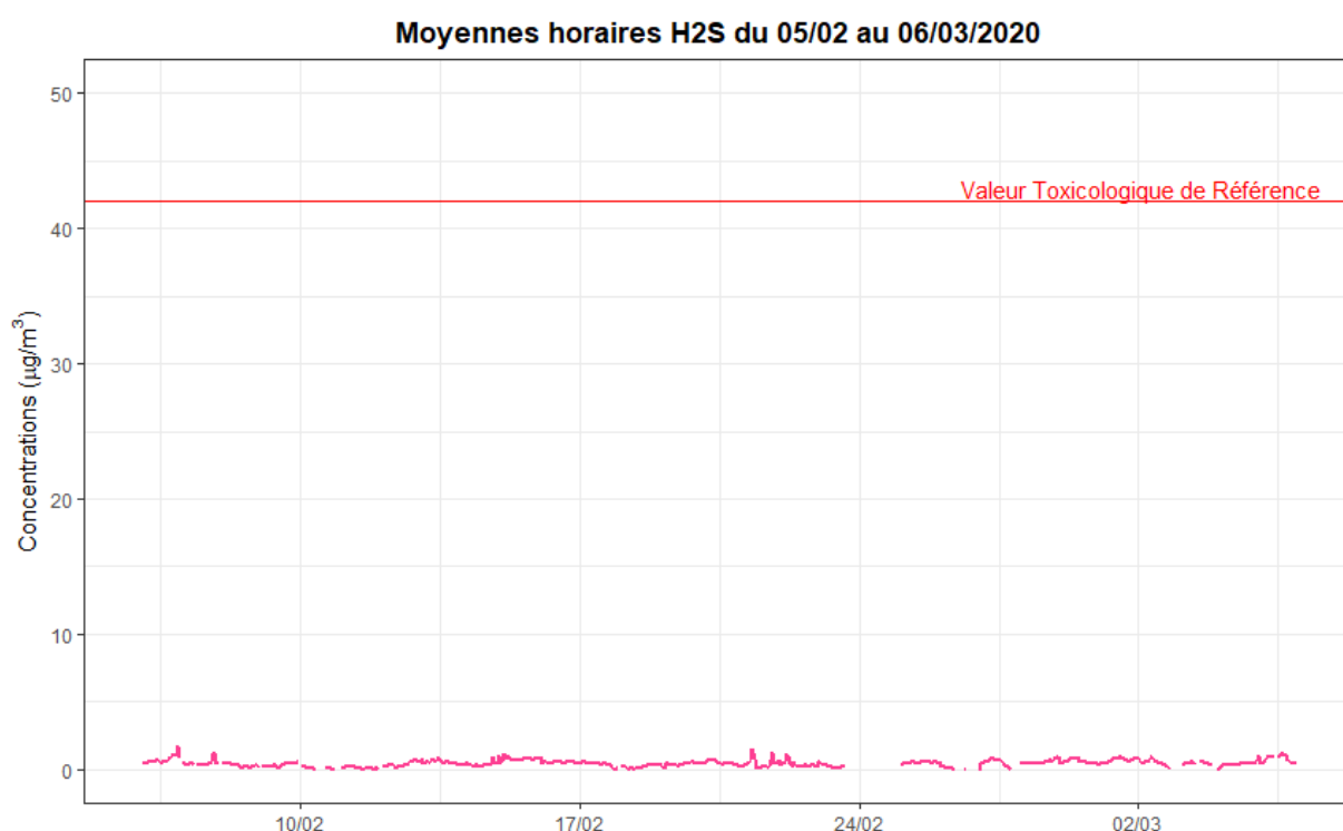
Figure 10 : Evolution des concentrations horaires d'H 2 S
