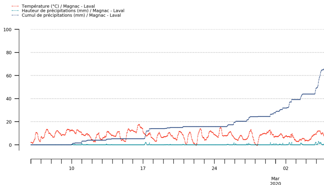
Figure 9 : Températures et hauteurs de précipitations horaires – 6/02 – 5/03/2020
