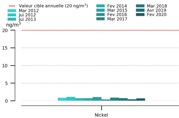
Figure 21 : Evolution des teneurs en nickel
