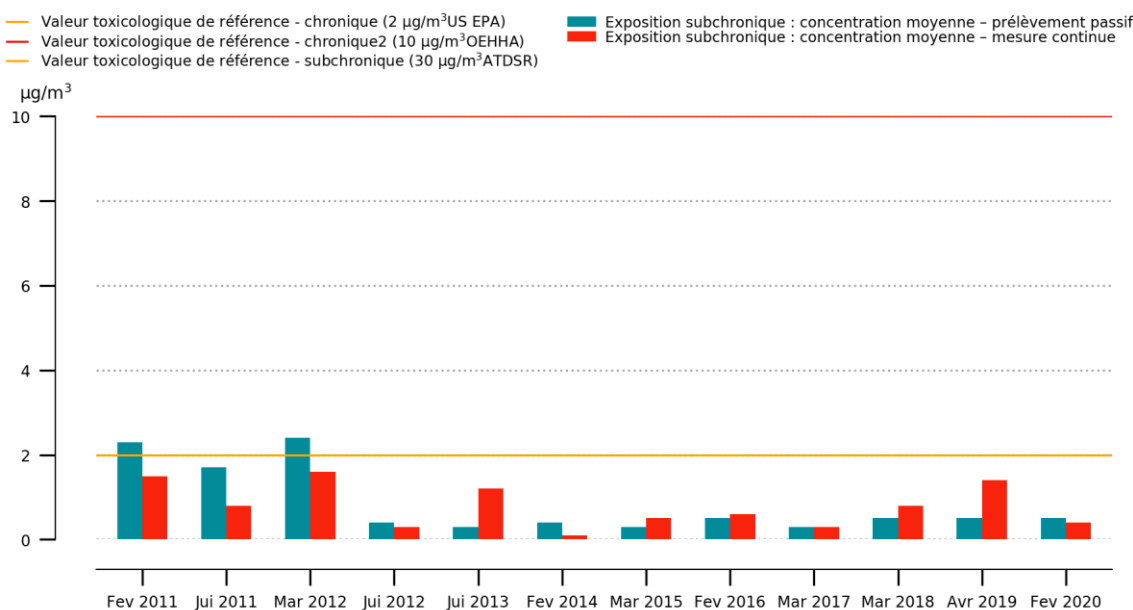
Figure 11 : Evolution des concentrations d'H 2 S en situation d'exposition subchronique
