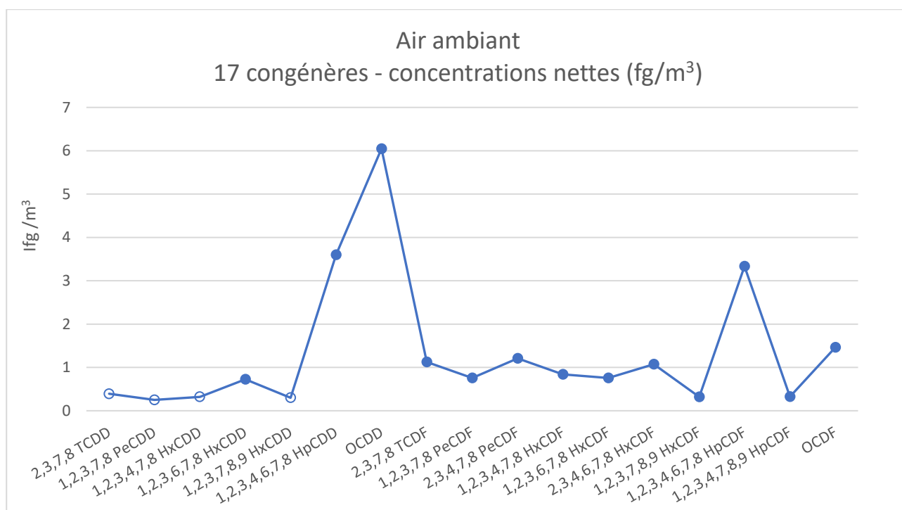
Figure 7 : Concentrations nettes des 17 congénères en air ambiant
