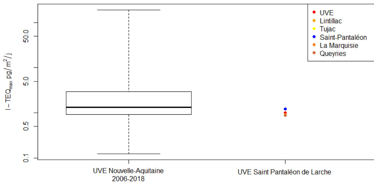
Figure 13 : Comparaison avec les concentrations mesurées en équivalent toxique dans les retombées atmosphériques sur la région Nouvelle-Aquitaine
