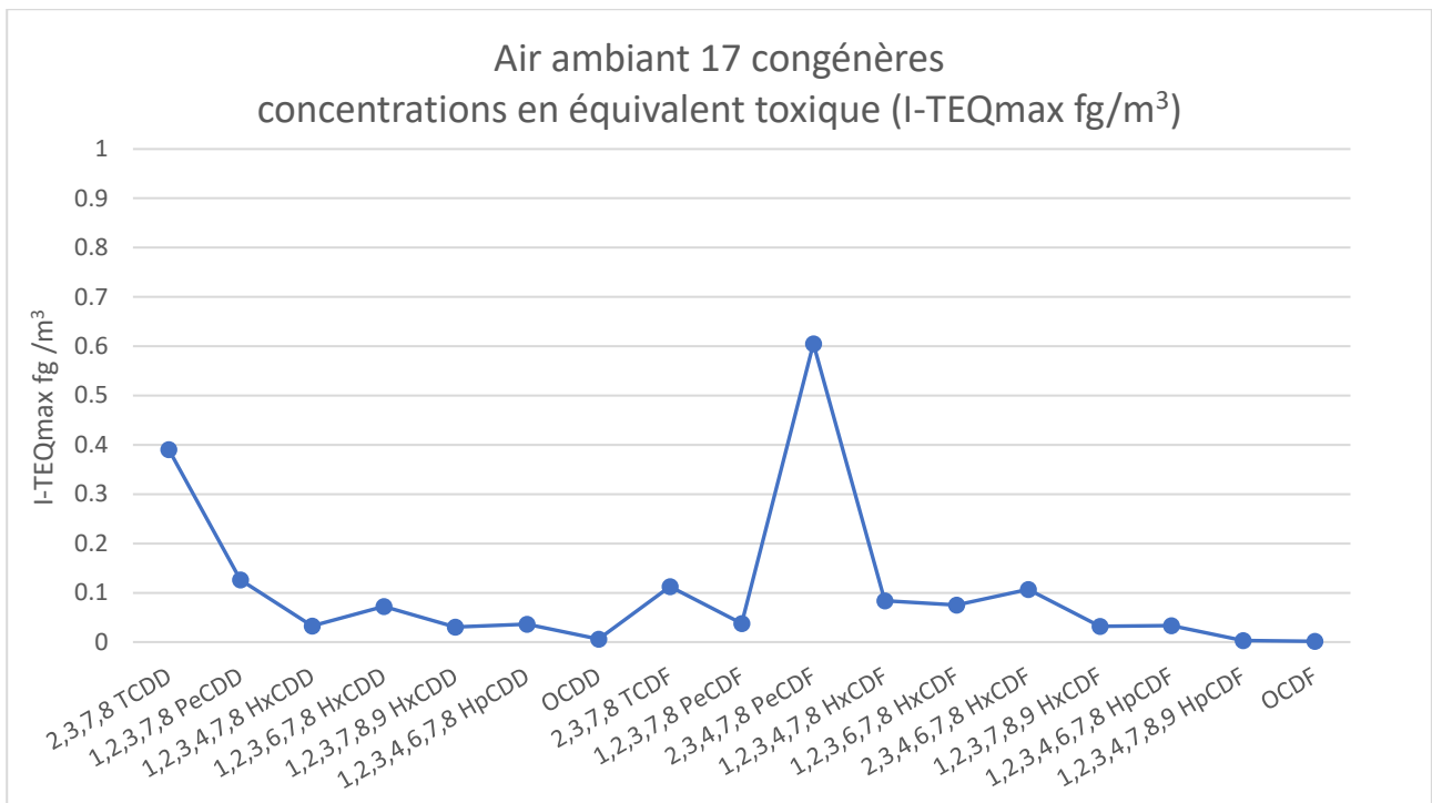
Figure 8 : Concentrations en équivalence toxique des 17 congénères en air ambiant
