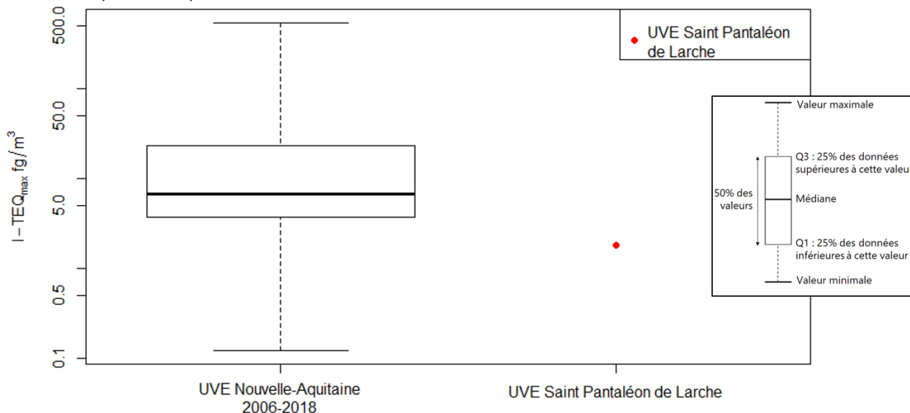
Figure 10 : Comparaison avec les concentrations mesurées en équivalent toxique en air ambiant sur la région Nouvelle-Aquitaine
