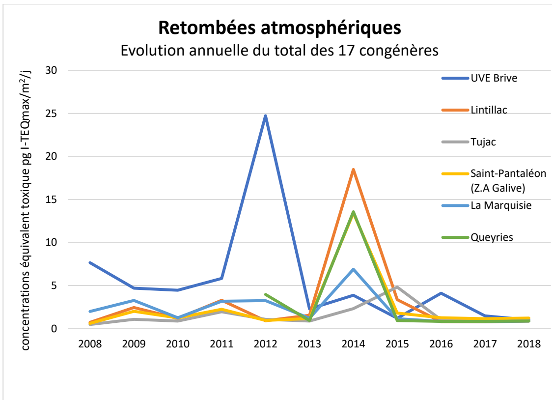
Figure 12 : Évolution annuelle de l'indice ITEQ dans les retombées atmosphériques
