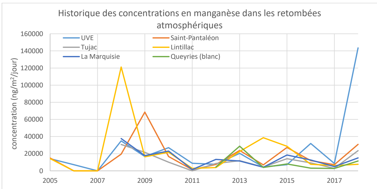
Figure 23 : Historique des concentrations en manganèse dans les retombées atmosphériques
