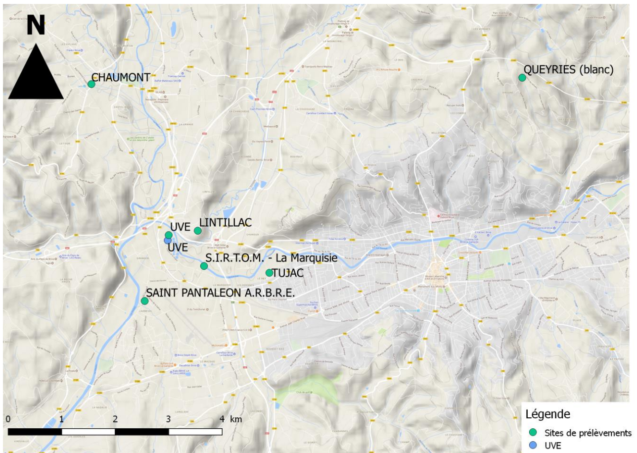
Figure 1 : Sites de mesure – UVE de Saint-Pantaléon-de-Larche
