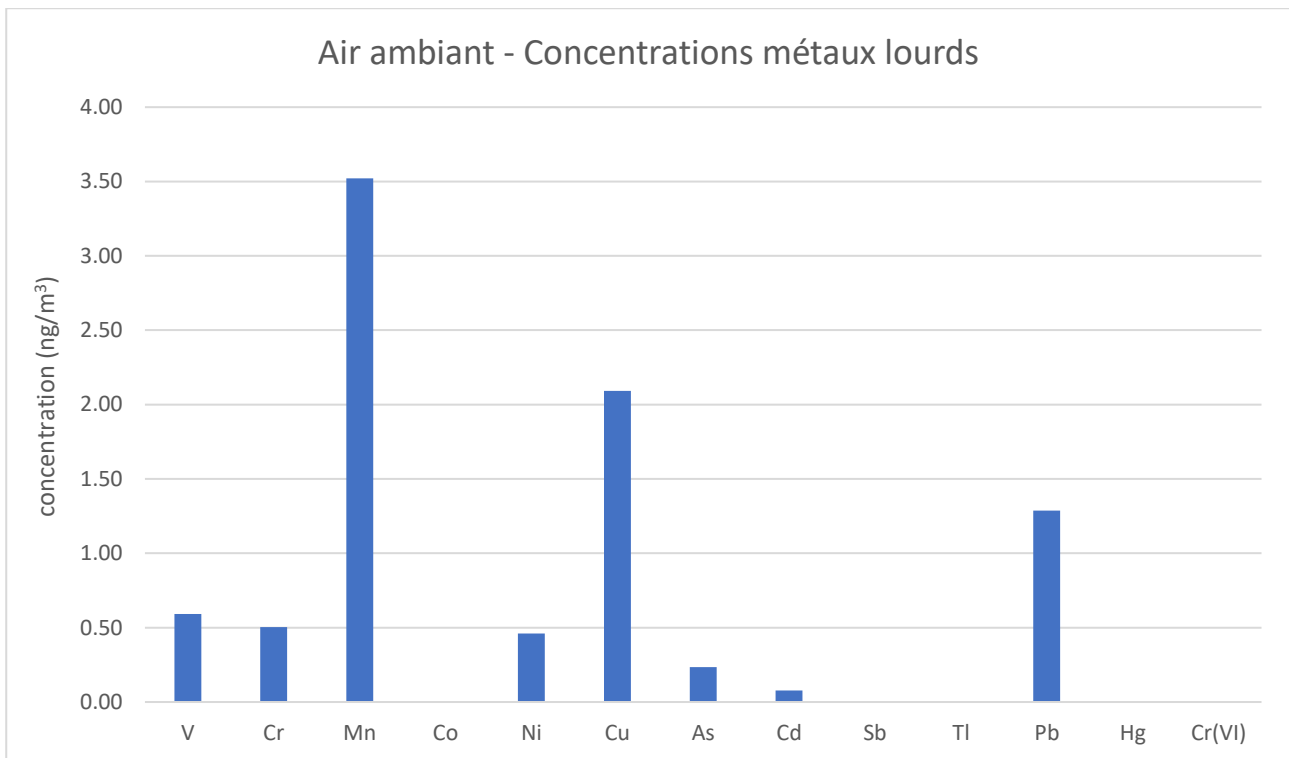
Figure 41 : Concentration en métaux lourds en air ambiant
