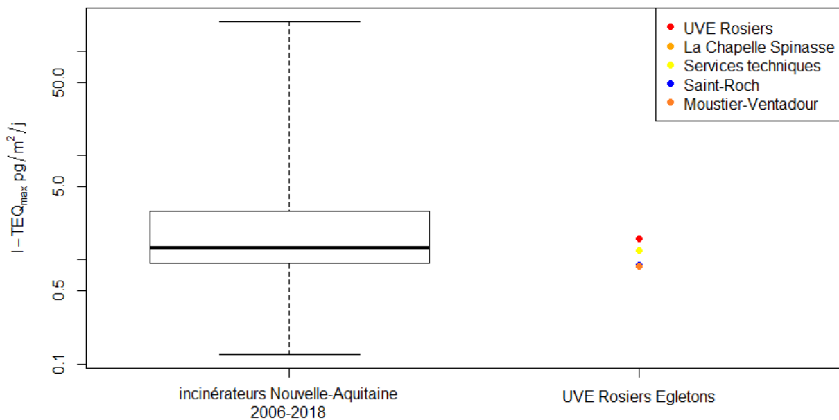
Figure 36 : Comparaison avec les concentrations mesurées en équivalent toxique dans les retombées atmosphériques sur la région Nouvelle-Aquitaine
