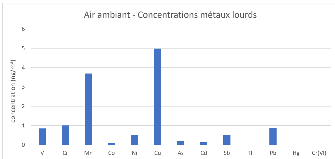
Figure 18 : Concentrations métaux lourds en air ambiant
