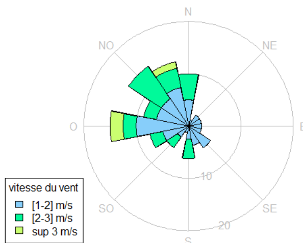
Figure 6 : Rose des vents du 12/09/2018 au 19/09/2018 station Brive
