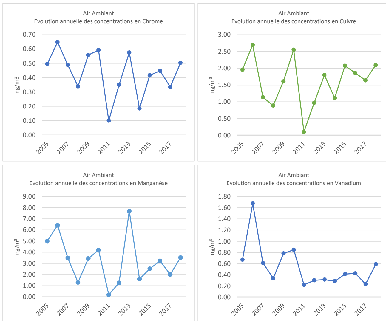
Figure 43 : Évolution des concentrations des métaux lourds non réglementés en air ambiant
