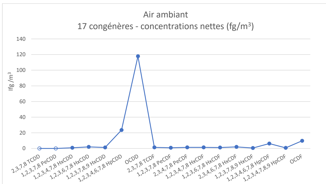
Figure 30 : Concentration nette des 17 congénères en air ambiant
