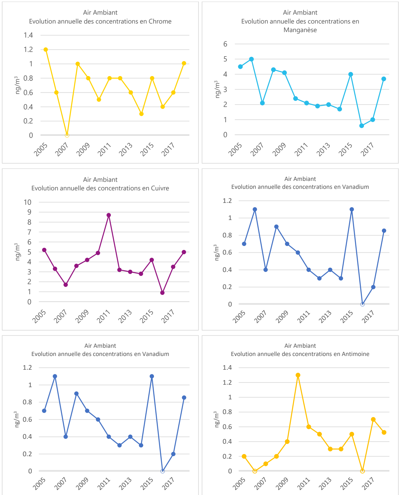
Figure 20 : Évolution des concentrations métaux lourds non réglementés en air ambiant
