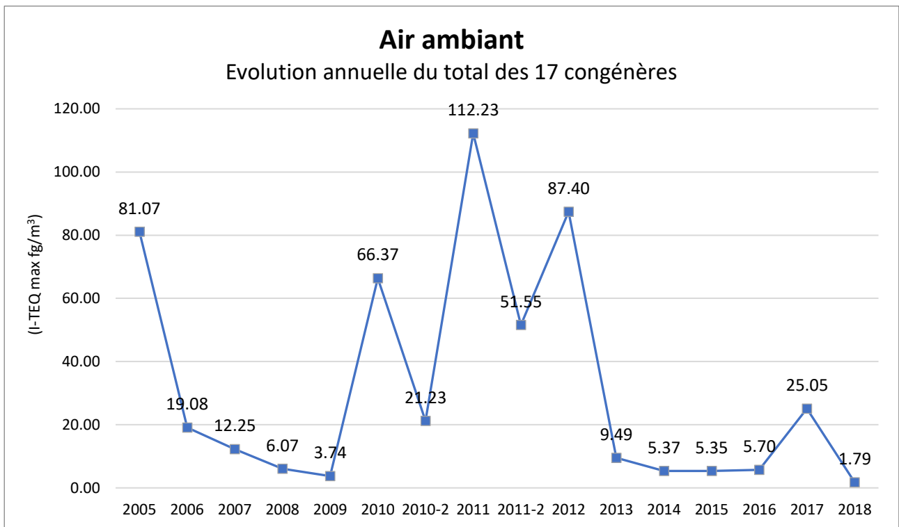
Figure 9 : Évolution annuelle des concentrations en équivalence toxique du total des 17 congénères
