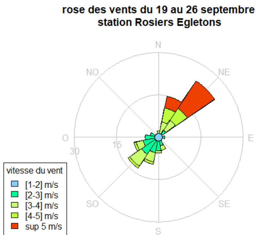
Figure 29 : : Rose des vents semaine de prélèvement en air ambiant
