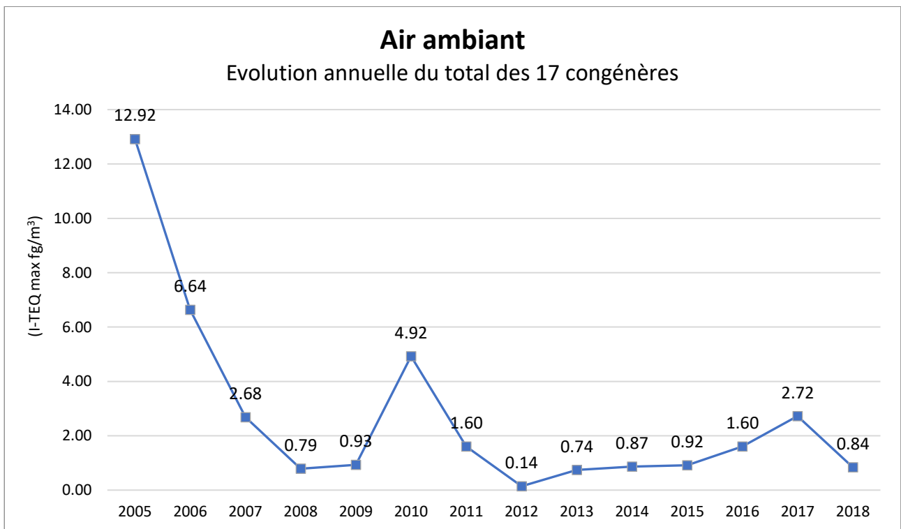
Figure 32 : Évolution annuelle des concentrations en équivalence toxique du total des 17 congénères
