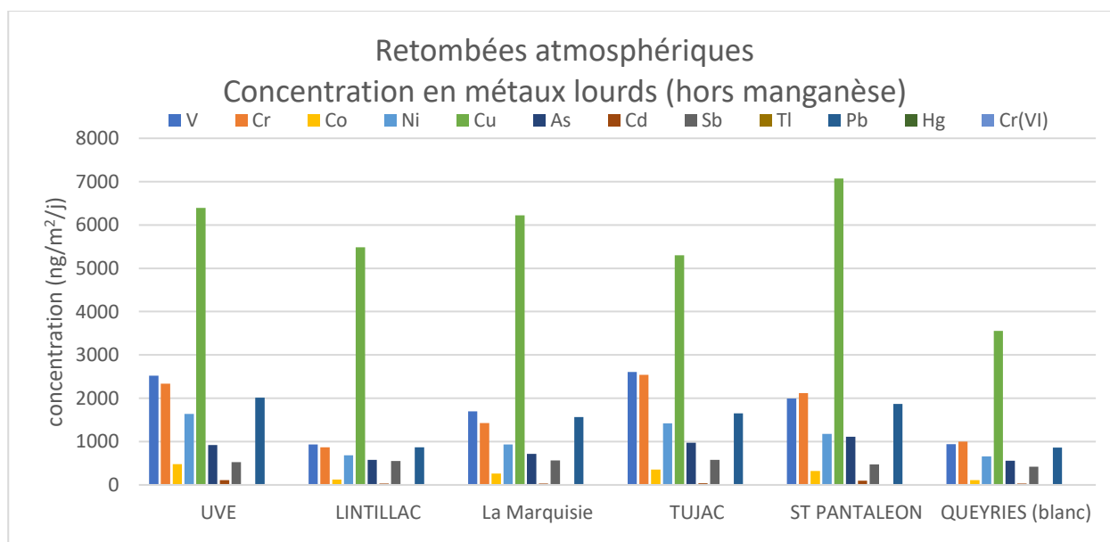
Figure 21 : Concentrations métaux lourds (hors manganèse) dans les retombées atmosphériques
