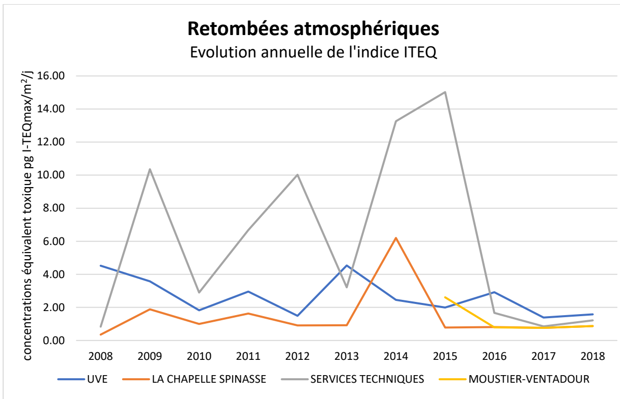
Figure 35 : Historique des concentrations du total des 17 congénères en équivalent toxique dans les retombées atmosphériques
