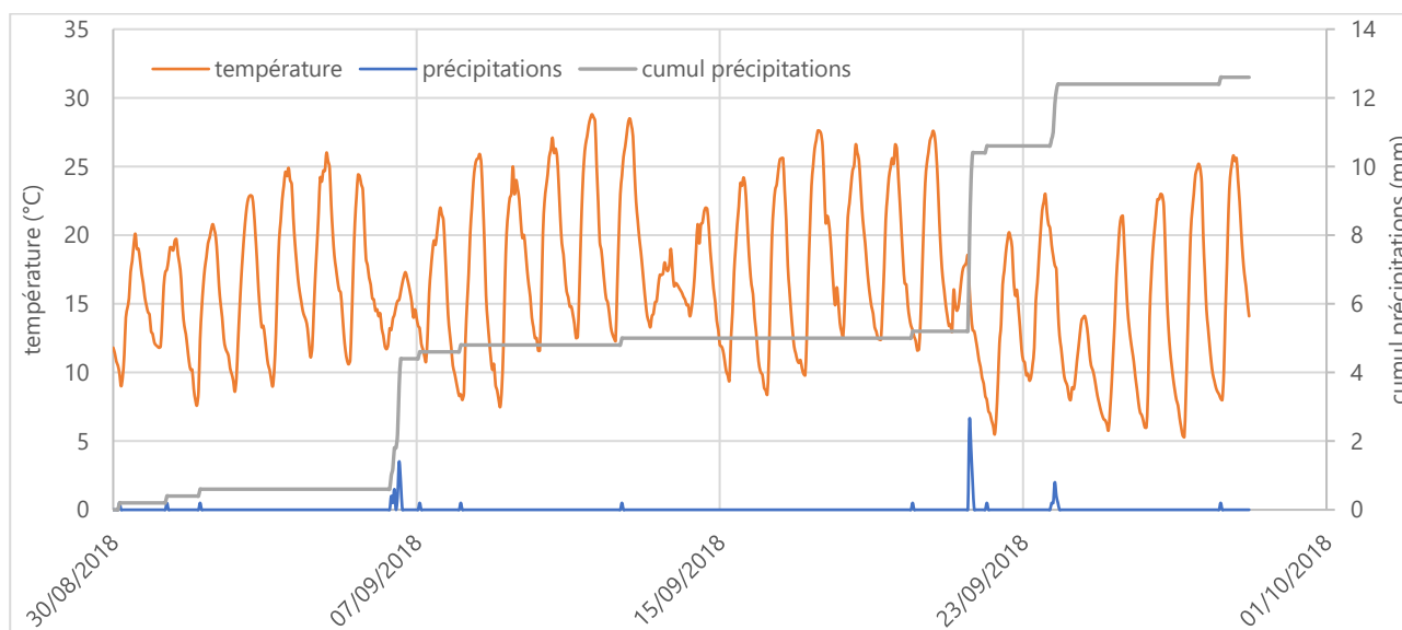
Figure 28 : Température et hauteur de précipitations horaires
