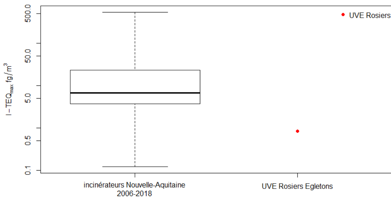
Figure 33 : Comparaison avec les concentrations mesurées en équivalent toxique en air ambiant sur la région Nouvelle-Aquitaine
