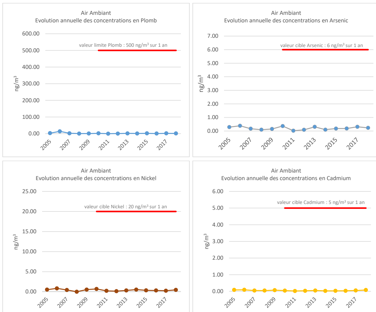
Figure 42 : Évolution des concentrations des métaux lourds réglementés en air ambient
