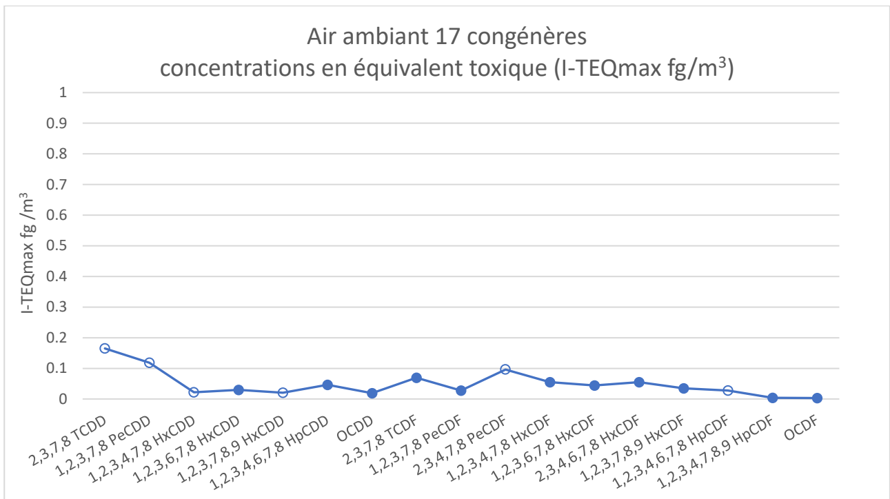
Figure 31 : Concentration en équivalence toxique des 17 congénères en air ambiant
