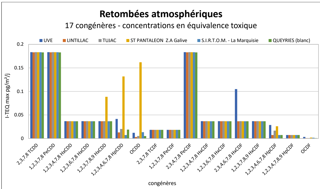
Figure 11 : Résultats d'analyses en équivalents toxiques des 17 congénères dans les retombées atmosphériques
