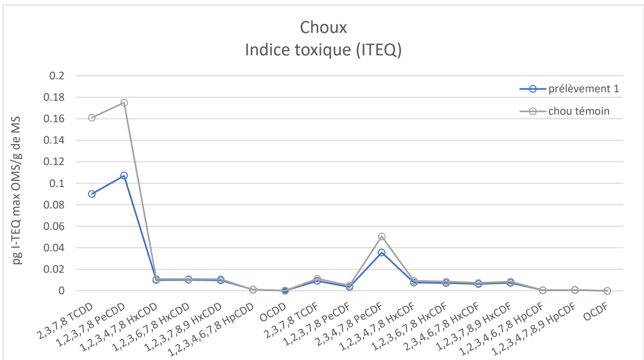
Figure 39 : Concentration des dioxines et furannes dans le chou exposé (en équivalent toxique par gramme de matière sèche)
