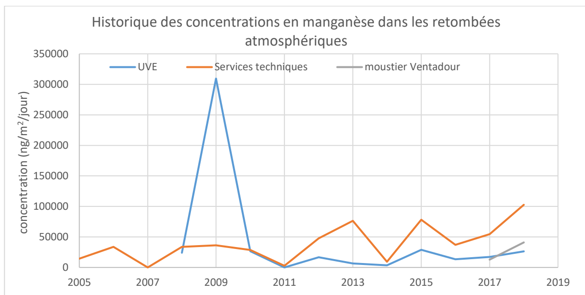
Figure 45 : Historique des concentrations en manganèse dans les retombées atmosphériques
