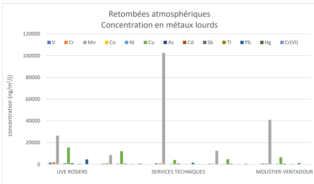
Figure 44 : Concentrations en métaux lourds dans les retombées atmosphériques
