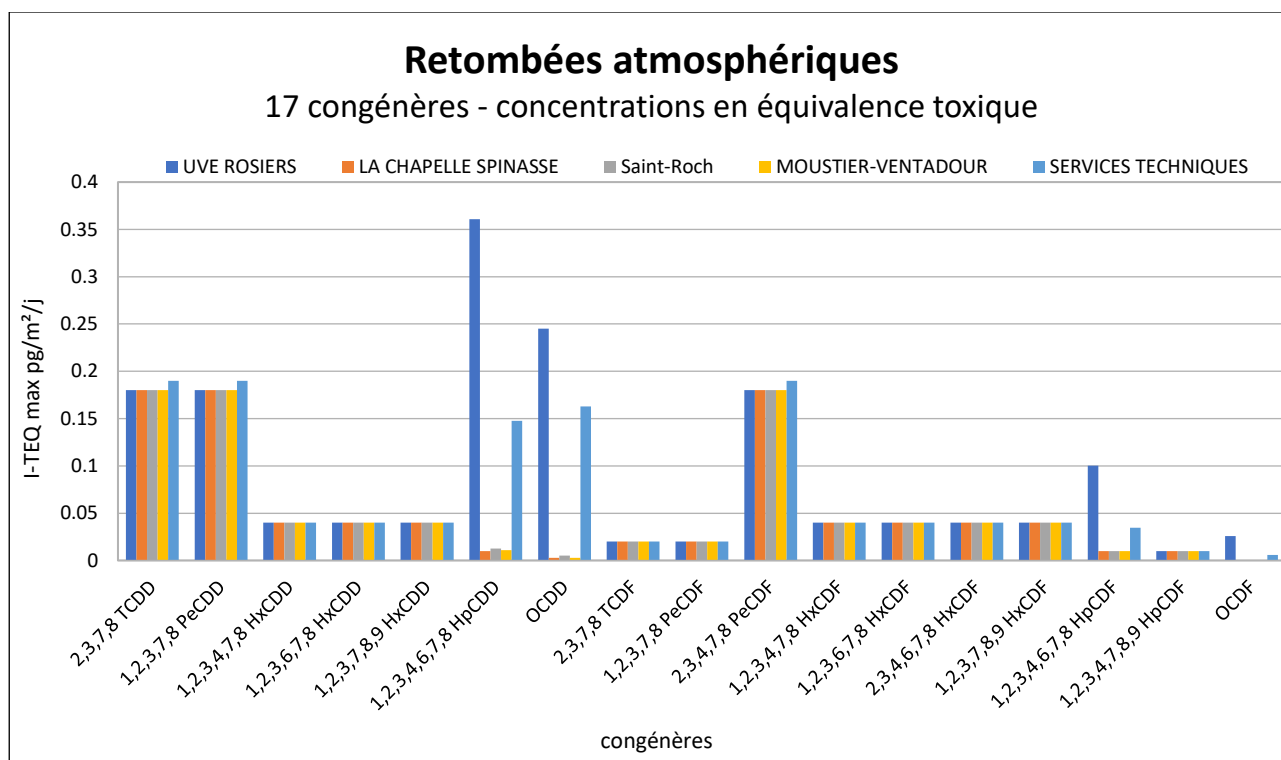
Figure 34 : Résultats d'analyses en équivalents toxiques des 17 congénères dans les retombées atmosphériques
