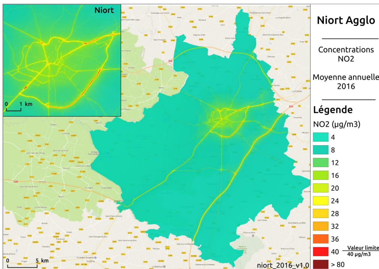
Figure 102: Modélisation des concentrations de NO 2 sur l'agglomération de Niort en 2016.
