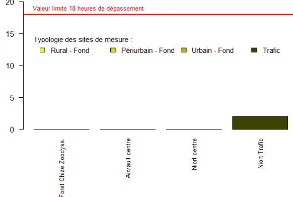
Figure 101 : Deux-Sèvres - Maxima des valeurs horaires et nombre d'heures de dépassement du seuil de 200 µg/m 3 en NO 2
