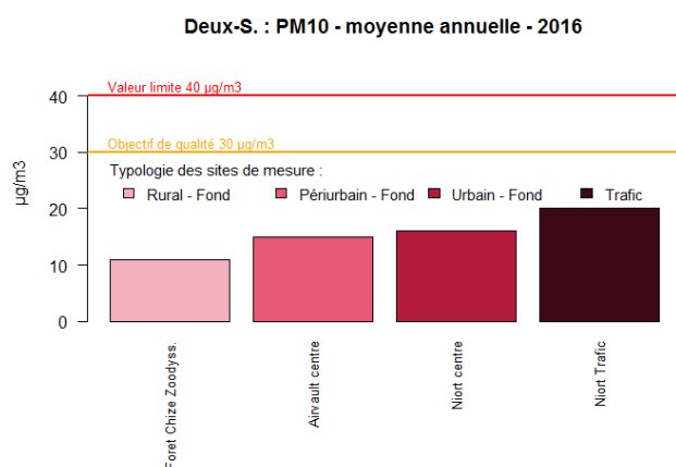
Figure 103 : Deux-Sèvres - Moyennes annuelles en PM10
