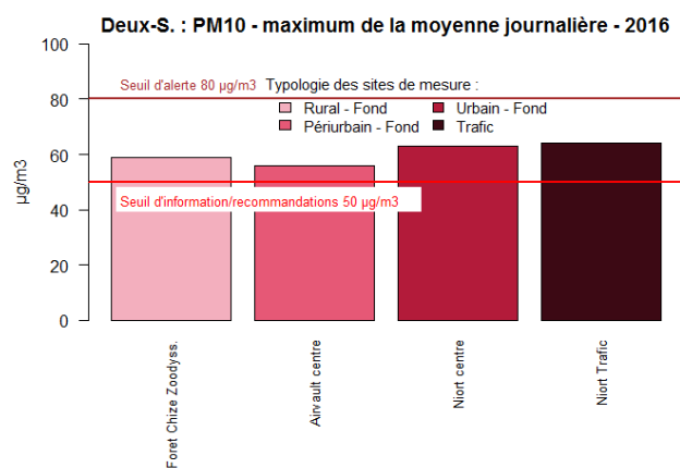
Figure 104 : Deux-S. - Maxima des valeurs journalières et nombre de jours de dépassement du seuil de 50 µg/m 3 en PM10
