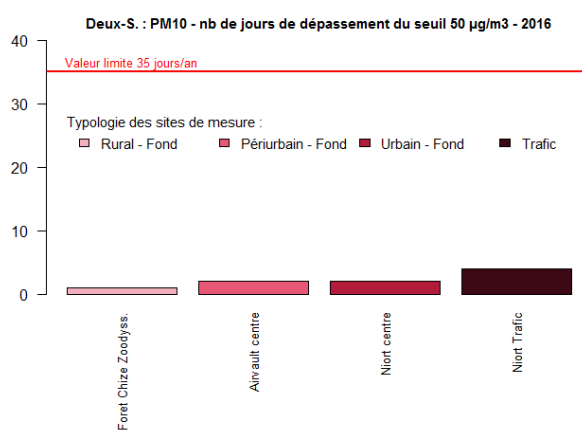
Figure 104 : Deux-S. - Maxima des valeurs journalières et nombre de jours de dépassement du seuil de 50 µg/m 3 en PM10
