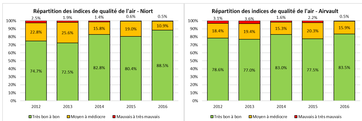
Figure 99 : Deux-Sèvres - Répartition des indices de qualité de l'air depuis 2012
