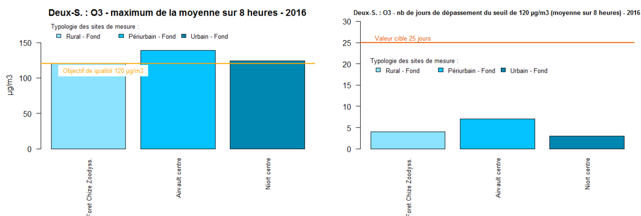
Figure 108 : Deux-S. - Max des moy. sur 8 h et nb moyen sur 3 ans de j de dépassement du seuil de 120 µg/m 3 sur 8 h en O 3
