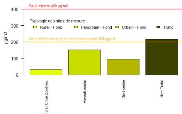
Figure 101 : Deux-Sèvres - Maxima des valeurs horaires et nombre d'heures de dépassement du seuil de 200 µg/m 3 en NO 2
