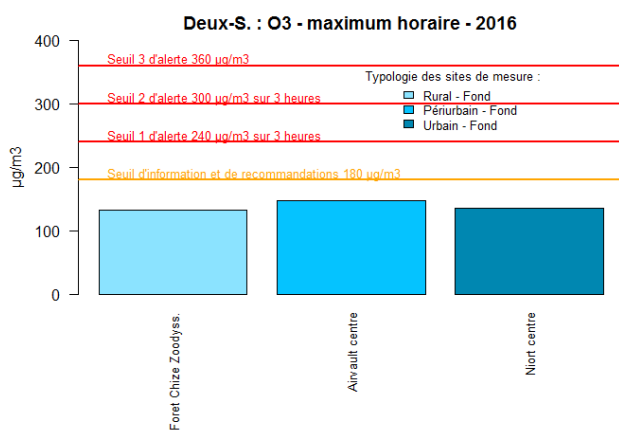
Figure 107 : Deux-Sèvres - Maxima horaires en O 3
