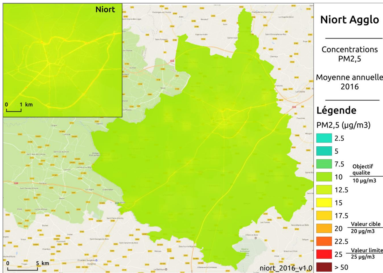
Figure 106: Modélisation des concentrations de PM 2,5 sur l'agglomération de Niort en 2016.
