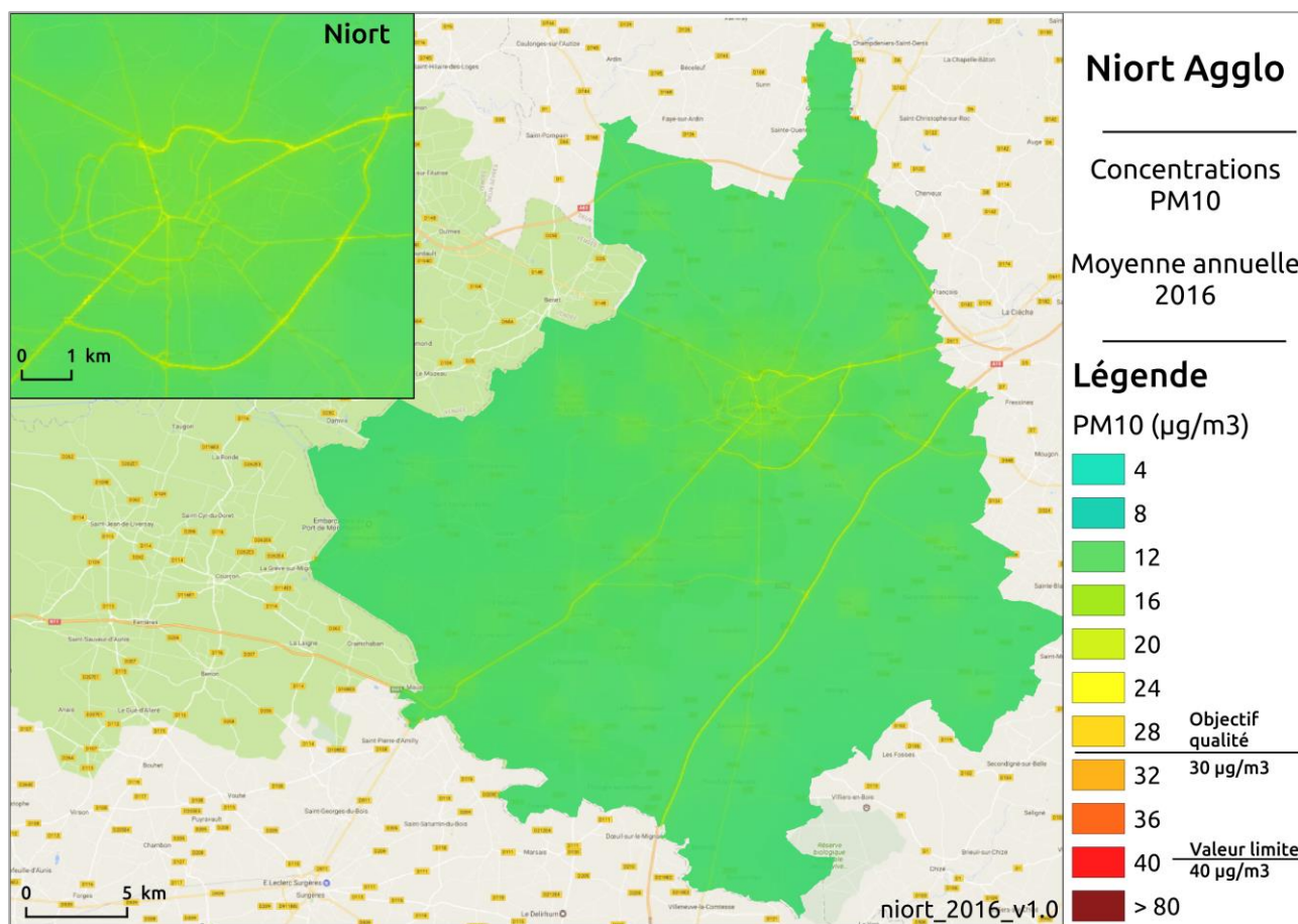
Figure 105: Modélisation des concentrations de PM10 sur l'agglomération de Niort en 2016.
