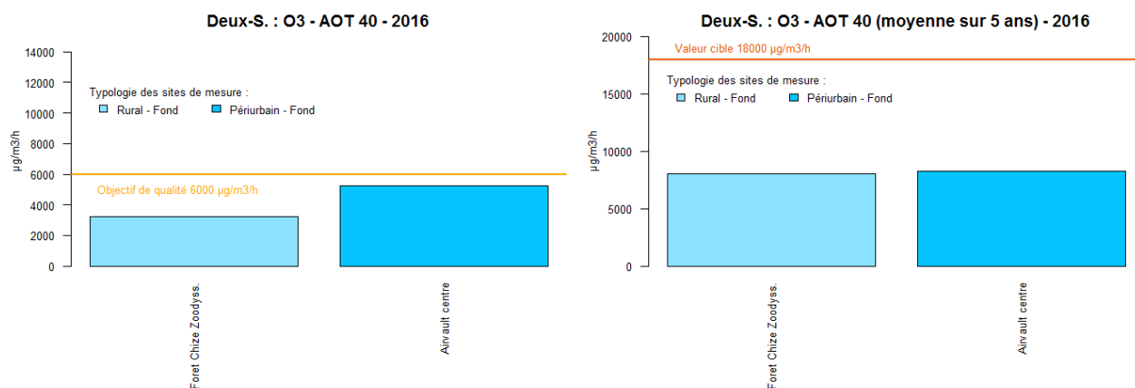
Figure 109 : Deux-Sèvres - AOT40 et moyenne des AOT40 sur 5 ans en O 3
