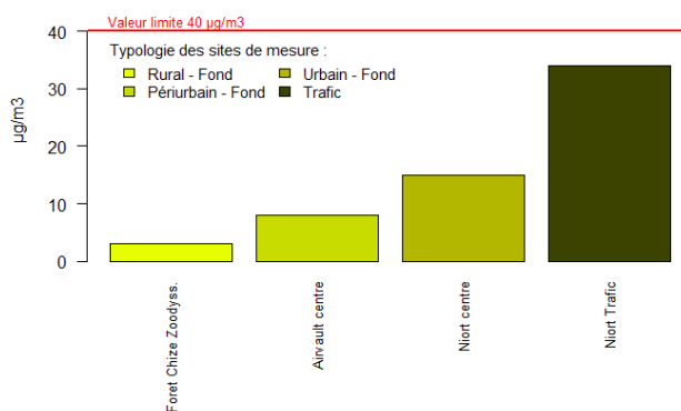
Figure 100 : Deux-Sèvres - Moyennes annuelles en NO 2
