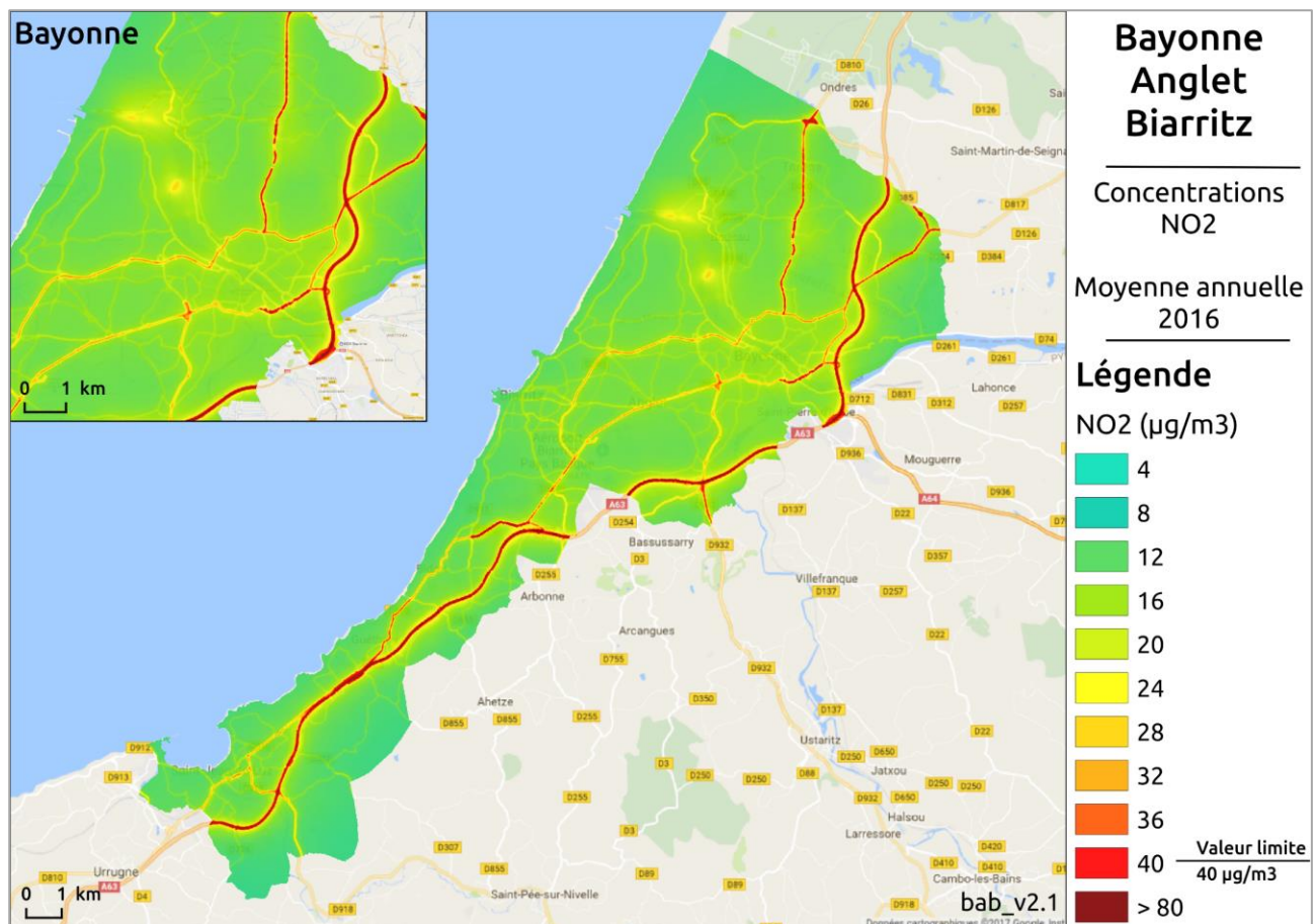
Figure 88: Modélisation des concentrations de NO 2 sur l'agglomération BAB en 2016.
