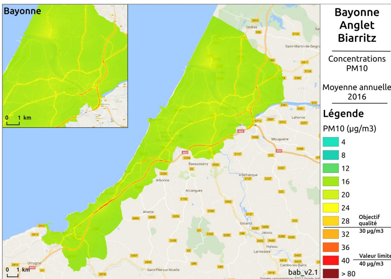
Figure 91: Modélisation des concentrations de PM10 sur l'agglomération du BAB en 2016.
