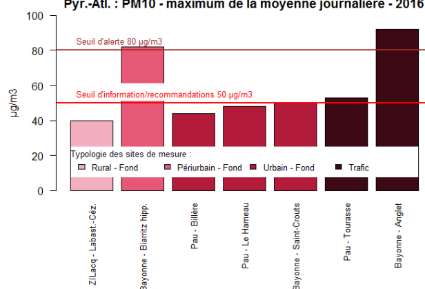
Figure 90 : Pyr.-Atl. - Maxima des valeurs journalières et nombre de jours de dépassement du seuil de 50 µg/m 3 en PM10
