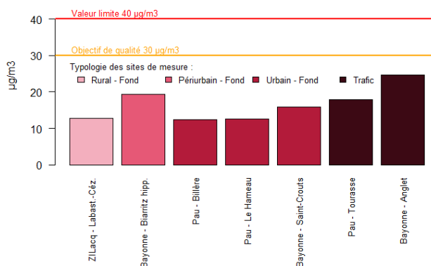
Figure 89 : Pyrénées-Atlantiques - Moyennes annuelles en PM10
