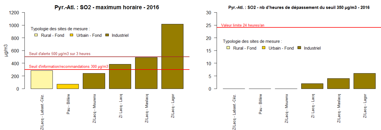
Figure 98 : Pyr.-Atl. - Maxima des valeurs horaires et nombre d'heures de dépassement du seuil de 350 µg/m 3 en SO 2
