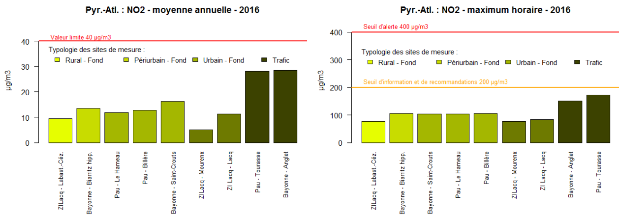
Figure 87 : Pyrénées-Atlantiques - Moyennes annuelles et maxima horaires en NO 2
