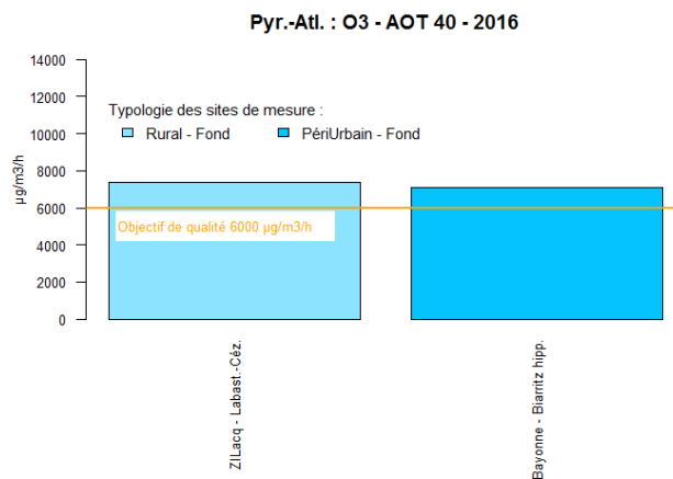
Figure 96 : Pyrénées-Atlantiques – AOT40 en O 3
