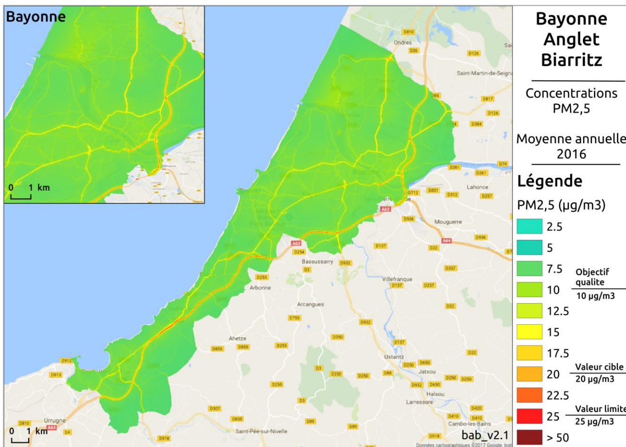
Figure 93: Modélisation des concentrations de PM 2,5 sur l'agglomération du BAB en 2016.
