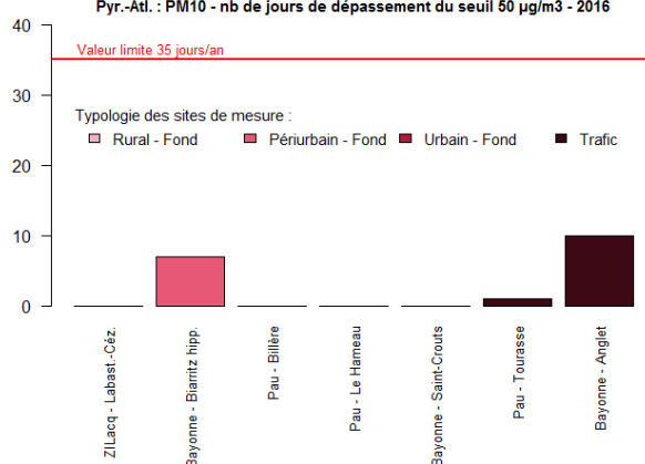
Figure 90 : Pyr.-Atl. - Maxima des valeurs journalières et nombre de jours de dépassement du seuil de 50 µg/m 3 en PM10
