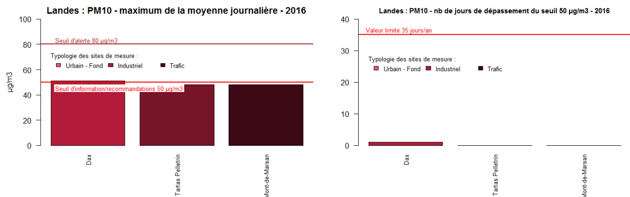
Figure 80 : Landes - Maxima des valeurs journalières et nombre de jours de dépassement du seuil de 50 µg/m 3 en PM10
