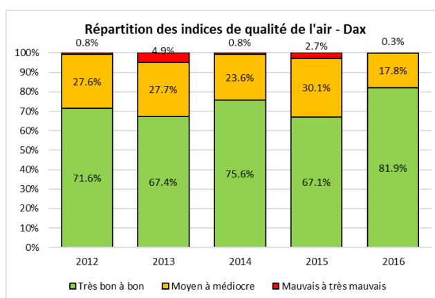
Figure 77 : Landes - Répartition des indices de qualité de l'air depuis 2012
