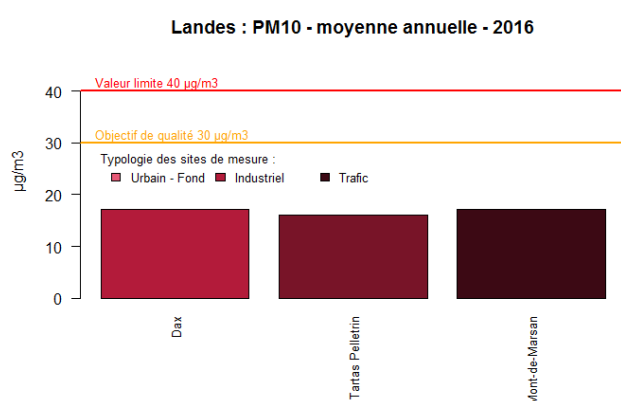
Figure 79 : Landes - Moyennes annuelles en PM10
