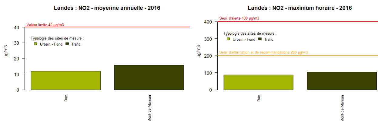
Figure 78 : Landes - Moyennes annuelles et maxima horaires en NO 2
