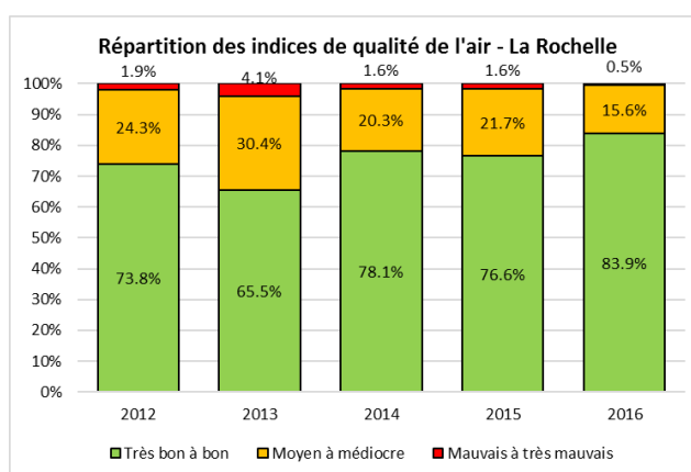
Figure 43 : Charente-Maritime - Répartition des indices de qualité de l'air depuis 2012
