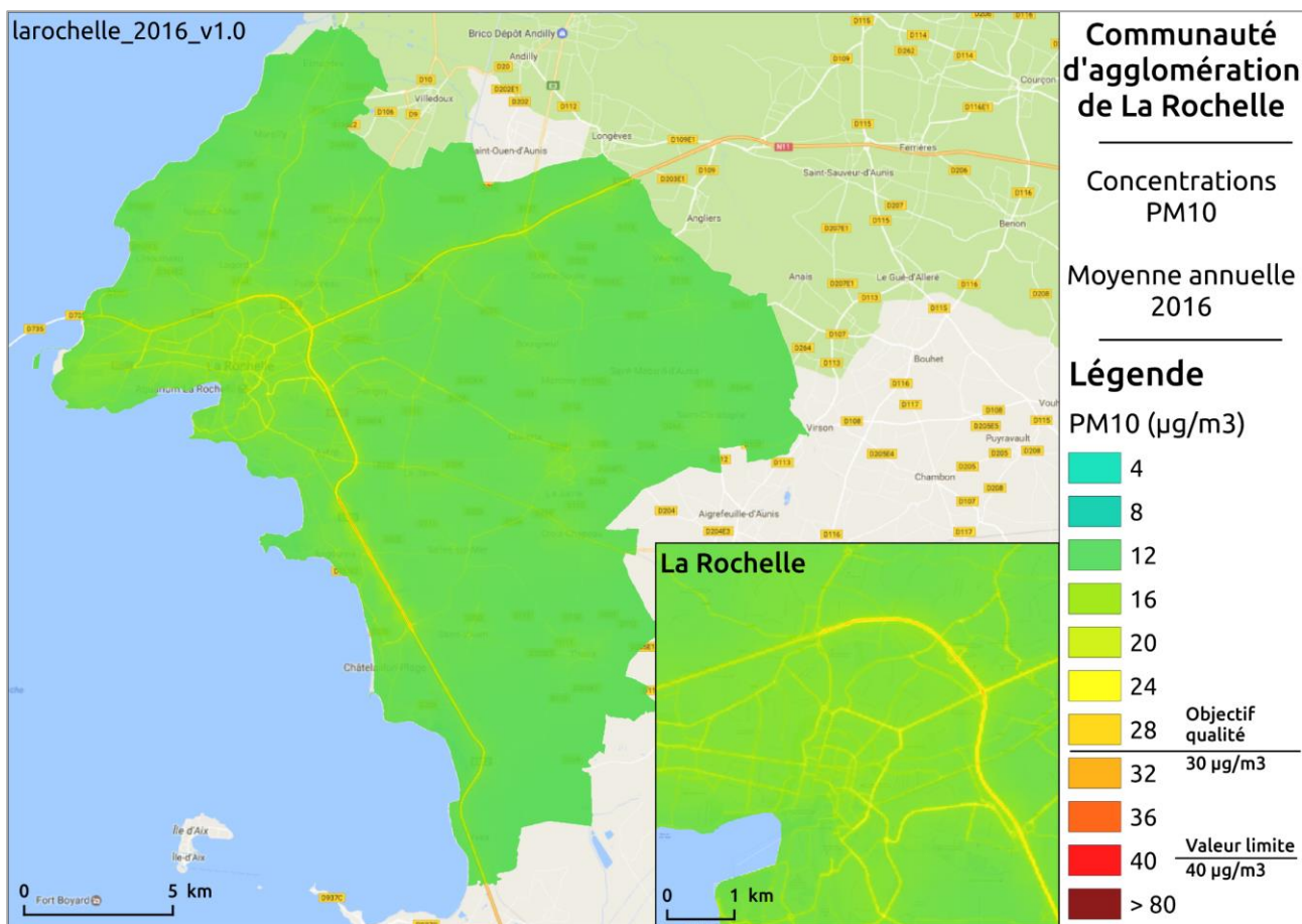
Figure 48: Modélisation des concentrations de PM10 sur l'agglomération de La Rochelle en 2016.
