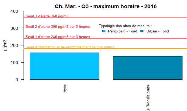
Figure 51 : Charente-Maritime - Maxima horaires en \text{O}_3
