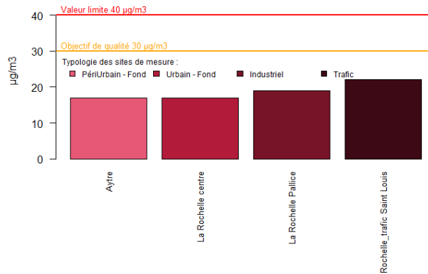
Figure 46 : Charente-Maritime - Moyennes annuelles en PM10
