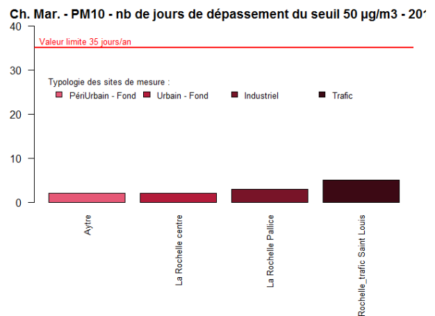
Figure 47 : Char.-Mar. - Maxima des valeurs journalières et nombre de jours de dépassement du seuil de 50 µg/m³ en PM10
