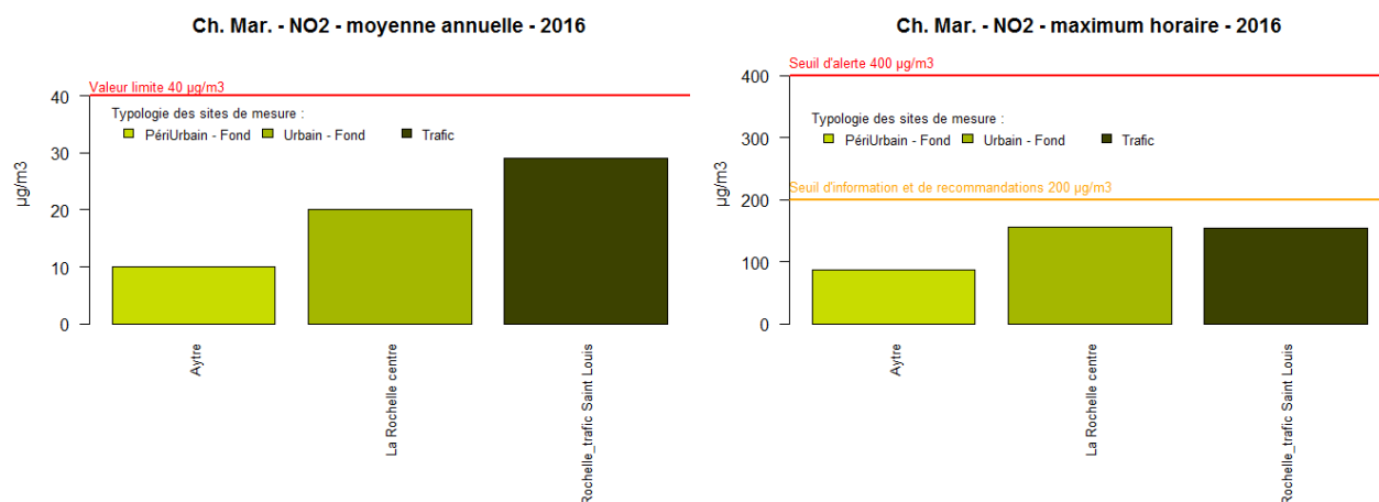
Figure 44 : Charente-Maritime - Moyennes annuelles et maxima horaires en NO 2
