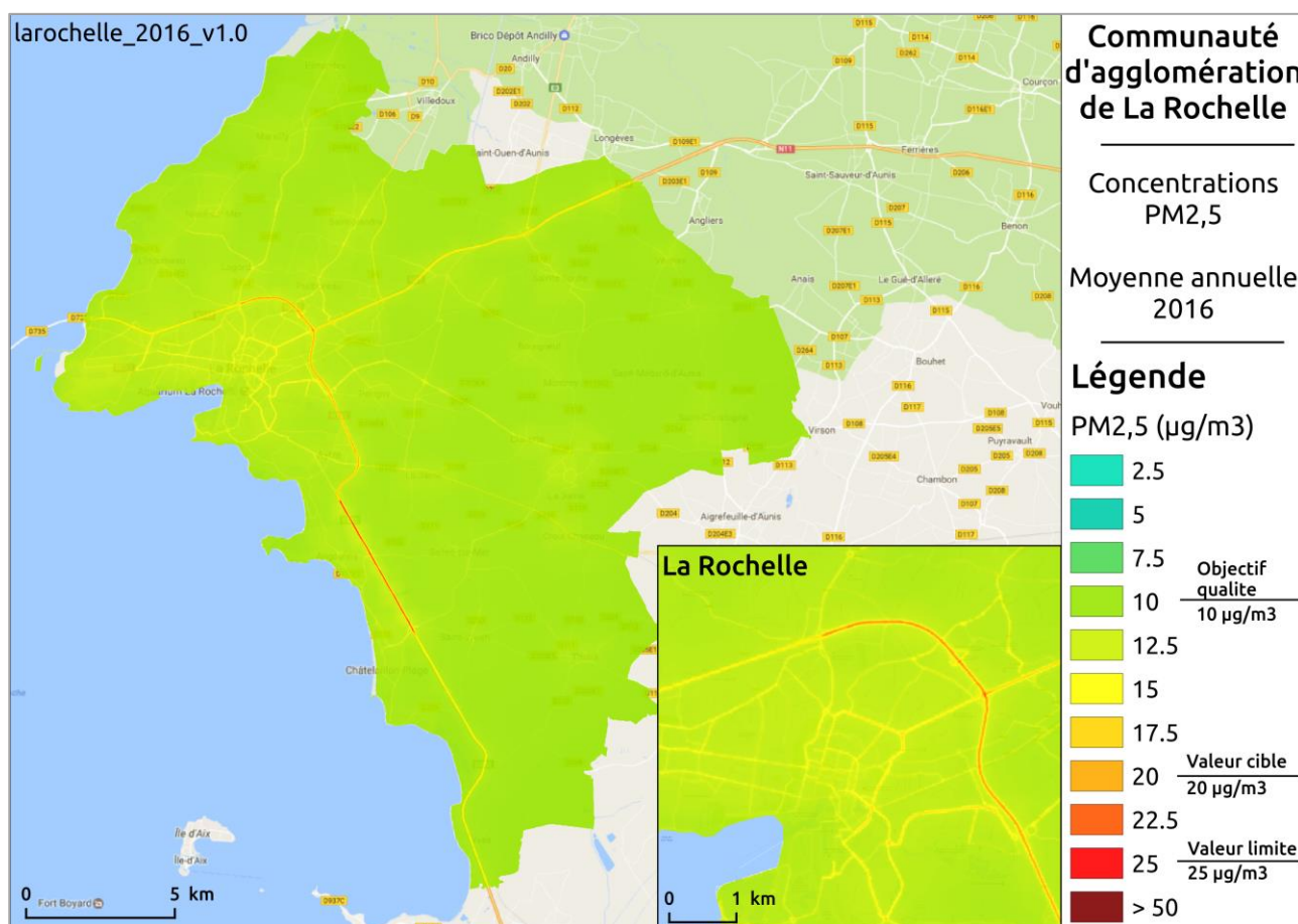
Figure 50: Modélisation des concentrations de PM2,5 sur l'agglomération de La Rochelle en 2016.
