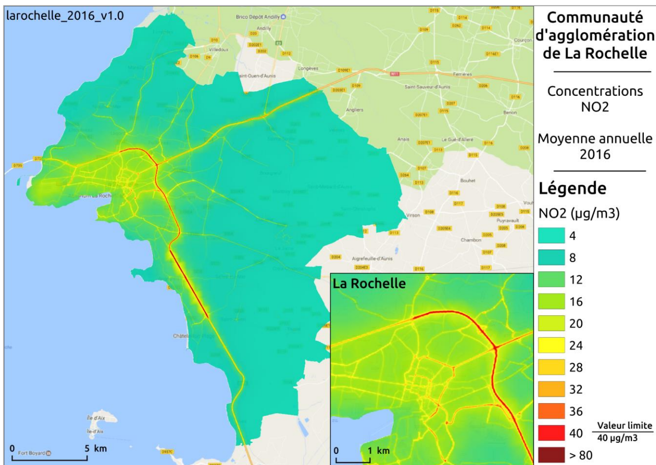
Figure 45 : Modélisation des concentrations de NO 2 sur l'agglomération de La Rochelle en 2016
