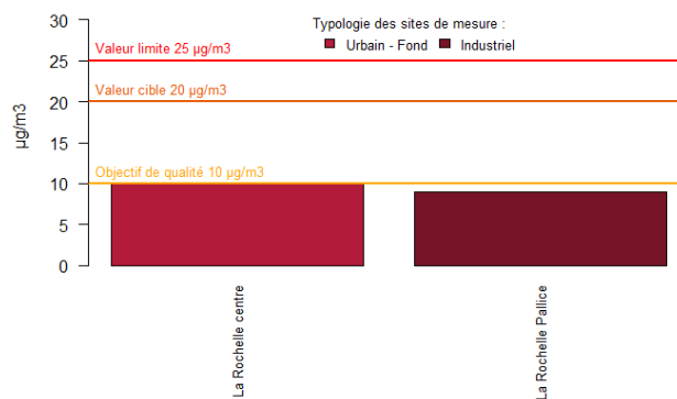
Figure 49 : Charente-Maritime - Moyennes annuelles en PM2,5
