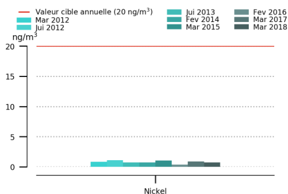
Figure 19 : Evolution des teneurs en nickel
