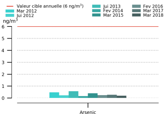
Figure 17 : Evolution des teneurs en arsenic
