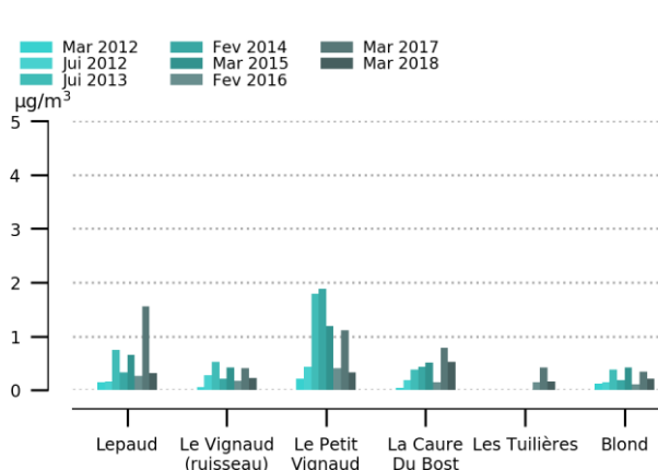
Figure 14 : Evolution des concentrations de toluène
