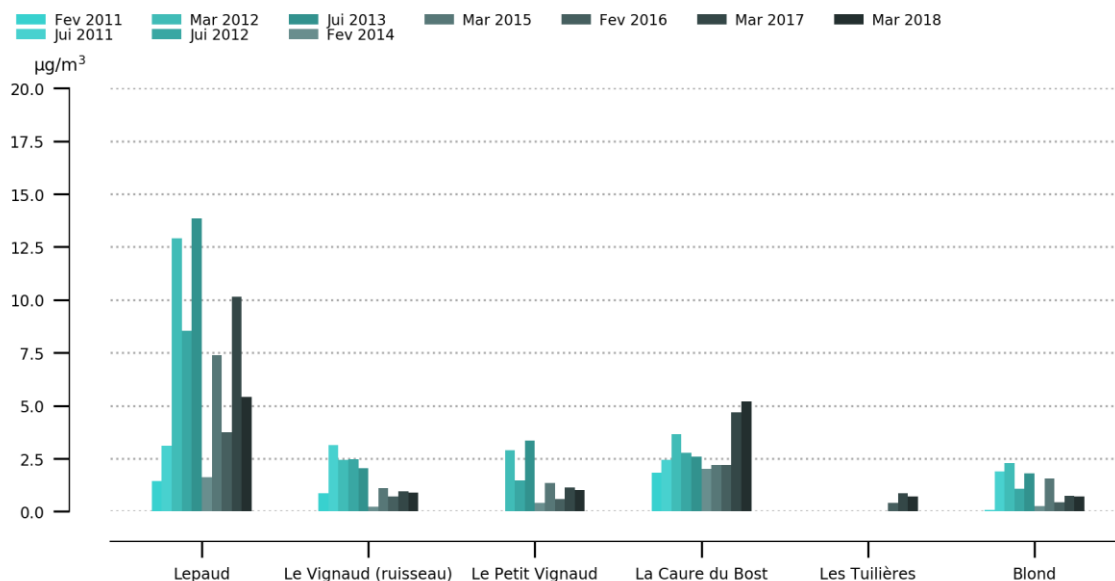
Figure 12 : Evolution des concentrations de NH 3
