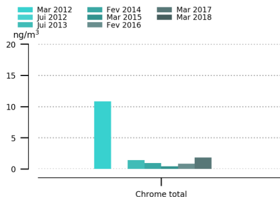
Figure 16 : Evolution des teneurs en chrome
