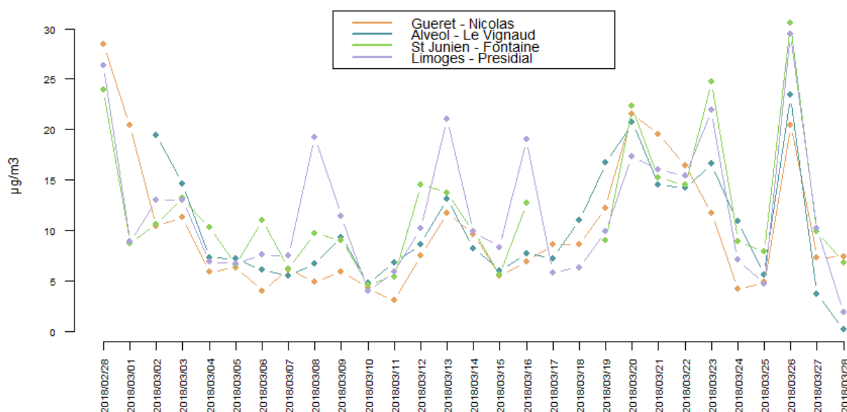
Figure 21 : Evolution des concentrations journalières de PM10
