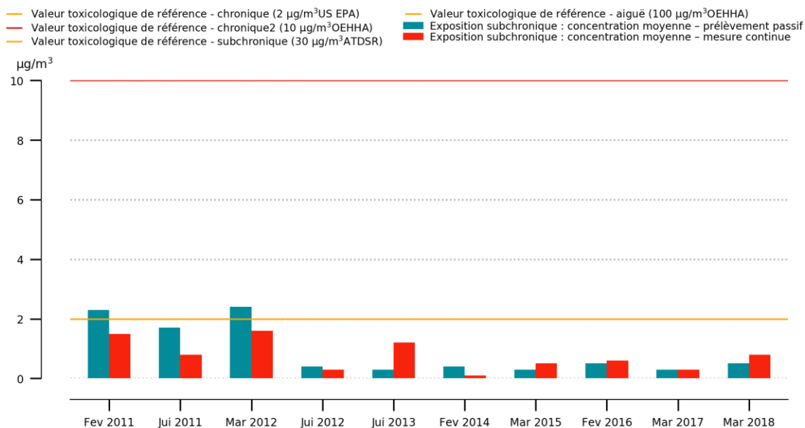
Figure 9 : Evolution des concentrations d'H 2 S en situation d'exposition subchronique
