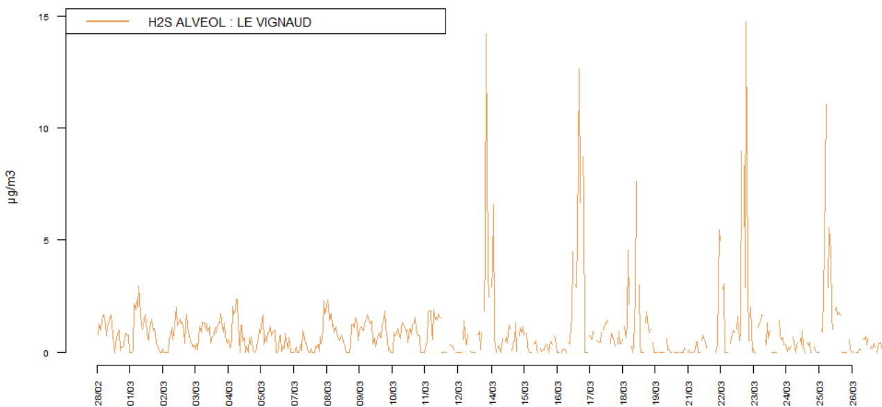
Figure 8 : Evolution des concentrations horaires d'H 2 S
