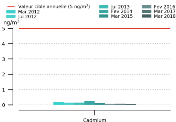
Figure 18 : Evolution des teneurs en cadmium
