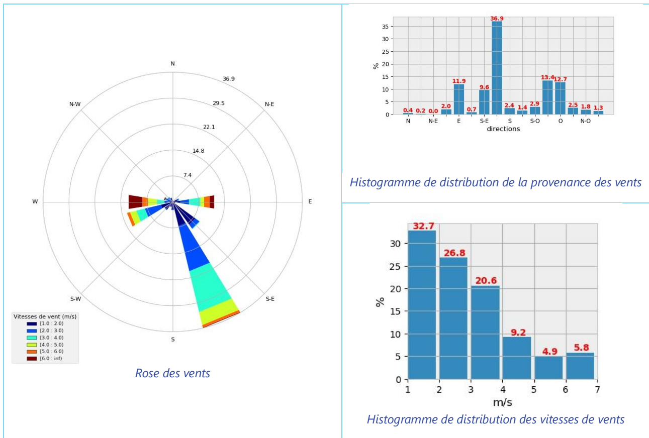
Figure 6 : Conditions météorologiques globales
