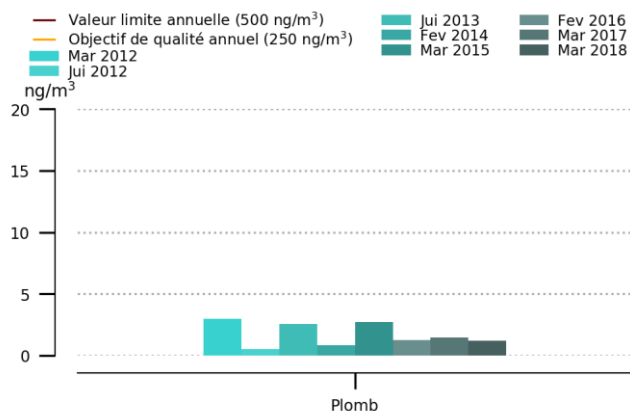
Figure 20 : Evolution des teneurs en plomb
