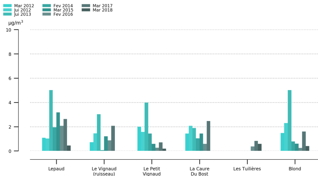
Figure 15 : Evolution des concentrations d'acide acétique
