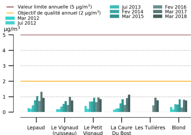
Figure 13 : Evolution des concentrations de benzène
