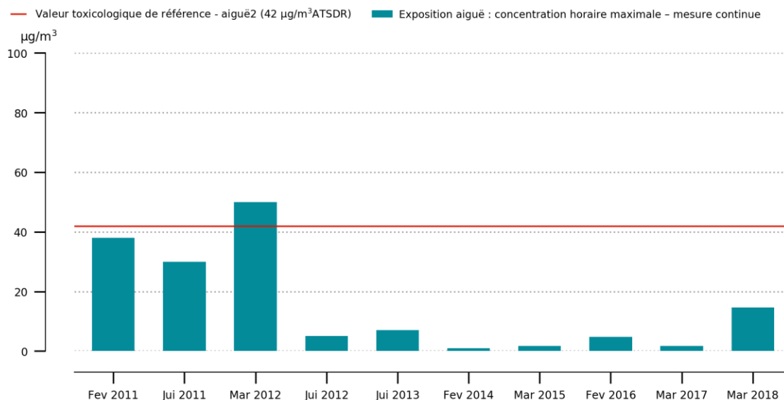
Figure 10 : Evolution des concentrations d'H 2 S en situation d'exposition aiguë
