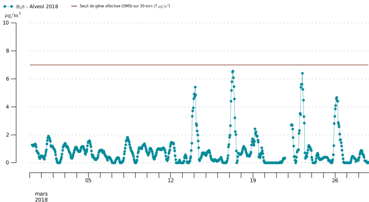
Figure 11 : Evolution de la moyenne glissante sur 30 min des concentrations quart-horaires d'H 2 S
