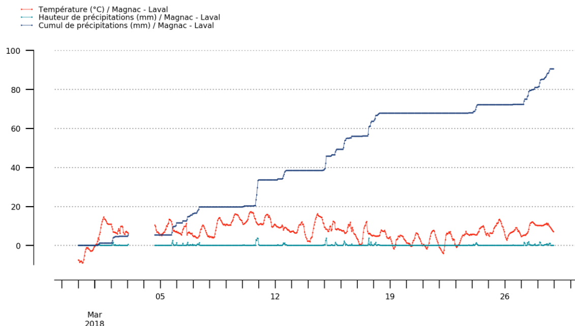
Figure 7 : Températures et hauteurs de précipitations horaires
