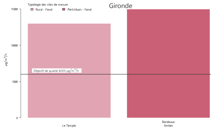
O 3 – AOT40 en 2019
