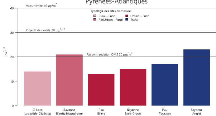
PM10 – moyenne annuelle 2019 Pyrénées-Atlantiques
