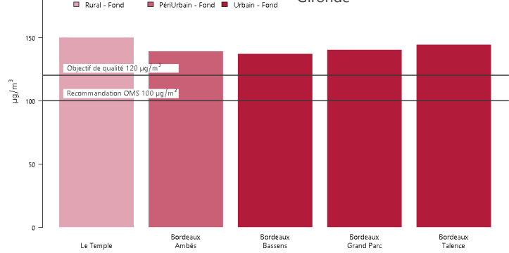
O 3 – maximum de la moyenne sur 8 heures en 2019
