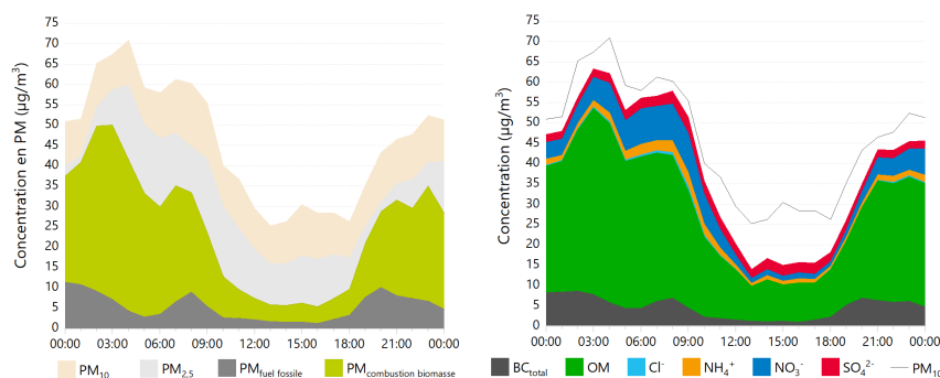
Composition chimique des particules le 26 février
