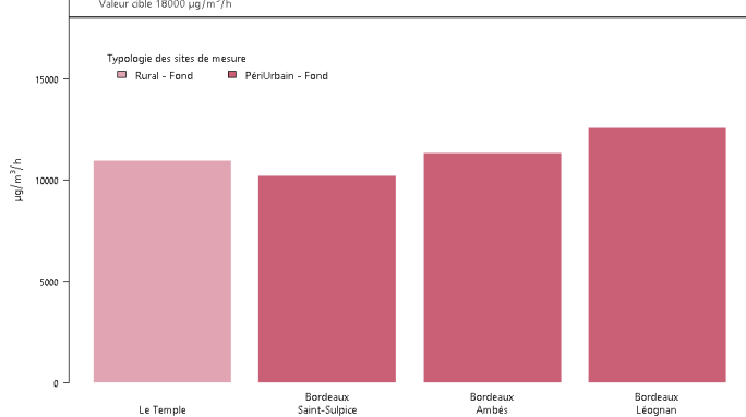
O 3 – AOT40 (moyenne sur 5 ans) en 2019
