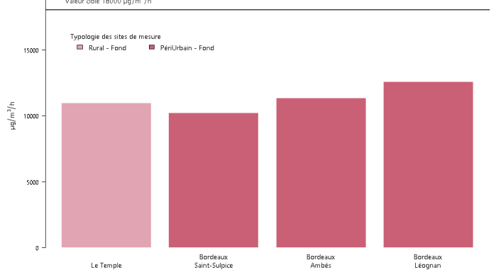
O 3 – AOT40 (moyenne sur 5 ans) en 2019
