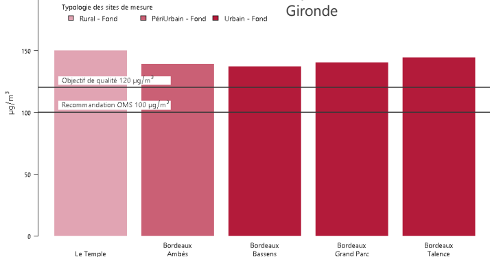
O 3 – maximum de la moyenne sur 8 heures en 2019
