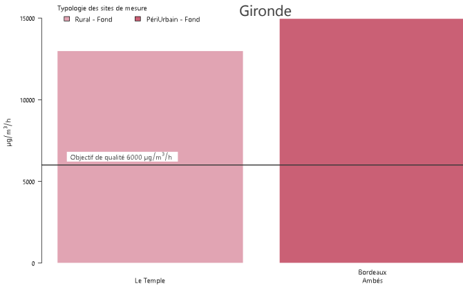
O 3 – AOT40 en 2019
