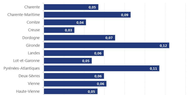
Emissions B(a)P par département - tonne - 2016
