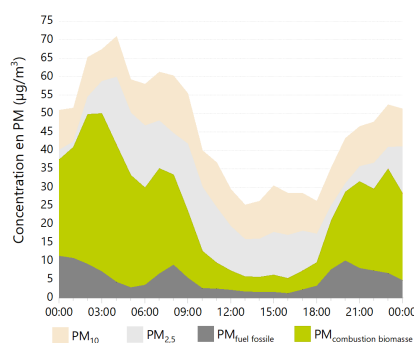
Composition chimique des particules le 26 février
