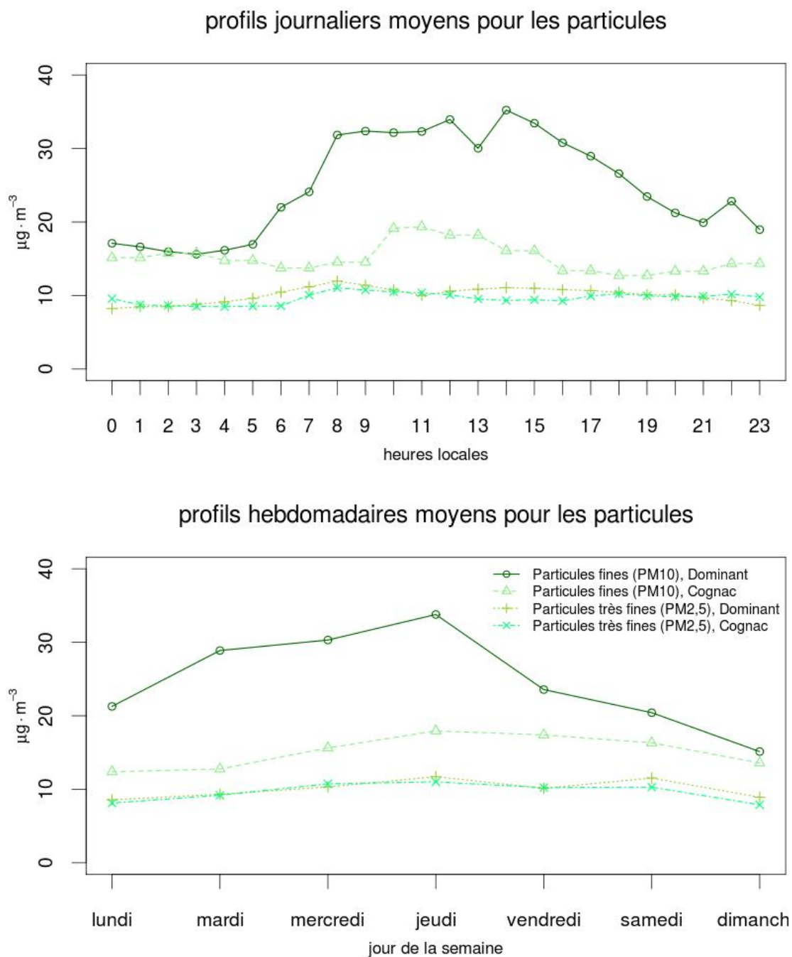
FIGURE 5.1 – Tendances temporelles moyennes en particules sur le site du Dominant
