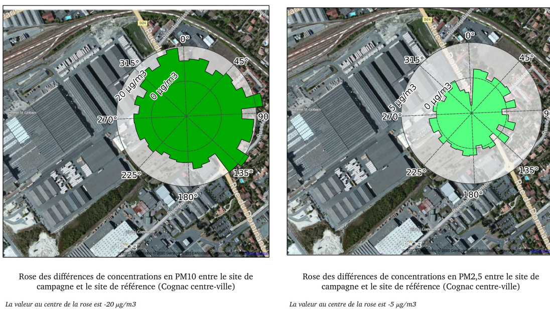
FIGURE 5.2 – Rose des différences moyennes en particules fines
