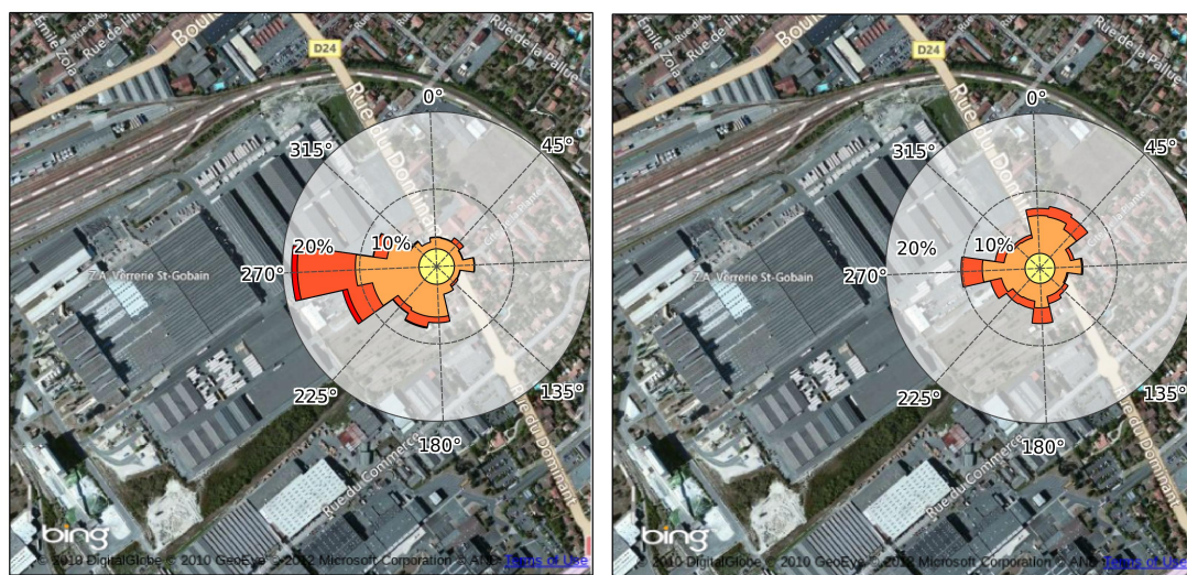
Rose des vents au cours de la campagne
