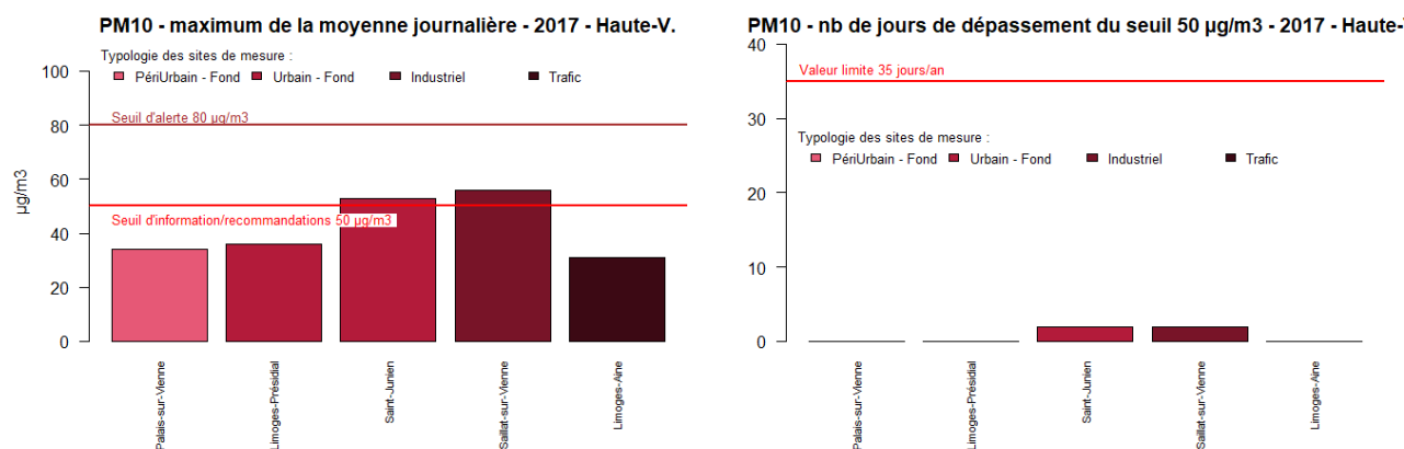
Figure 140 : Haute-V. - Maxima des valeurs journalières et nombre de jours de dépassement du seuil de 50 µg/m 3 en PM10
