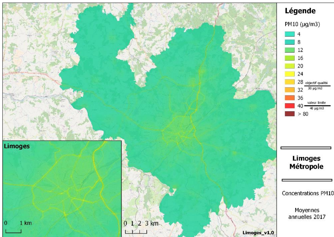
Figure 141 : Modélisation des concentrations de PM10 sur Limoges Métropole en 2017.
