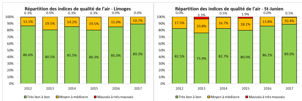
Figure 136 : Haute-Vienne - Répartition des indices de qualité de l'air depuis 2012
