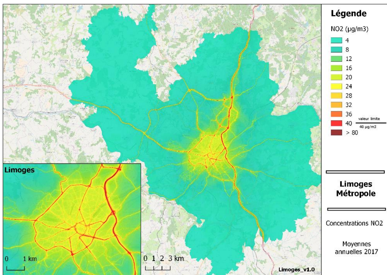
Figure 138 : Modélisation des concentrations de NO 2 sur Limoges Métropole en 2017.
