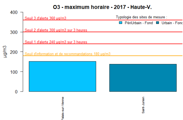
Figure 143 : Haute-Vienne - Maxima horaires en O 3
