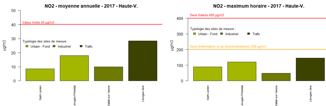
Figure 137 : Haute-Vienne - Moyennes annuelles et maxima des valeurs horaires en NO 2
