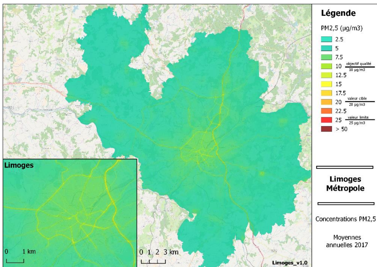
Figure 142 : Modélisation des concentrations de PM2,5 sur Limoges Métropole en 2017.
