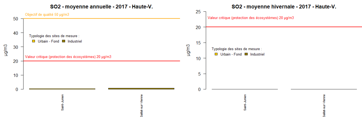
Figure 145 : Haute-Vienne – Moyennes annuelles et hivernales en \text{SO}_2
