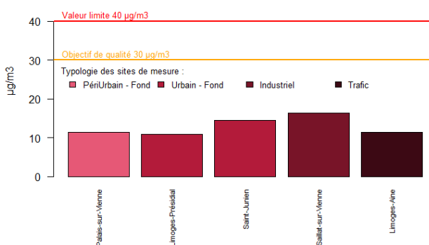
Figure 139 : Haute-Vienne - Moyennes annuelles en PM10
