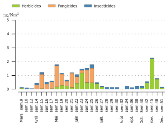
Figure 148 : Cumul des concentrations hebdomadaires par usage sur Limoges
