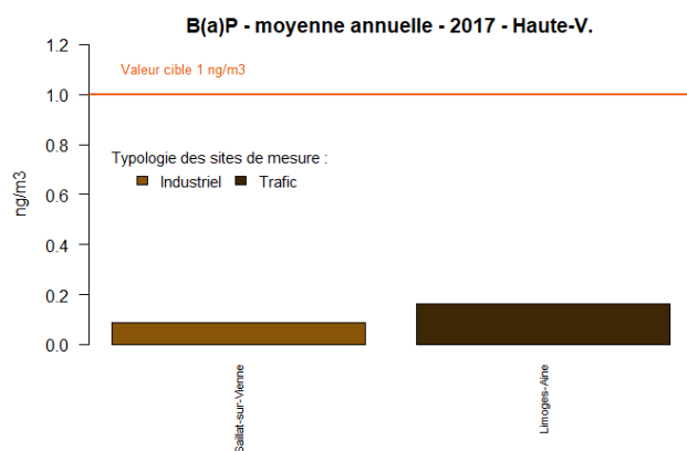
Figure 147 : Haute-Vienne - Moyennes annuelles en B(a)P
