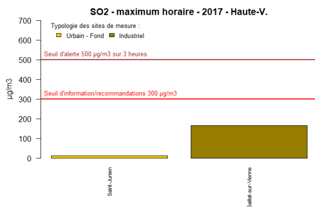
Figure 146 : Haute-Vienne Maxima des valeurs horaires en SO 2
