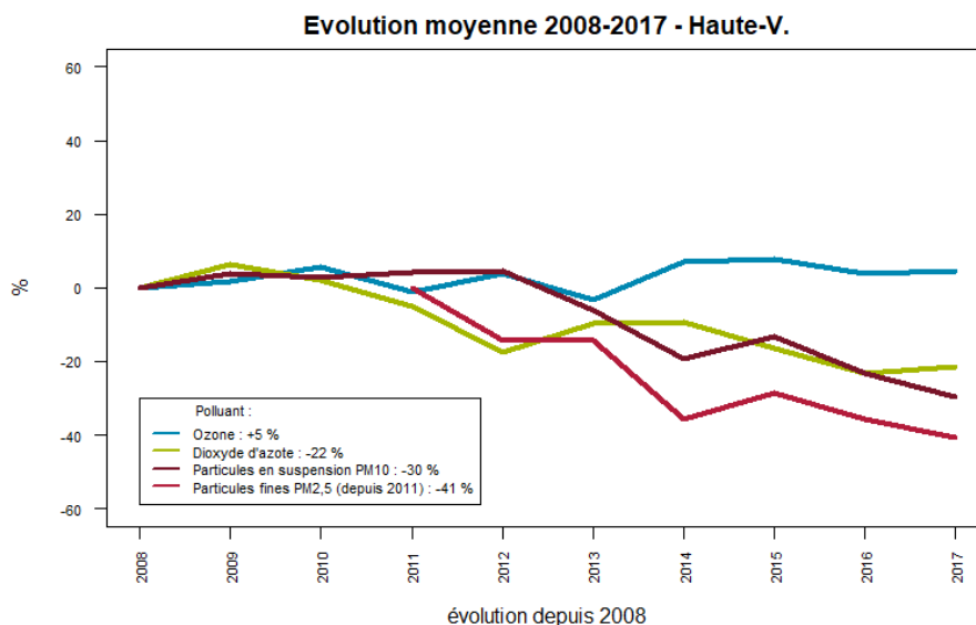
Figure 149 : Haute-Vienne - Evolution pluriannuelle des concentrations moyennes en polluants réglementés
