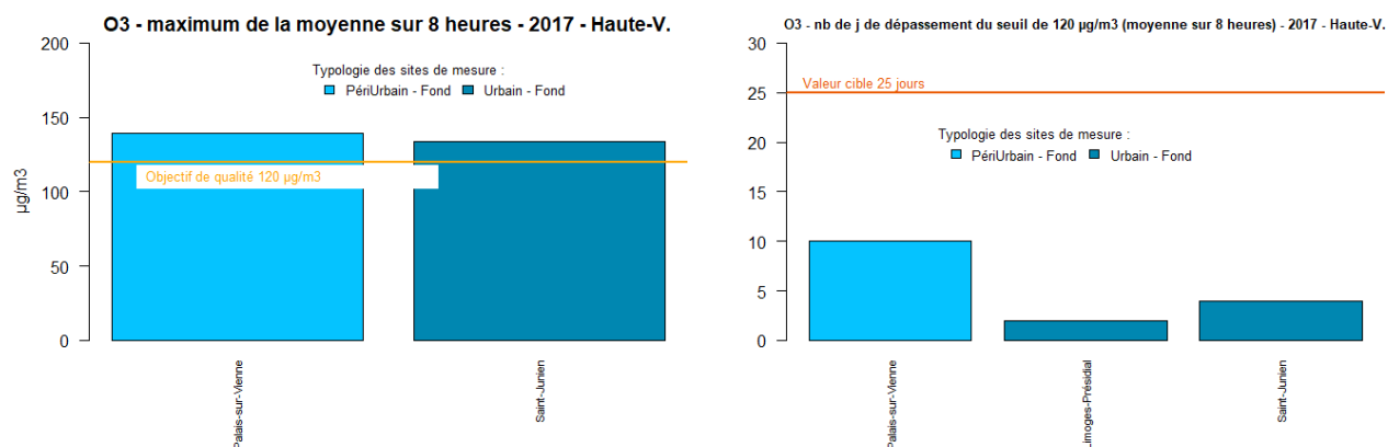
Figure 144 : Haute-V. - Max des moy. sur 8 h et nb moy. sur 3 ans de j de dépassement du seuil de 120 µg/m 3 sur 8 h en O 3
