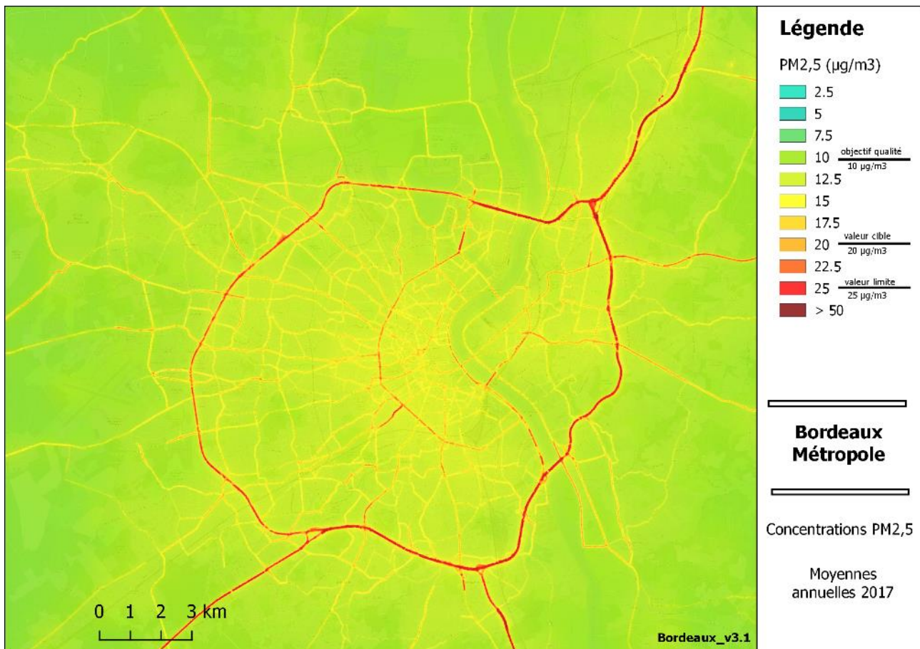
Figure 78 : Modélisation des concentrations de PM2,5 sur Bordeaux Métropole en 2017.
