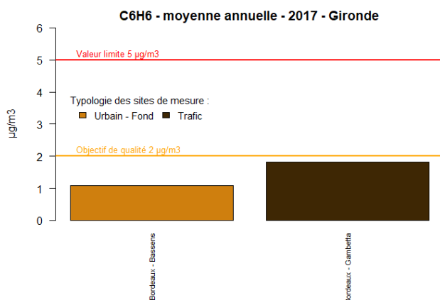
Figure 82 : Gironde - Moyennes annuelles en C 6 H 6
