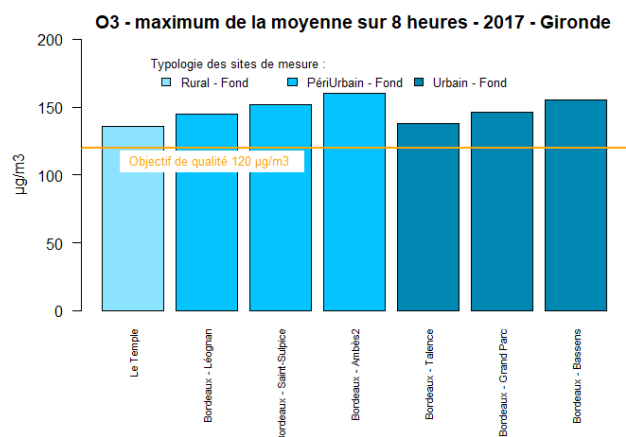
Figure 80 : Gironde - Max des moy. sur 8 h et nb moy sur 3 ans de j de dépassement du seuil de 120 µg/m 3 sur 8 h en O 3
