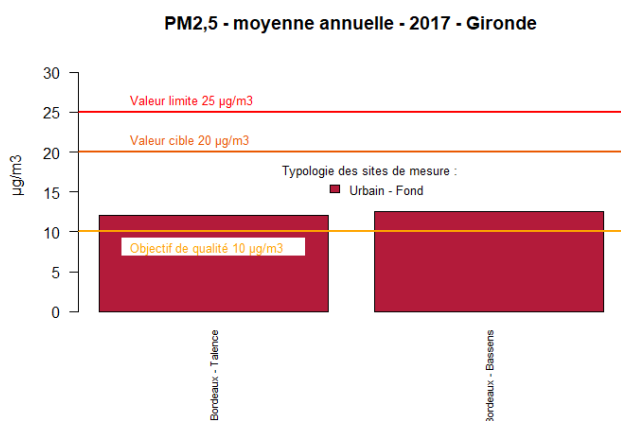
Figure 77 : Gironde - Moyennes annuelles en PM2,5
