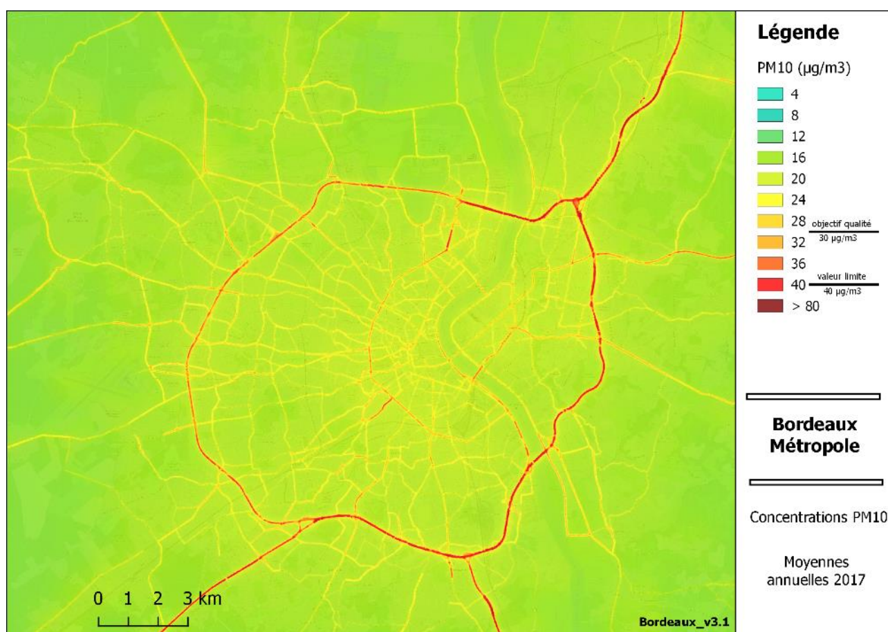
Figure 76 : Modélisation des concentrations de PM10 sur Bordeaux Métropole en 2017.
