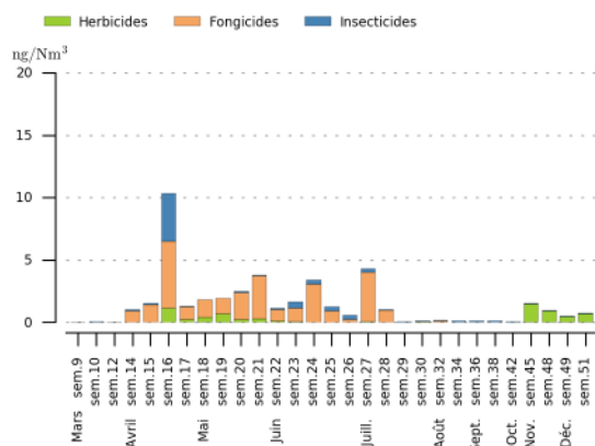
Figure 83 : Cumul des concentrations hebdomadaires par usage sur le site de Bordeaux
