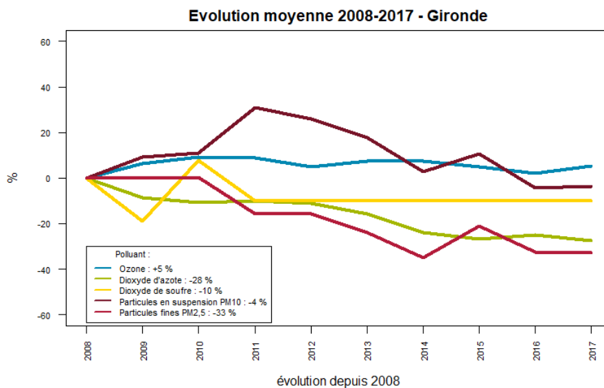
Figure 85 : Gironde - Evolution pluriannuelle des concentrations moyennes en polluants réglementés
