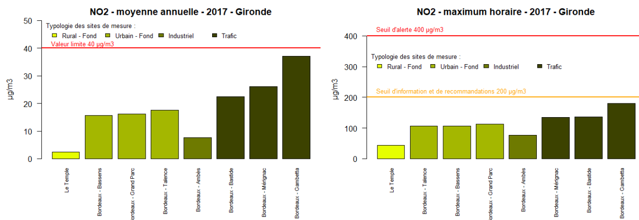
Figure 72 : Gironde - Moyennes annuelles et maxima horaires en NO 2
