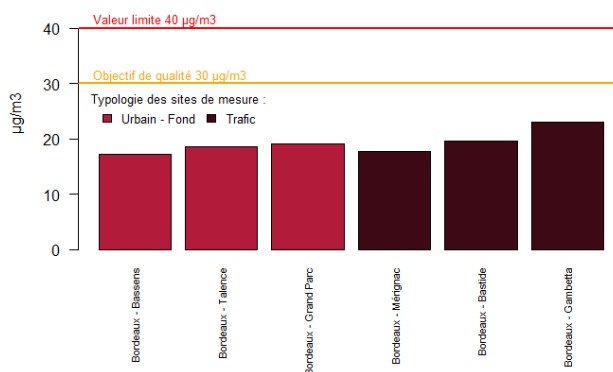
Figure 74 : Gironde - Moyennes annuelles en PM10
