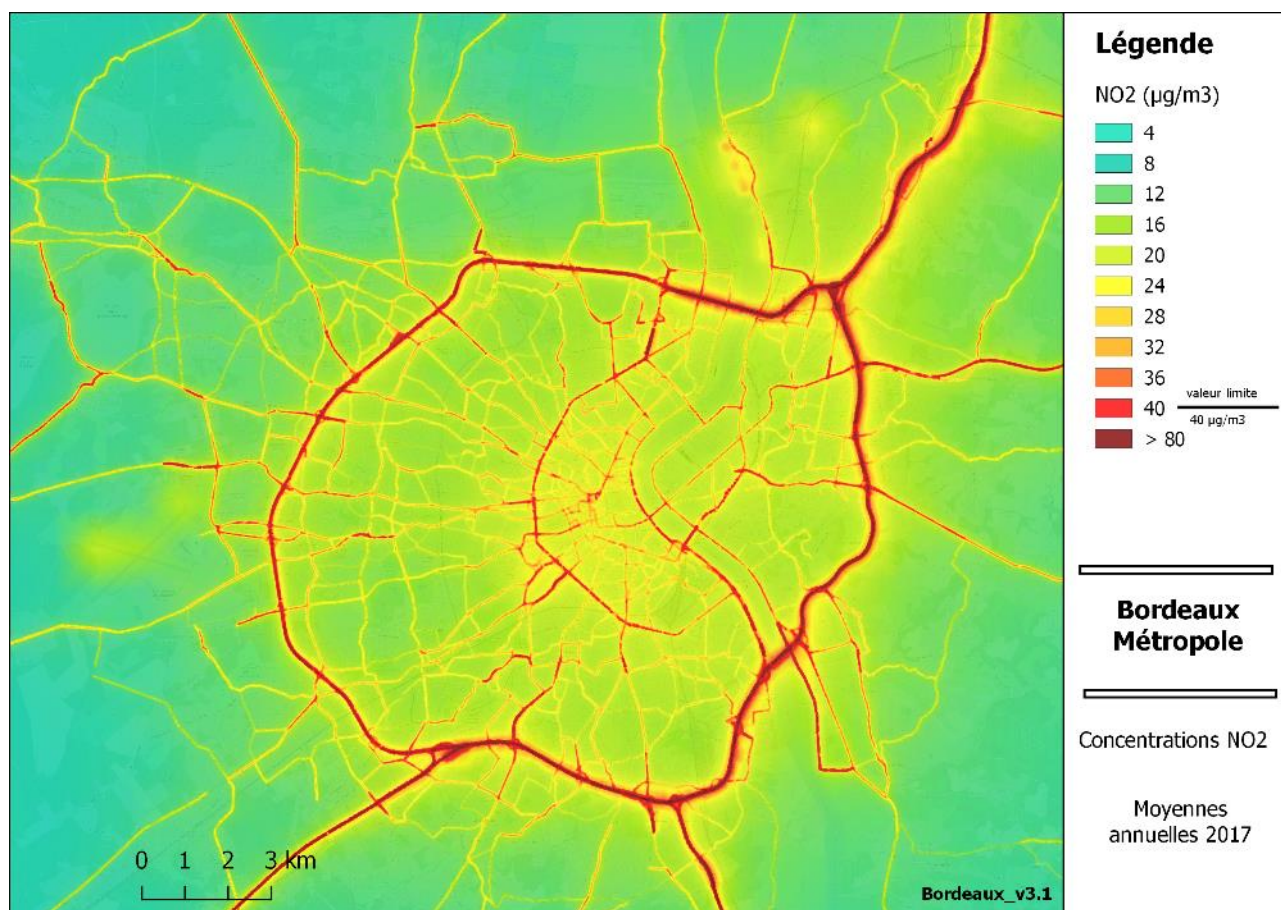
Figure 73 : Modélisation des concentrations de NO 2 sur Bordeaux Métropole en 2017.
