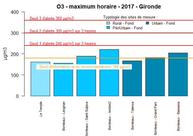
Figure 79 : Gironde - Maxima horaires en O 3
