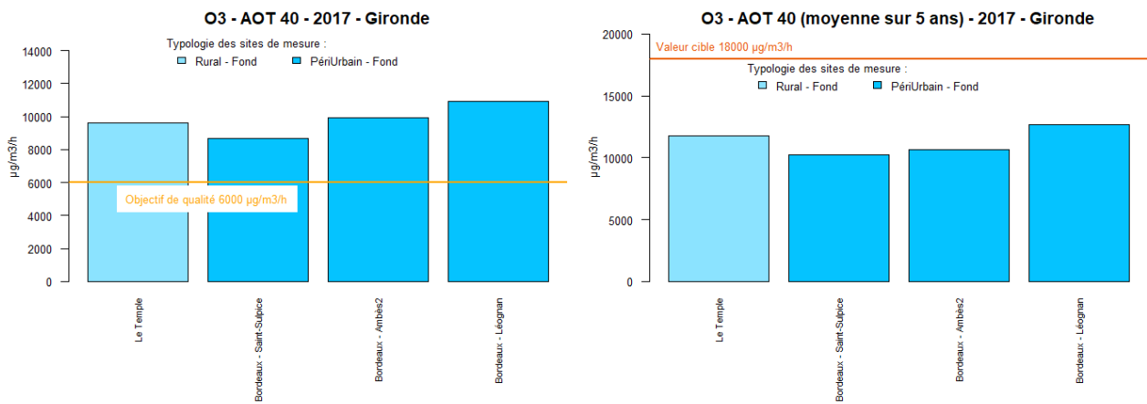
Figure 81 : Gironde – AOT40 et moyenne des AOT40 sur 5 ans en O 3
