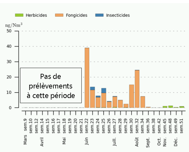
Figure 84 : Cumul des concentrations hebdomadaires par usage sur le site du Médoc
