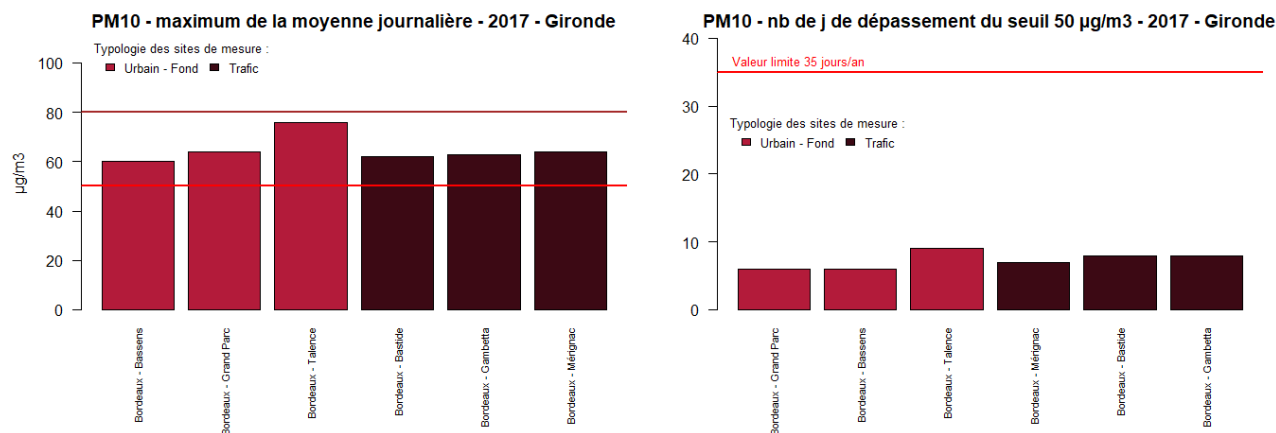
Figure 75 : Gironde - Maxima des valeurs journalières et nombre de jours de dépassement du seuil de 50 \mu\text{g}/\text{m}^3 en PM10
