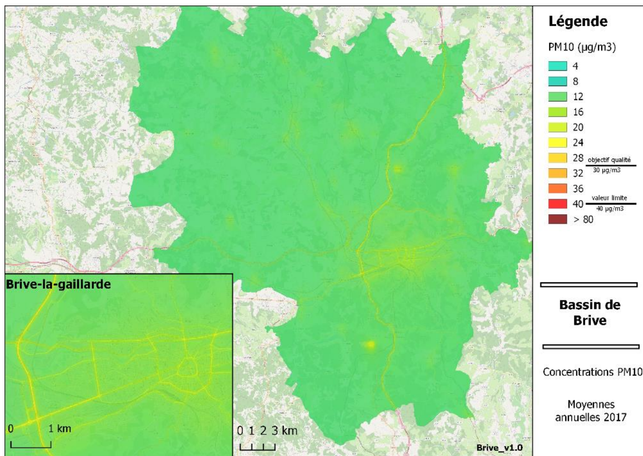
Figure 60 : Modélisation des concentrations de PM10 sur le Bassin de Brive en 2017.
