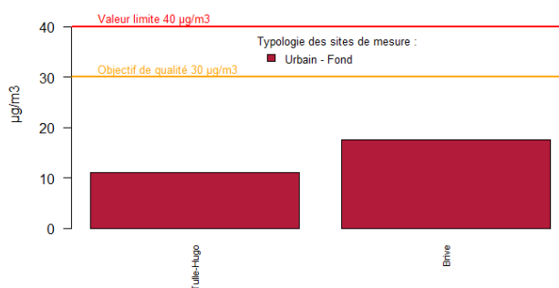
PM10 - moyenne annuelle - 2017 - Corrèze
