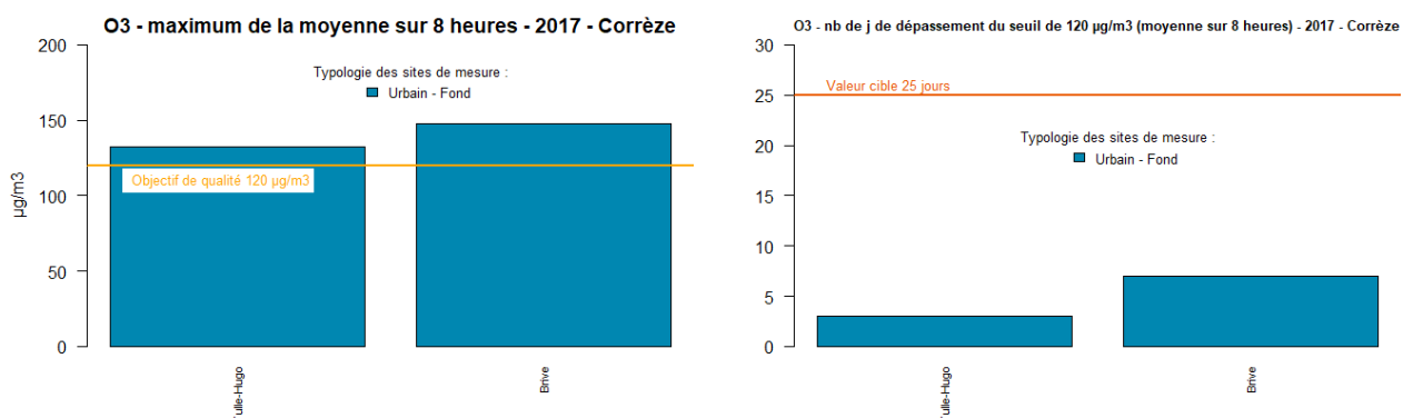
Figure 62 : Corrèze - Maxima horaires en O 3
