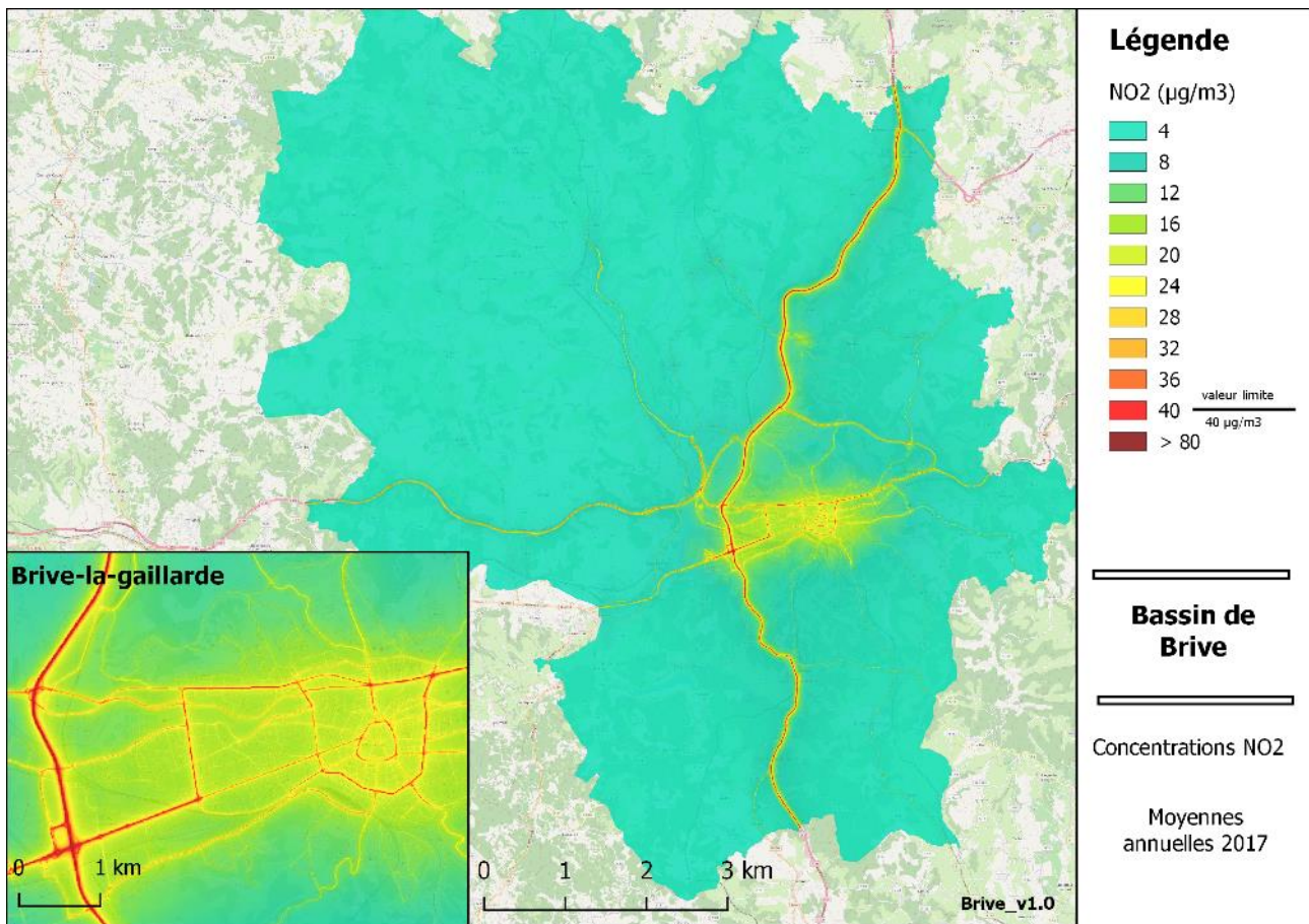
Figure 57 : Modélisation des concentrations de NO 2 sur le bassin de Brive en 2017.
