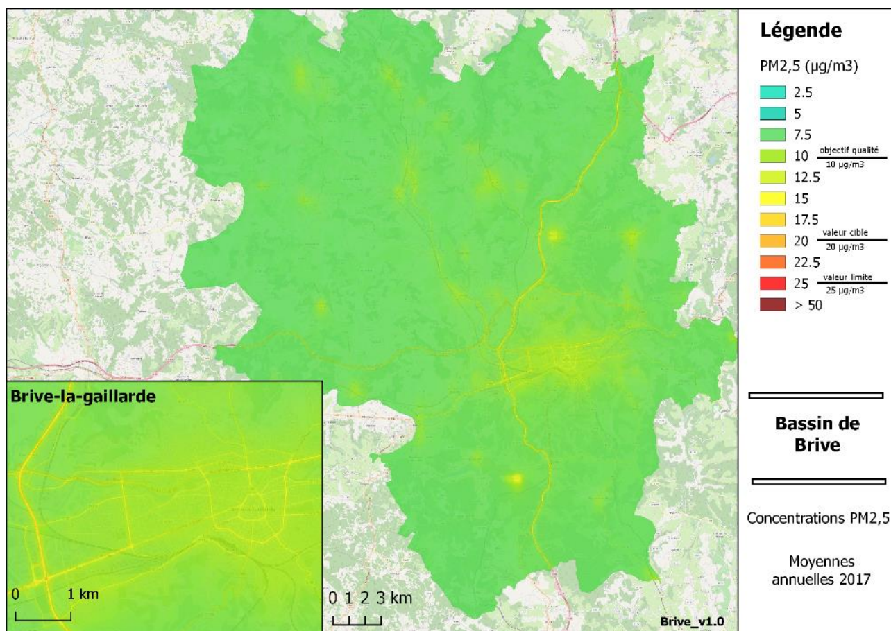
Figure 61 : Modélisation des concentrations de PM2,5 sur le bassin de Brive en 2017.
