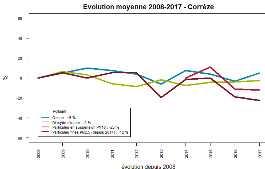
Figure 64 : Corrèze - Evolution pluriannuelle des concentrations moyennes en polluants réglementés
