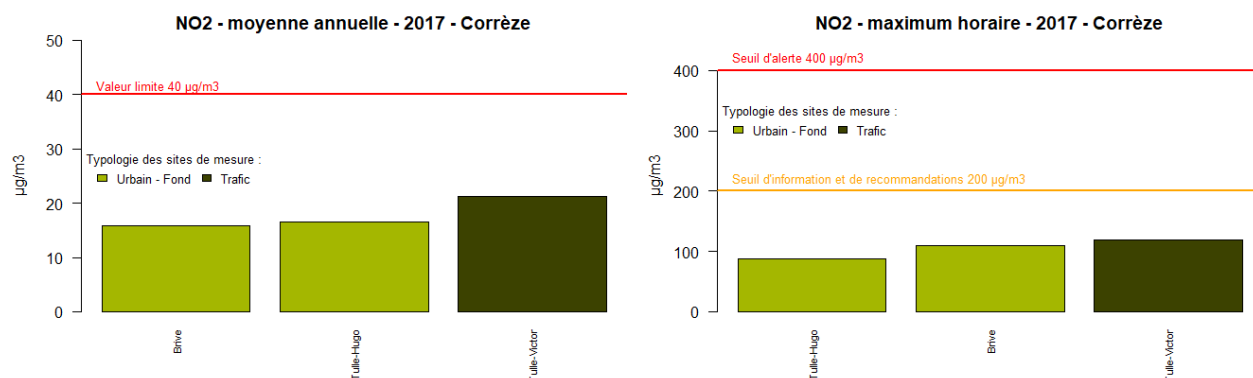
Figure 56 : Corrèze - Moyennes annuelles et maxima horaires en NO 2
