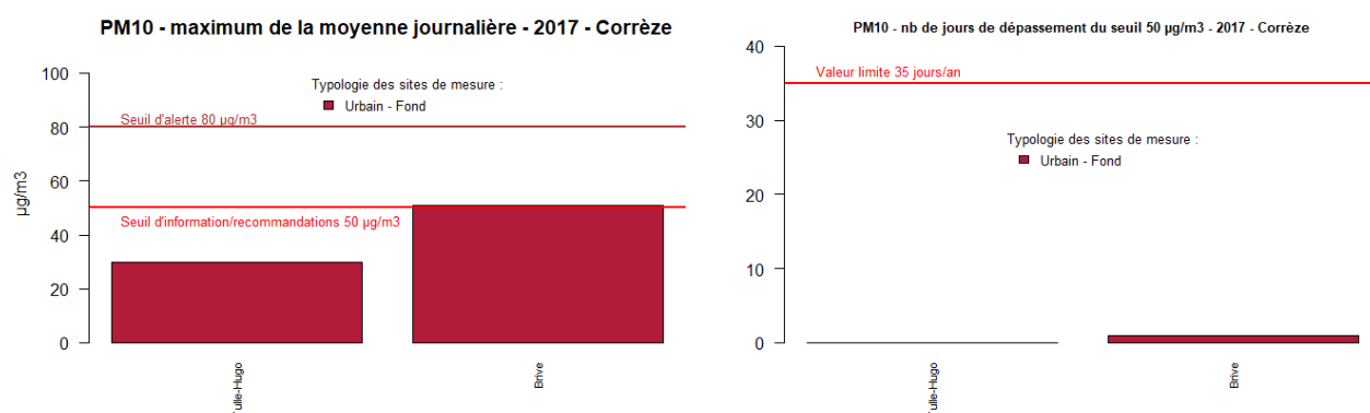
Figure 59 : Corrèze - Maxima des valeurs journalières et nombre de jours de dépassement du seuil de 50 \mu\text{g}/\text{m}^3 en PM10
