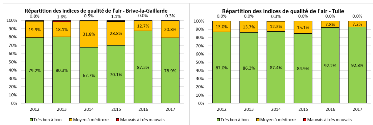
Figure 55 : Corrèze- Répartition des indices de qualité de l'air depuis 2012
