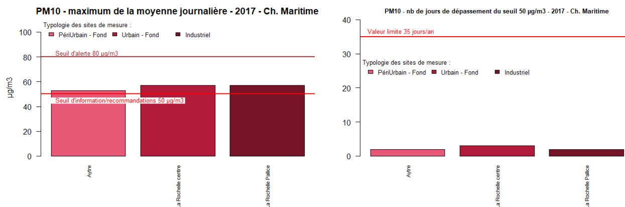
Figure 48 : Char.-Mar. - Maxima des valeurs journalières et nombre de jours de dépassement du seuil de 50 µg/m 3 en PM10
