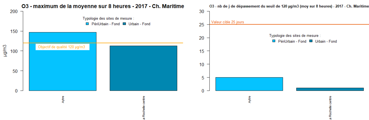
Figure 53 : Ch.-Mar. - Max des moy. sur 8 h et nb moy sur 3 ans de j de dépassement du seuil de 120 µg/m 3 sur 8 h en O 3
