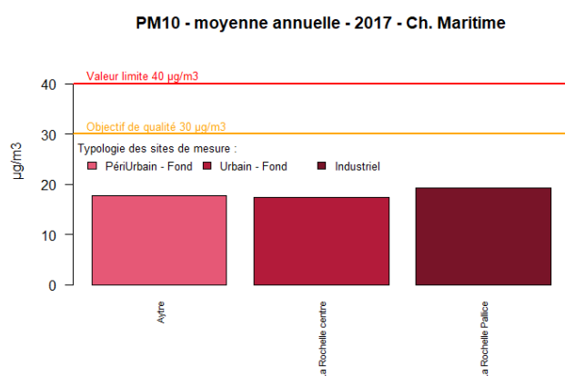
Figure 47 : Charente-Maritime - Moyennes annuelles en PM10
