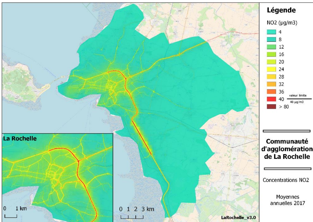
Figure 46 : Modélisation des concentrations de NO 2 sur l'agglomération de La Rochelle en 2017
