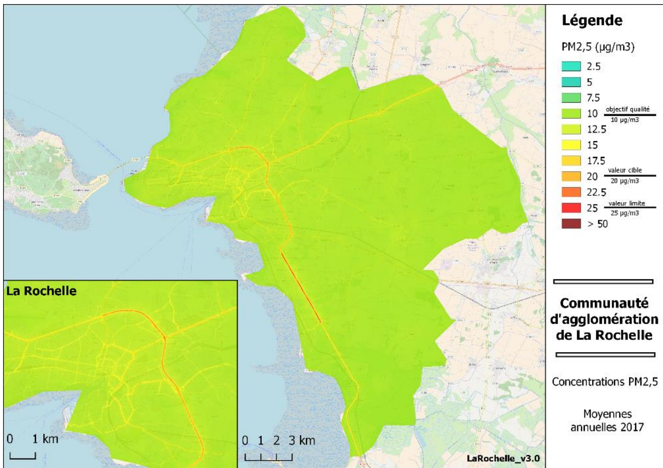
Figure 51 : Modélisation des concentrations de PM2,5 sur l'agglomération de La Rochelle en 2017.
