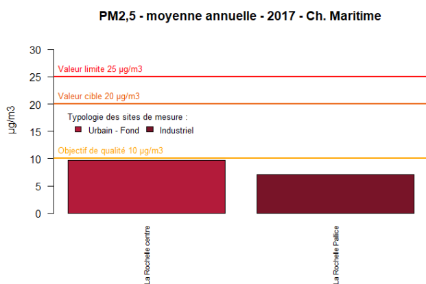
Figure 50 : Charente-Maritime - Moyennes annuelles en PM2,5
