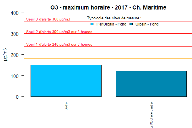
Figure 52 : Charente-Maritime - Maxima horaires en O 3
