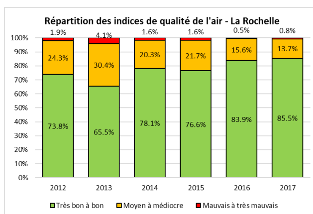
Figure 44 : Charente-Maritime - Répartition des indices de qualité de l'air depuis 2012
