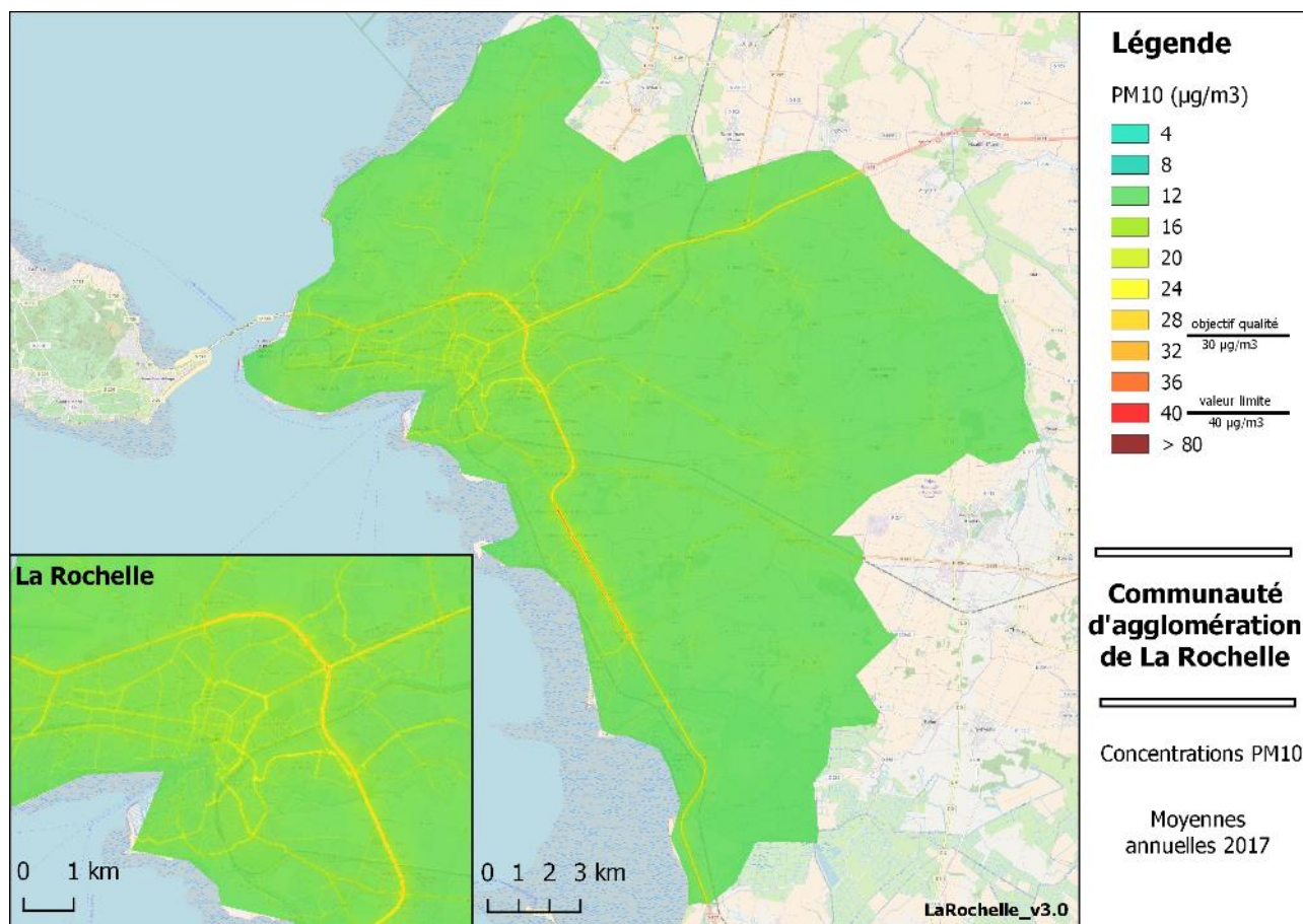
Figure 49: Modélisation des concentrations de PM10 sur l'agglomération de La Rochelle en 2017.
