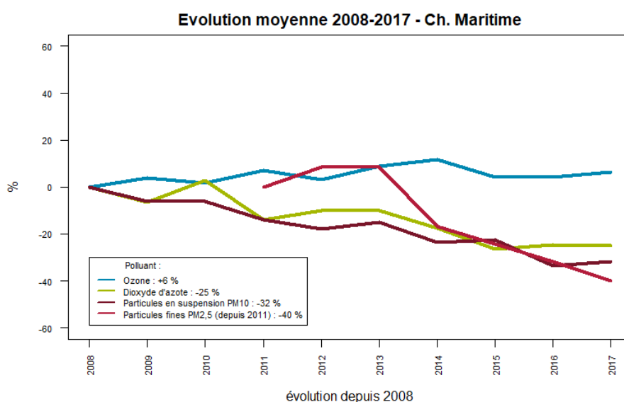
Figure 54 : Charente-Maritime- Evolution pluriannuelle des concentrations moyennes en polluants réglementés
