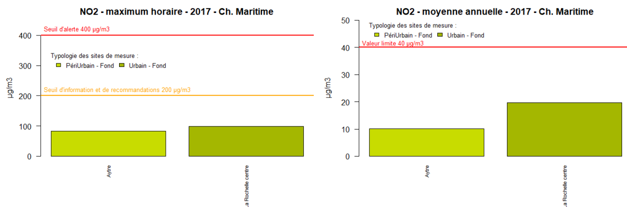
Figure 45 : Charente-Maritime - Moyennes annuelles et maxima horaires en NO 2
